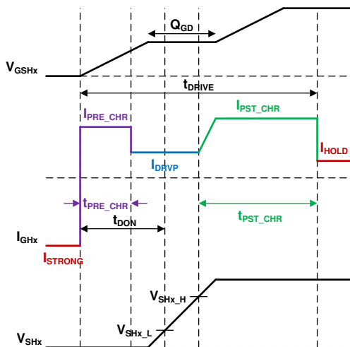
图 7-22. PDR 充电曲线
