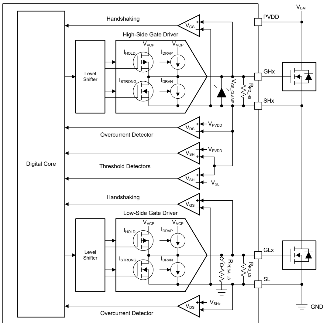
图 7-20. 栅极驱动器功能方框图
