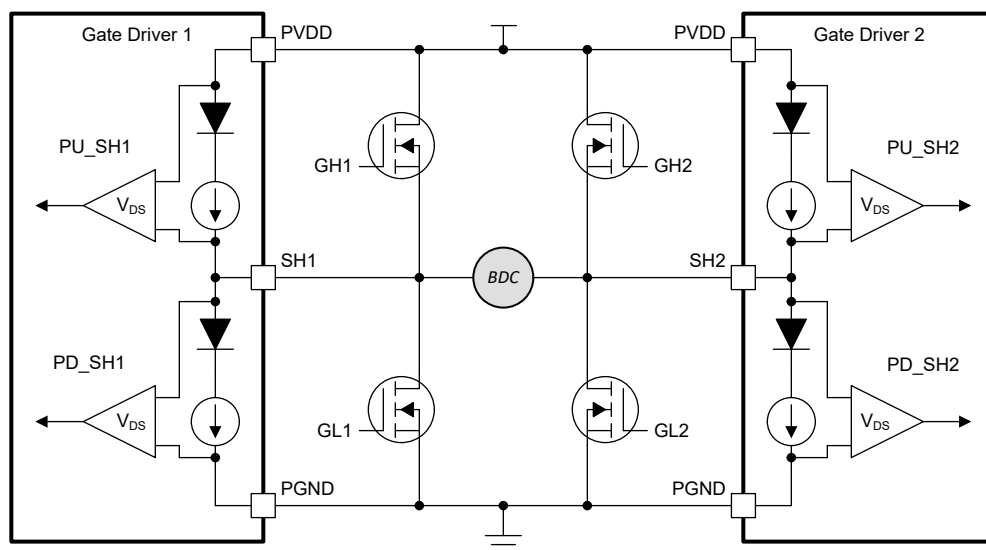
图 7-29. 离线诊断
