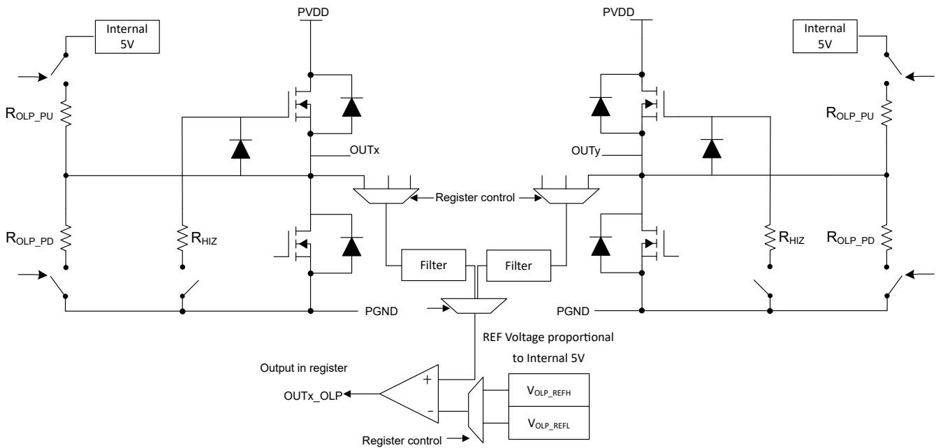
图 7-12. 关闭状态 ( 无源 ) 诊断
