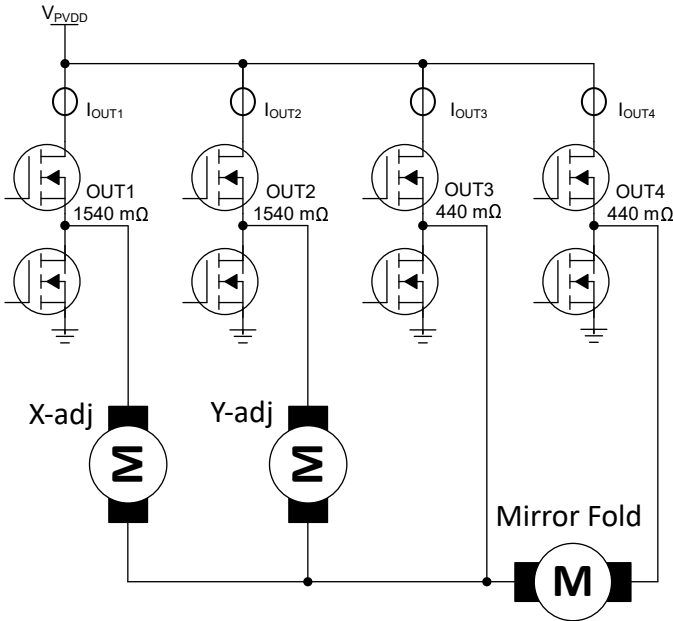
图 7-10. 适用于多达三个电机的半桥配置 (后视镜)
