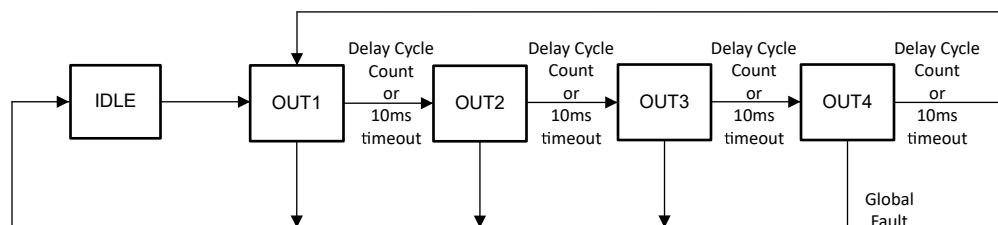
图 7-13. 半桥开路负载有源检测
