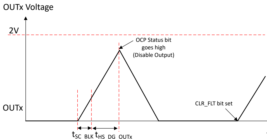
图 7-5. 高侧驱动器短路保护
