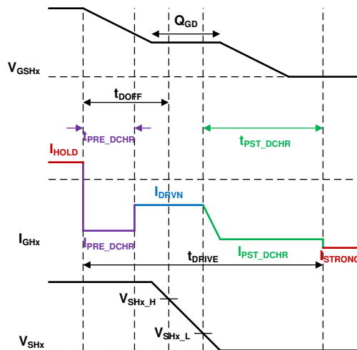
图 7-23. PDR 放电曲线
