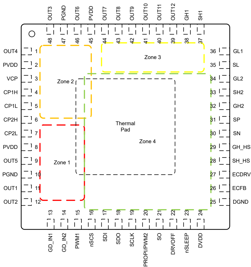
图 7-31. 热传感器区域
