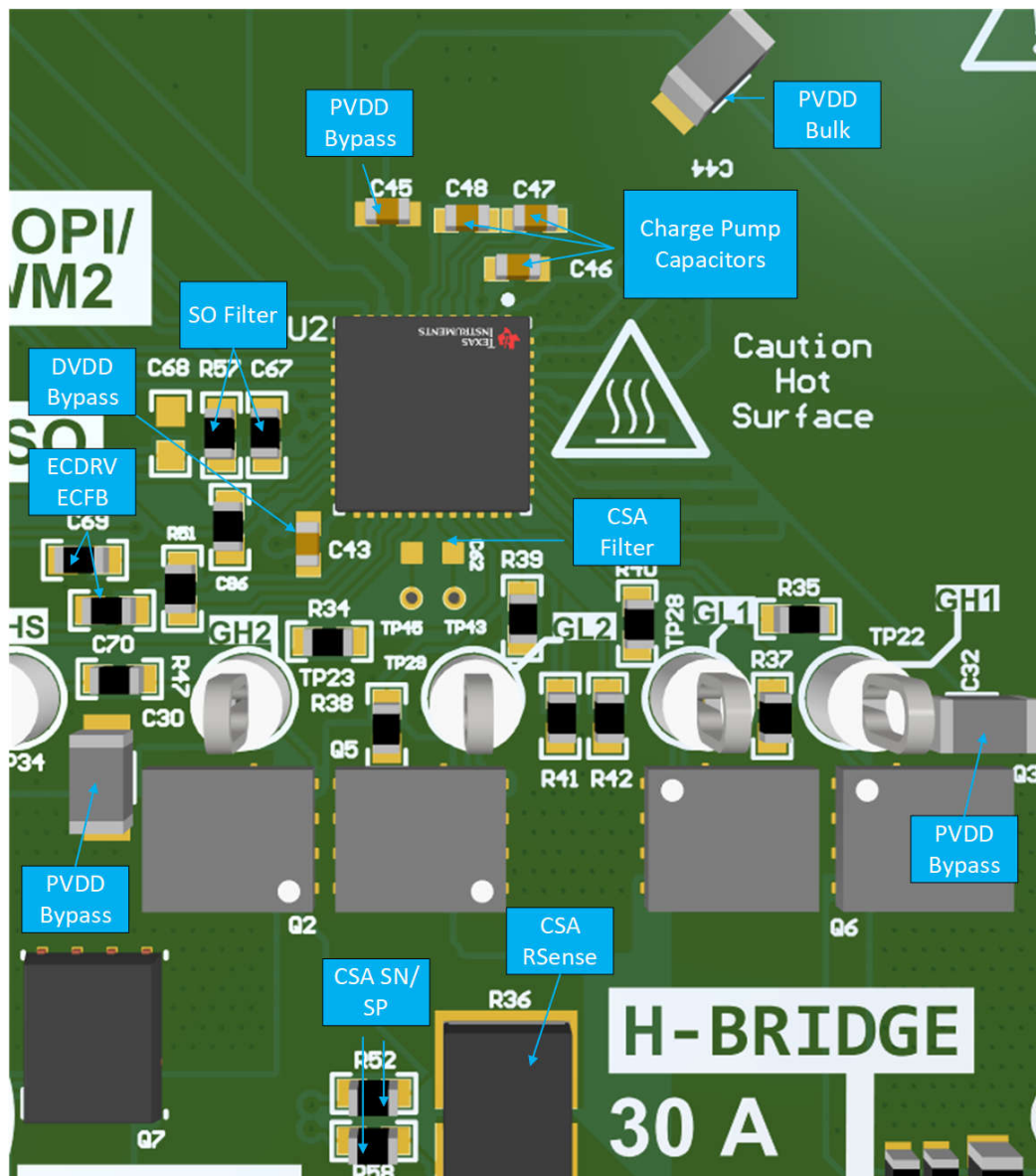
图 9-2. DRV8003-Q1 元件放置和布局
