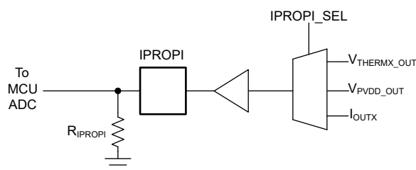
图 7-30. IPROPI 输出电路
