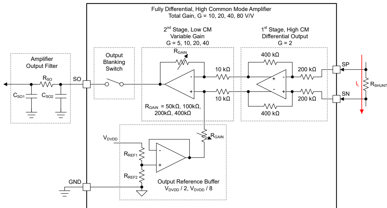
图 7-27. 放大器详细方框图
