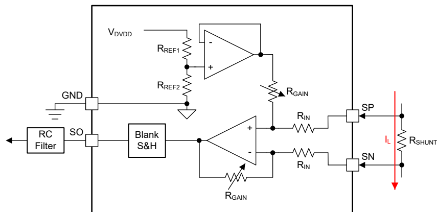
图 7-26. 放大器简化版方框图
