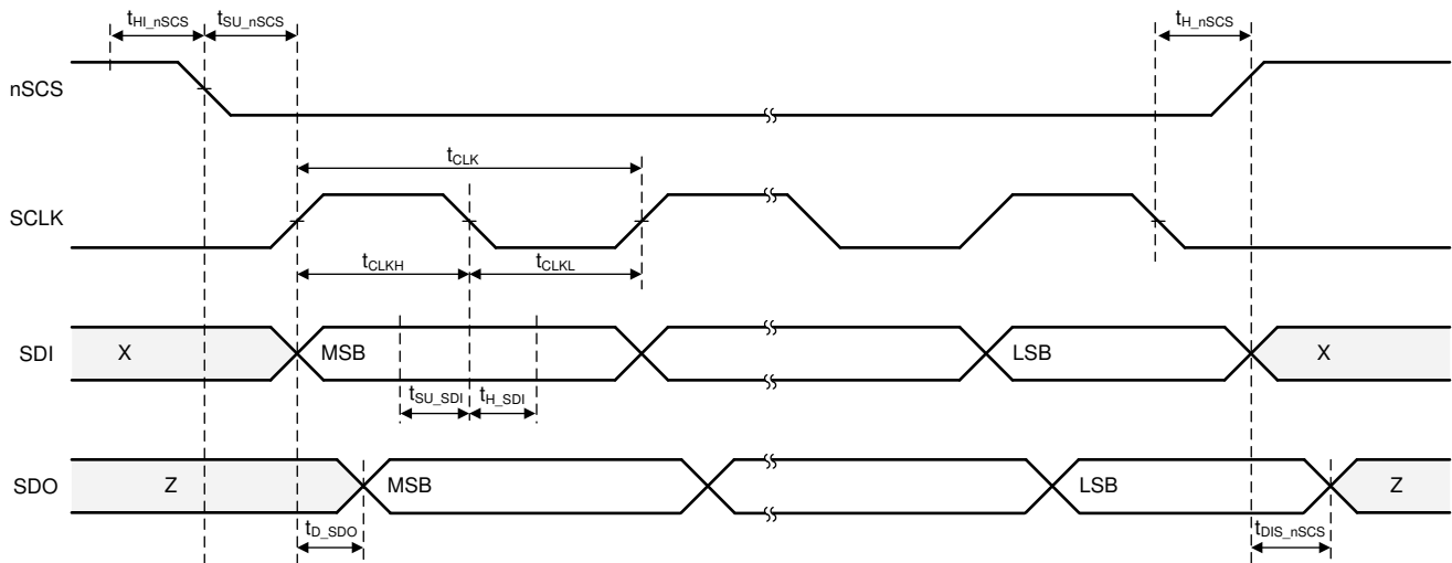
图 7-34. SPI 时序图
