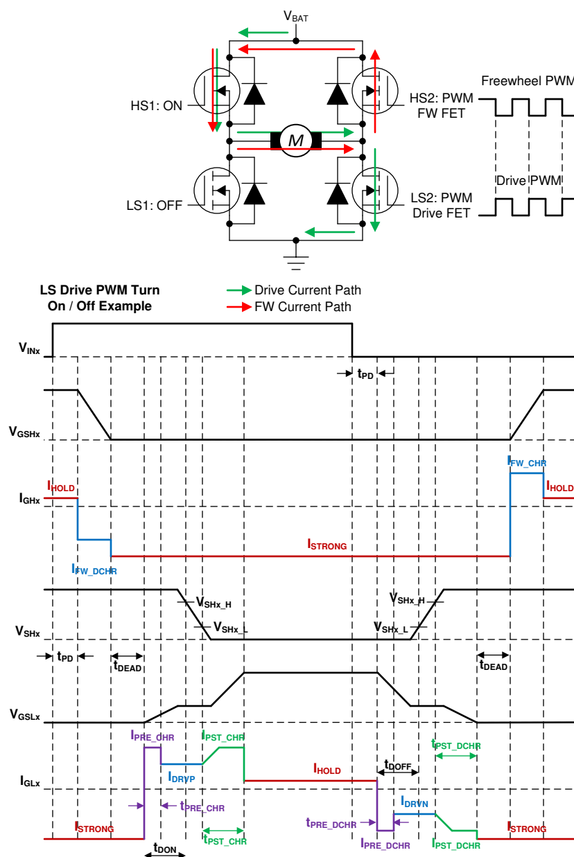
图 7-25. LS 驱动 PWM 导通/关断示例
