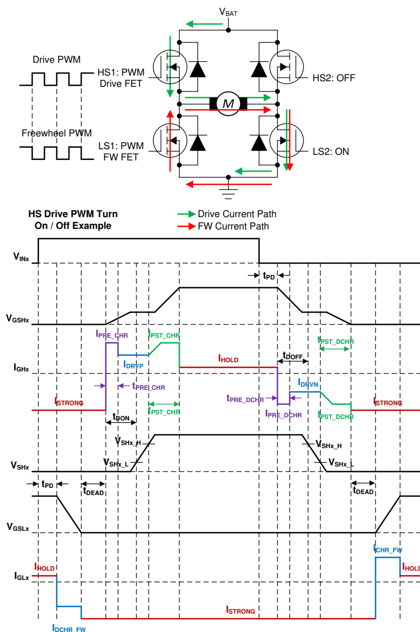
图 7-24. HS 驱动 PWM 导通/关断示例
