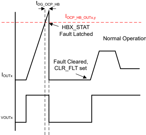
图 7-14. 半桥的过流行为
