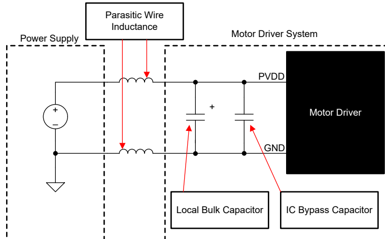
图 9-1. 电机驱动器电源寄生效应示例
