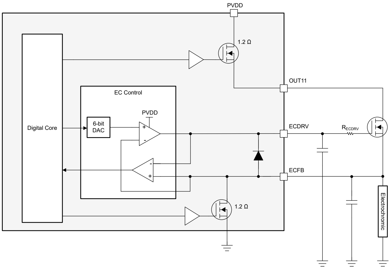
图 7-7. 电致变色驱动器方框图 - 默认配置
