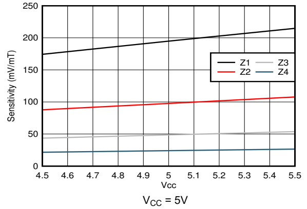
图 5-16. 灵敏度与电源电压之间的关系
