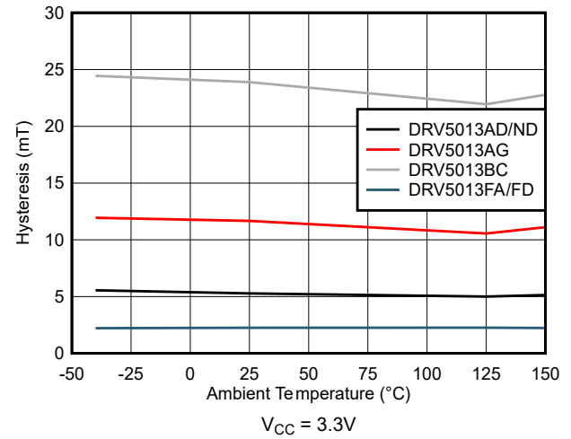
图 5-10. 迟滞与温度间的关系
