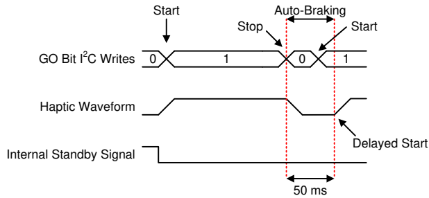
图 7-25. 具有延迟启动的 GO 位触发器 ( RTP 或波形序列发生器 )
