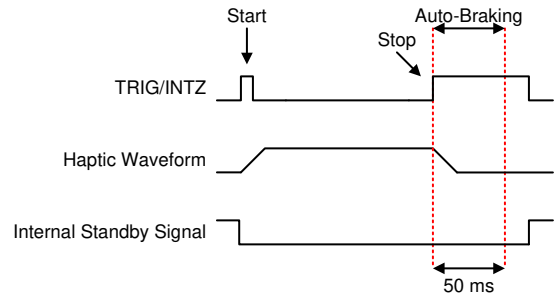
图 7-26. TRIG/INTZ 引脚保持高电平时的触发脉冲行为 ( RTP 或波形序列发生器 )
