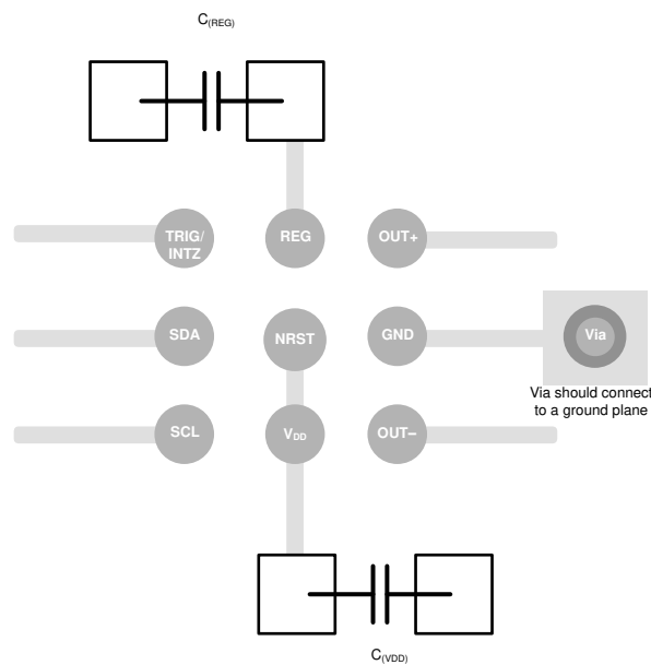
图 9-11. 不带 NRST 功能的布局
