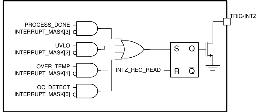
图 7-6. 中断模式下的 TRIG/INTZ 功能
