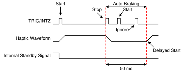
图 7-24. 触发脉冲和忽略脉冲的延迟启动 ( RTP 或波形序列发生器 )
