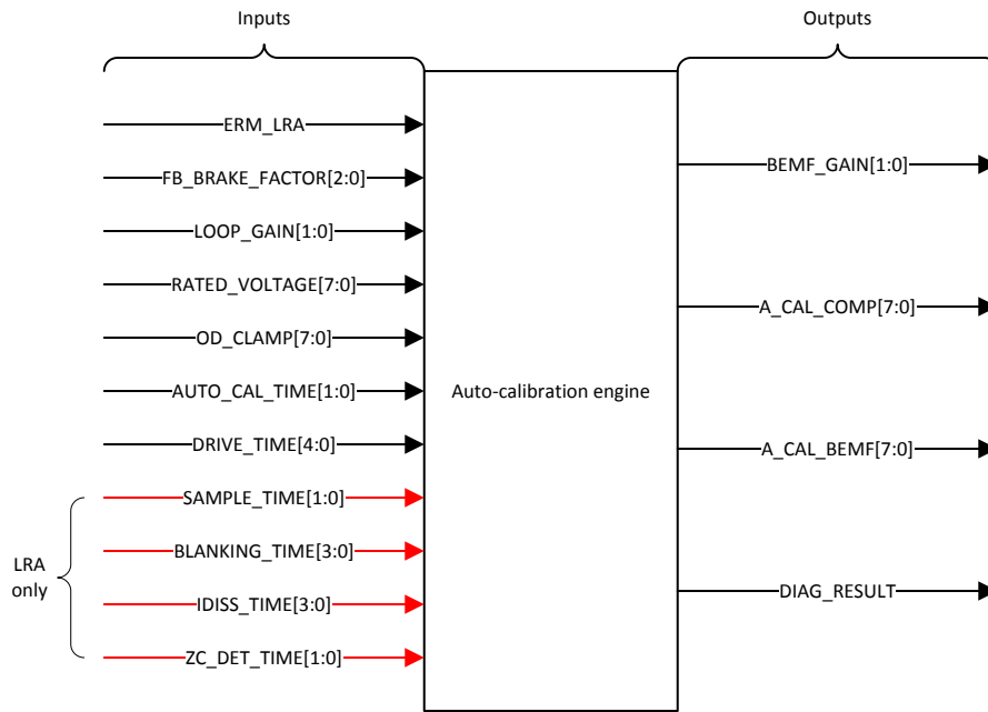
图 7-13. 校准引擎功能图
