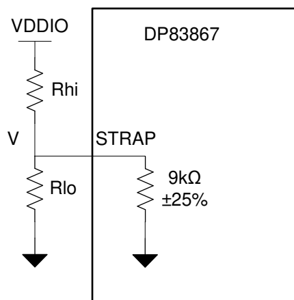
图 7-10. Strap Circuit
