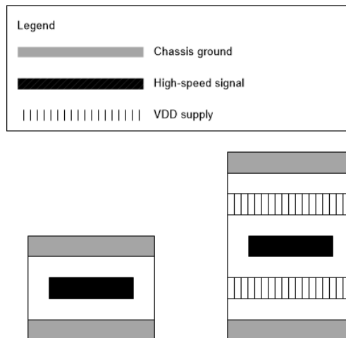
图 8-13. Alternative Layer Stack Up
