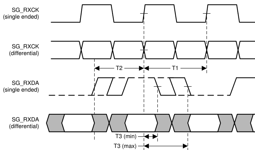
图 6-4. SGMII Timing
