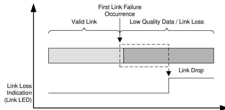
图 6-6. 快速链路丢失
