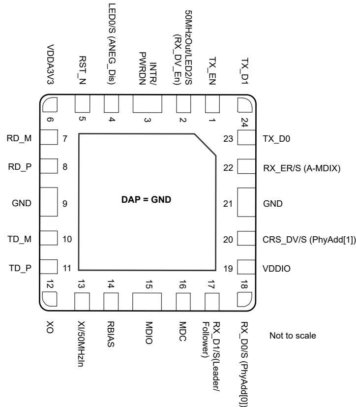
图 4-1. DP83825 RMQ 封装 24 引脚 QFN 顶视图
