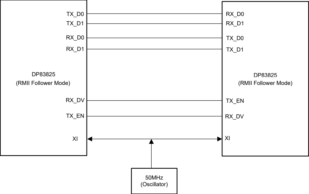
图 6-4. RMII 中继器模式
