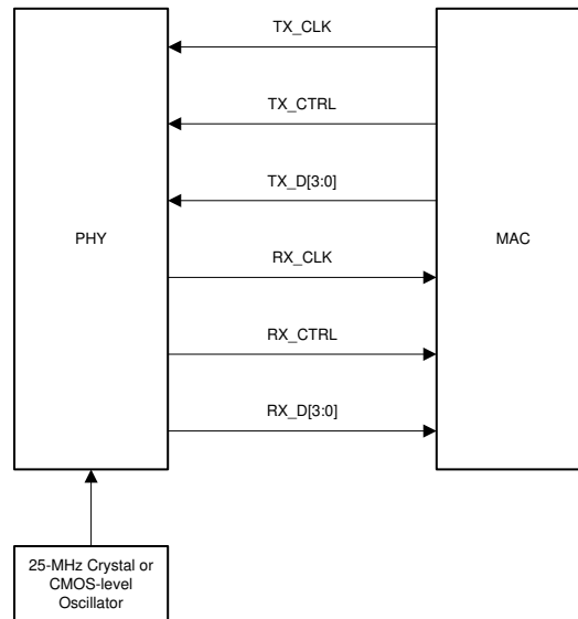
图 8-7. RGMII Signaling
