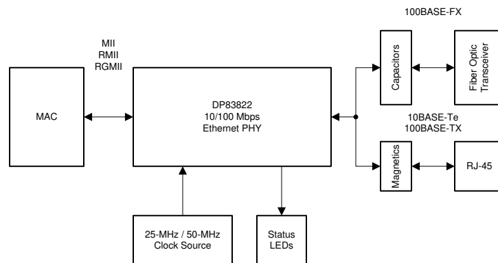
简化原理图
