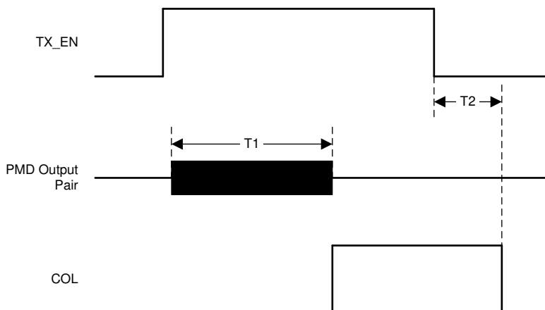
图 7-15. 10BASE-T Jabber Timing
