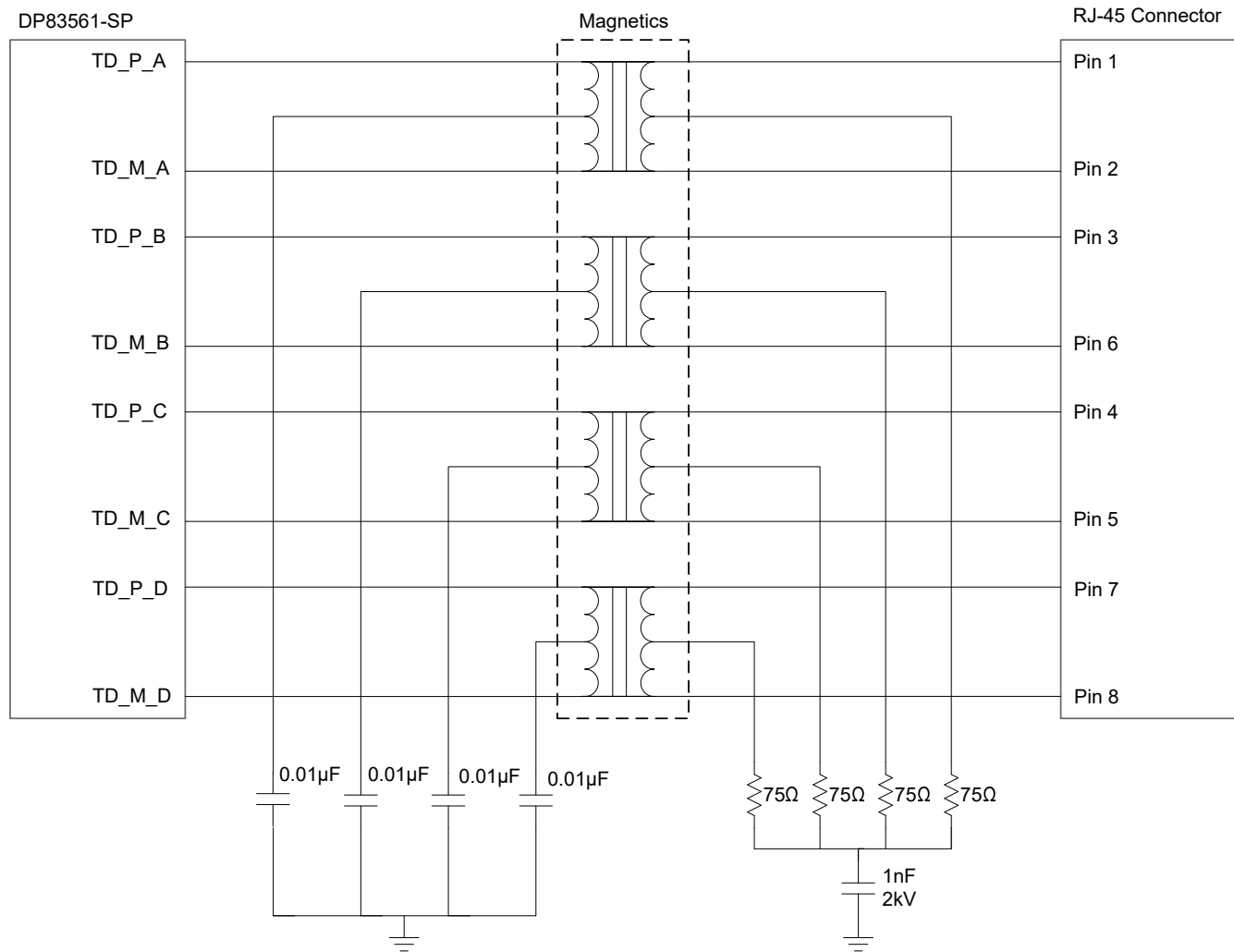
图 8-3. Magnetics Connection
