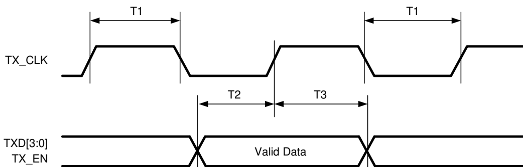
图 6-3. 100-Mbps MII Transmit Timing
