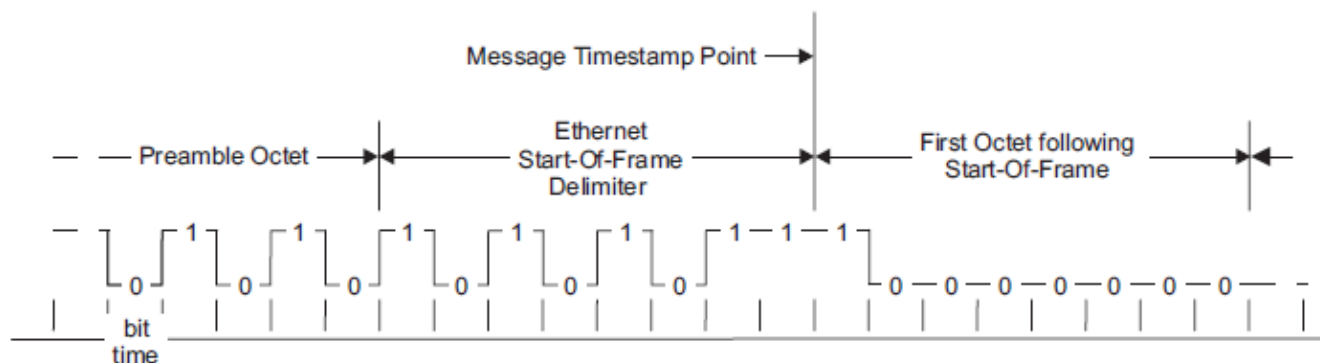
图 7-7. IEEE 1588 Message Timestamp Point
