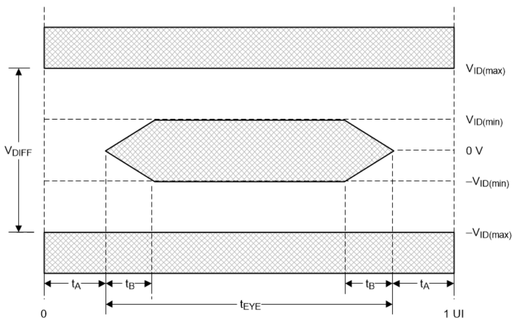
图 5-8. V-By-One 时序
