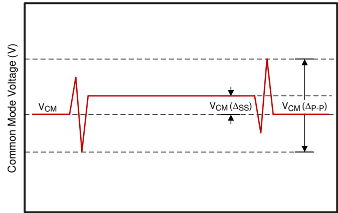
图 6-2. 共模电压
