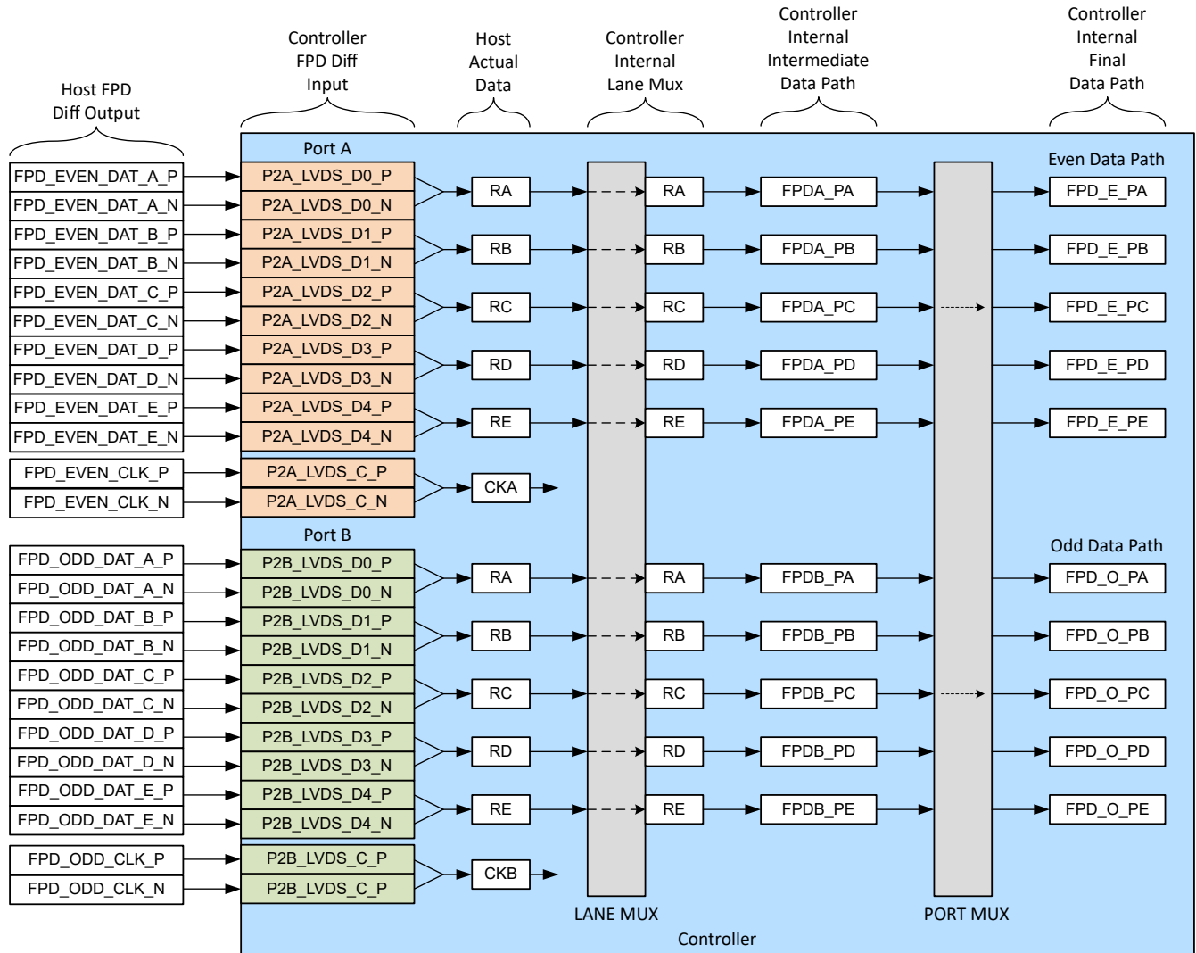
图 7-3. 典型 FPD-Link 端口通道映射示例
