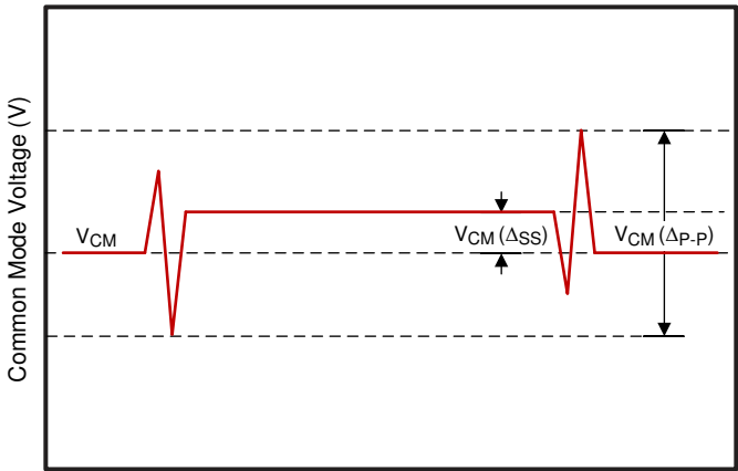
图 6-2. 共模电压
