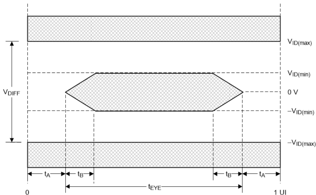
图 6-8. V-By-One 时序
