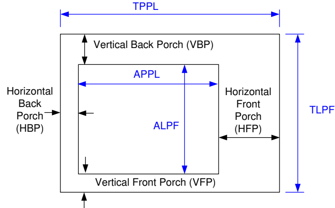
图 10-1. 参数定义
