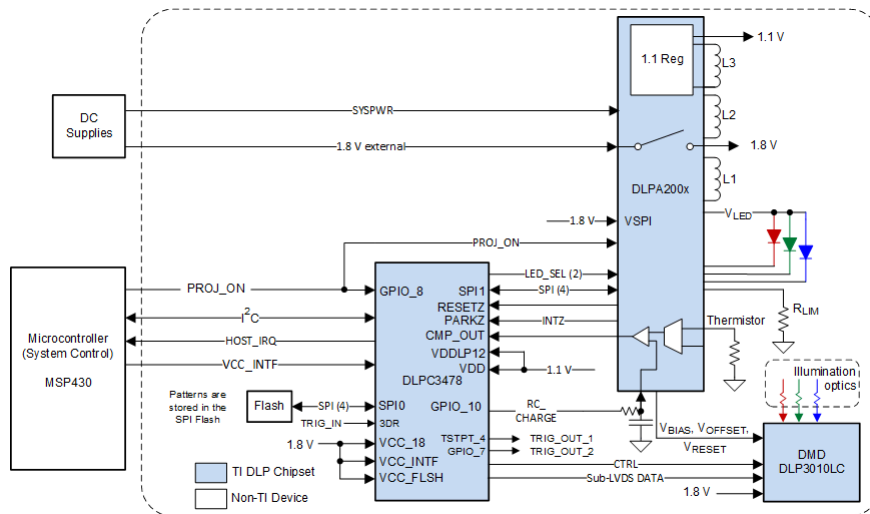
图 7-3. 内部图形流模式
