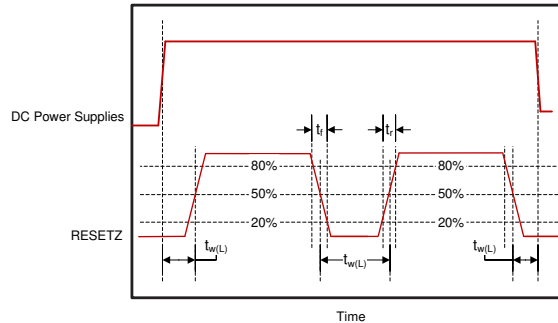
图 5-6. 上电和下电 RESETZ 时序
