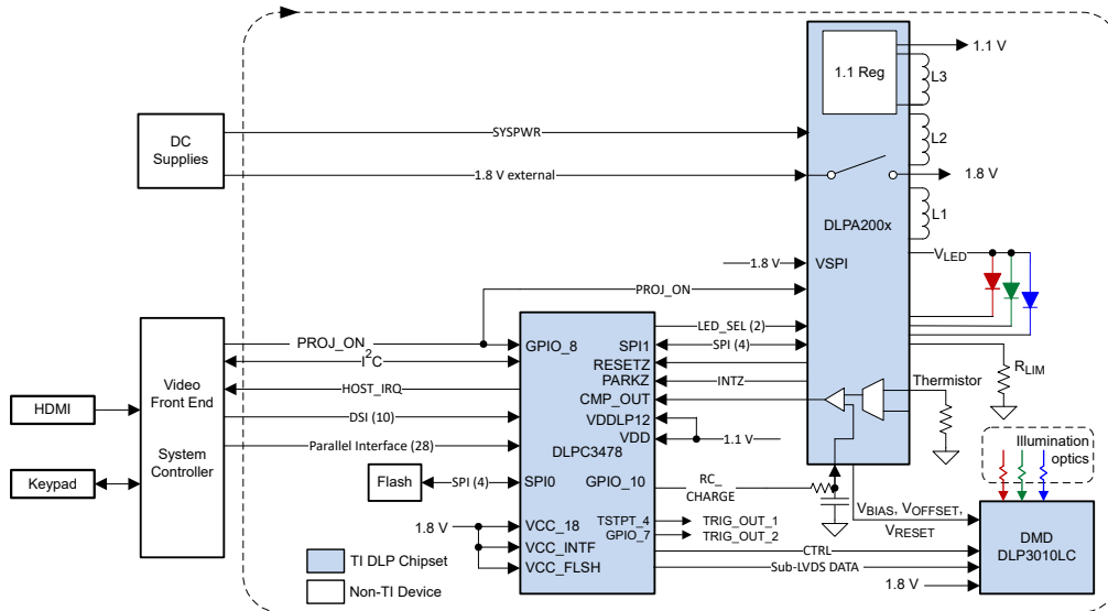
图 7-1. 外部图形流模式
