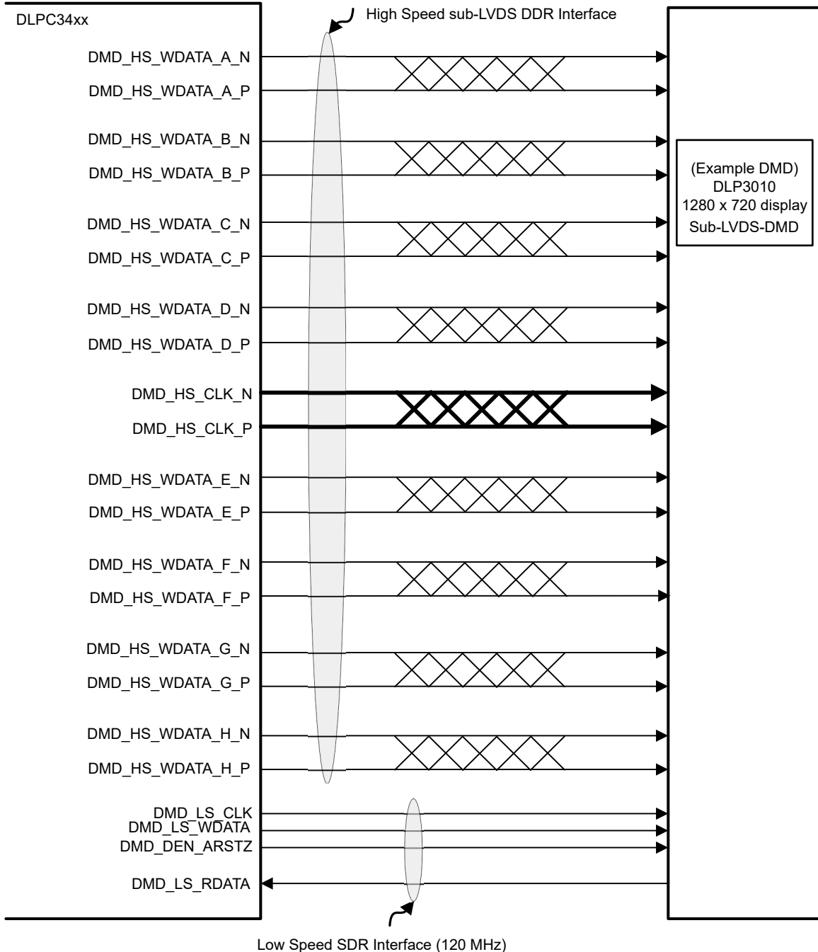
图 6-23. DLP3010LC (.3 720p) DMD 接口示例
