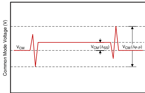
图 5-1. 共模电压
