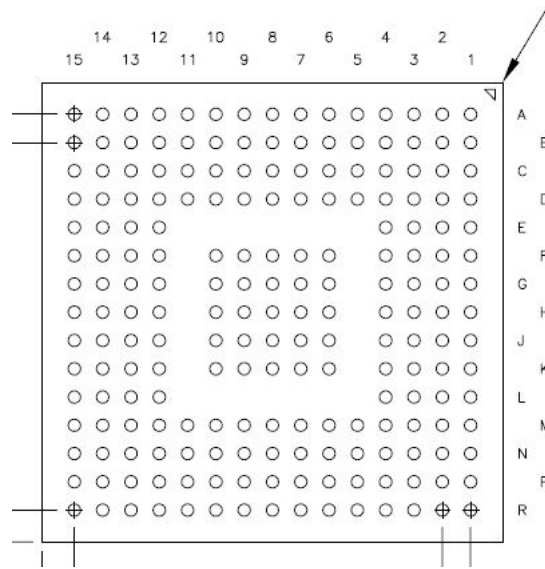
图 4-1. ZEZ 封装 201 引脚 NFBGA 底视图
