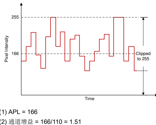
图 6-18. CAIC 处理后颜色通道的像素
