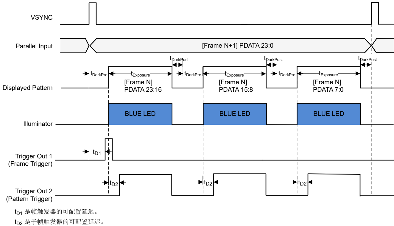
图 6-8. 3 \times 8 位 (蓝色) 图形配置
