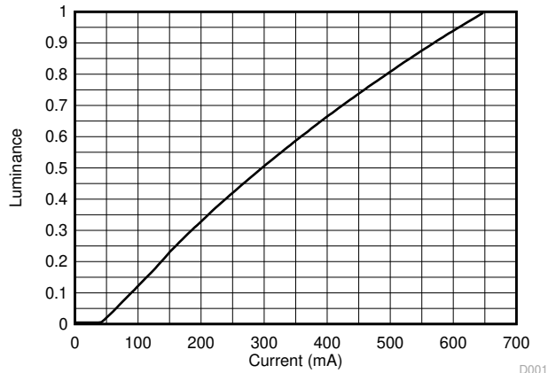
图 7-2. 亮度与电流之间的关系
