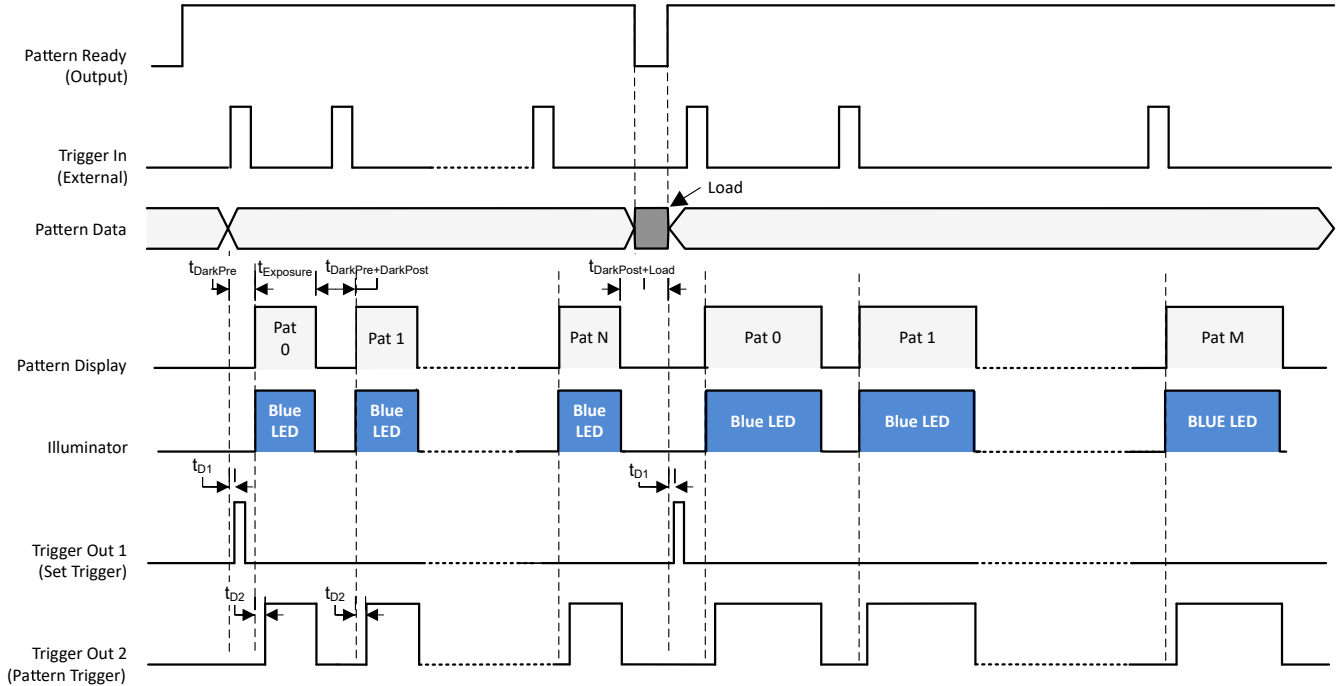
图 6-15. 触发模式
