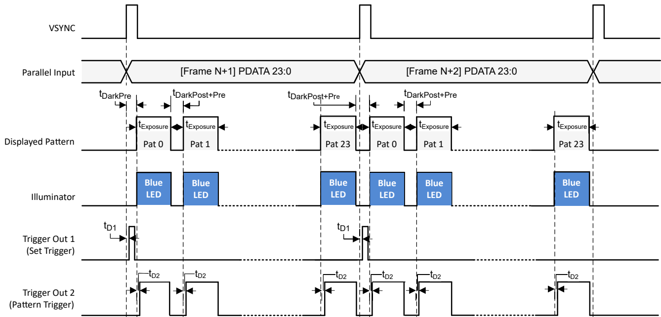
图 6-11. 24 \times 1 位 (蓝色) 图形配置
