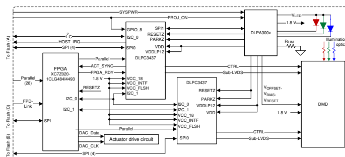
典型简化版系统图
