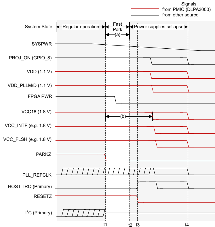
图 9-3. DLPC3437 Fast Power-Down
