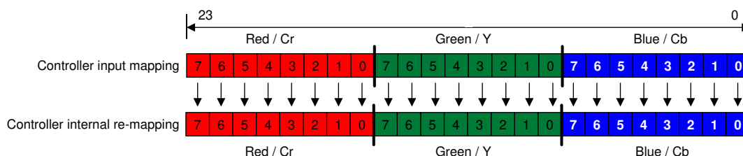
图 7-4. RGB-888 I/O Mapping
