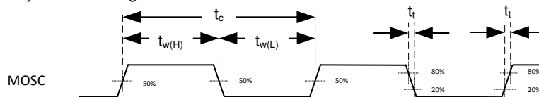
图 5-5. System Oscillators
