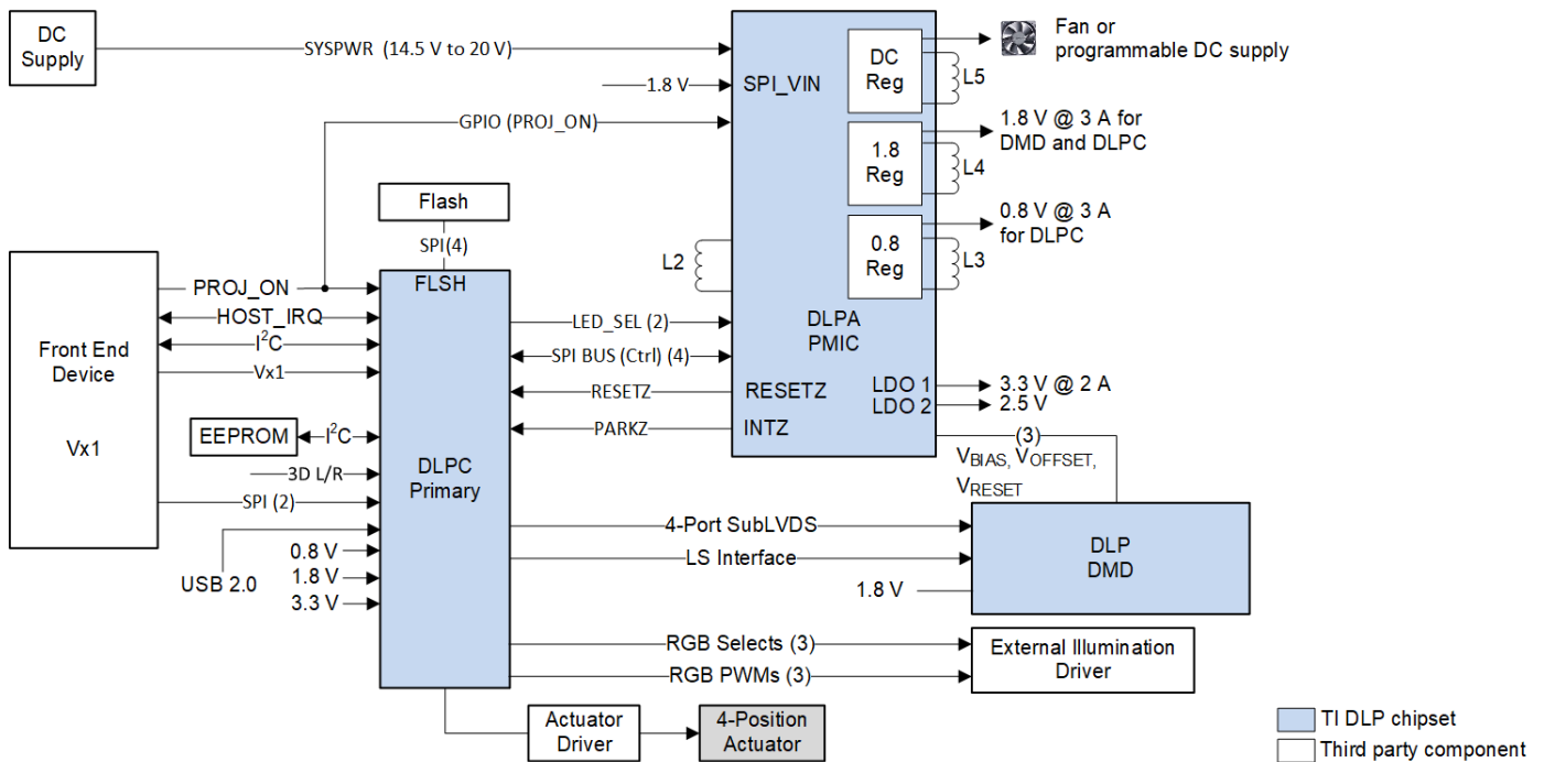
图 7-1. 采用外部照明驱动器的典型 4K+ 超高清系统图
