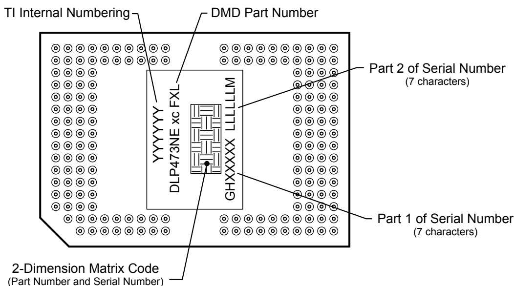
图 9-2. DMD 标识位置
