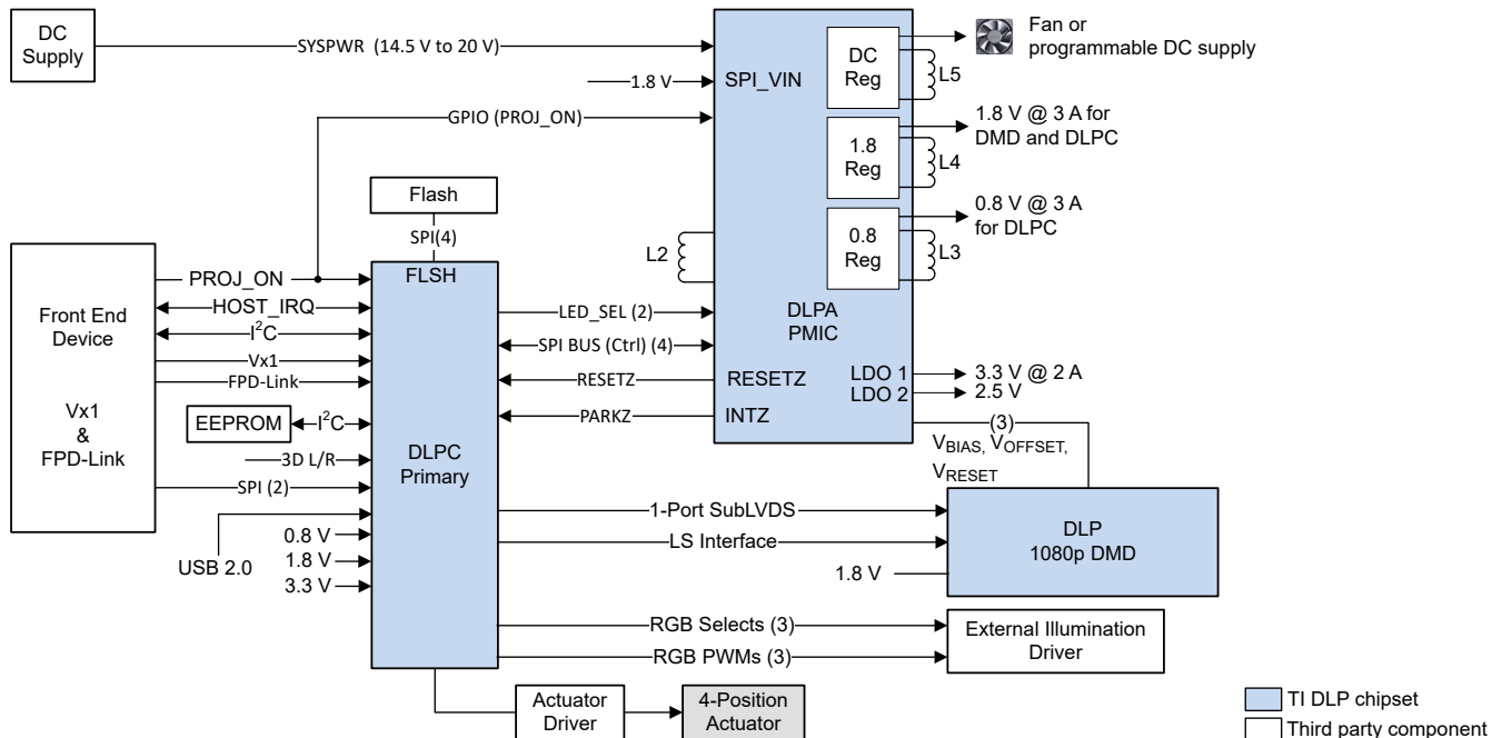
图 7-1. 采用外部照明驱动器的典型 1080p 系统图
