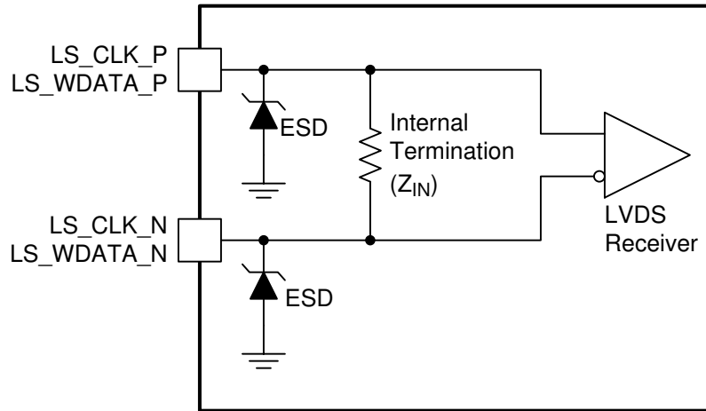
图 5-7. LSIF Equivalent Input
