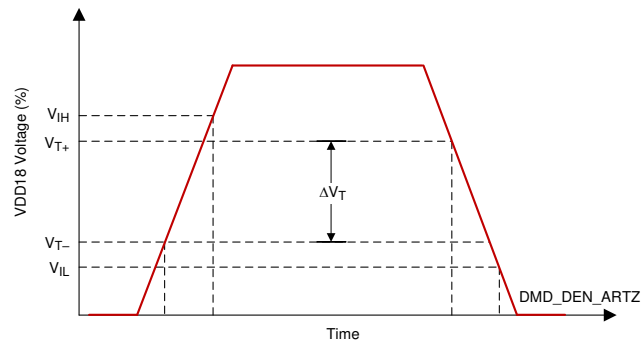
图 5-8. LVCMOS Input Hysteresis
