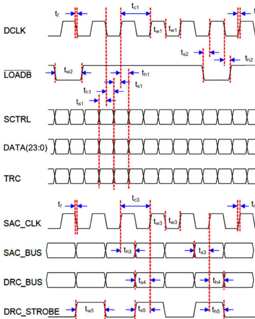
图 7-2. Timing Diagram
