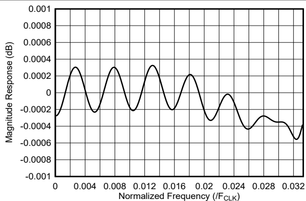
图 7-25. 12 倍内插滤波器通带响应
