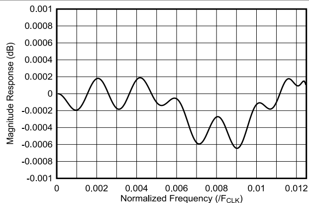
图 7-31. 32 倍内插滤波器通带响应
