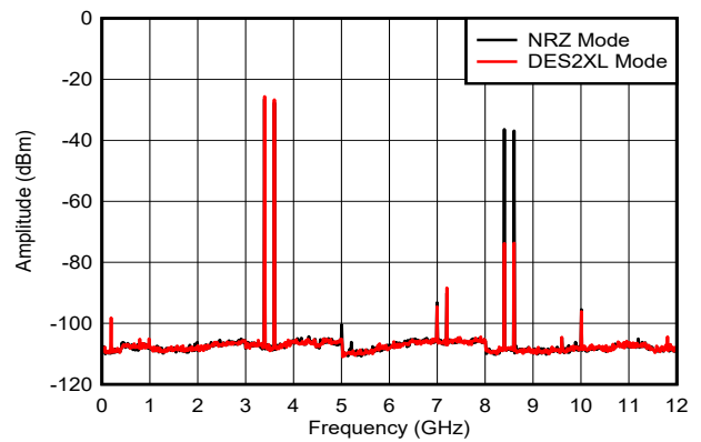
图 6-35. 双音， f_{\text{OUT}} = 3497\text{MHz} ，0dBFS
