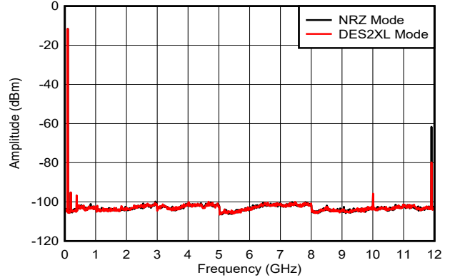
图 6-9. f_{\text{OUT}} = 97\text{MHz} ，-6dBFS
