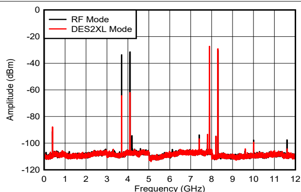
图 6-38. 双音， f_{\text{OUT}} = 8097\text{MHz} ，0dBFS
