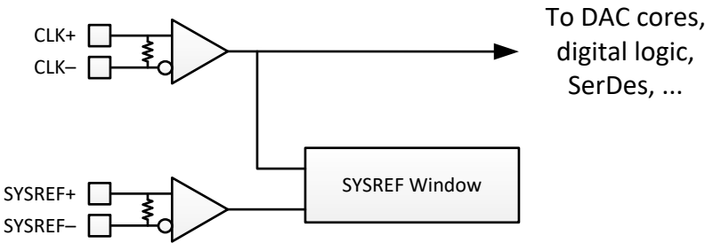
图 7-12. 器件时钟子系统
