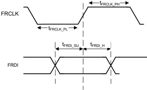
图 6-6. FRDI 时序图
