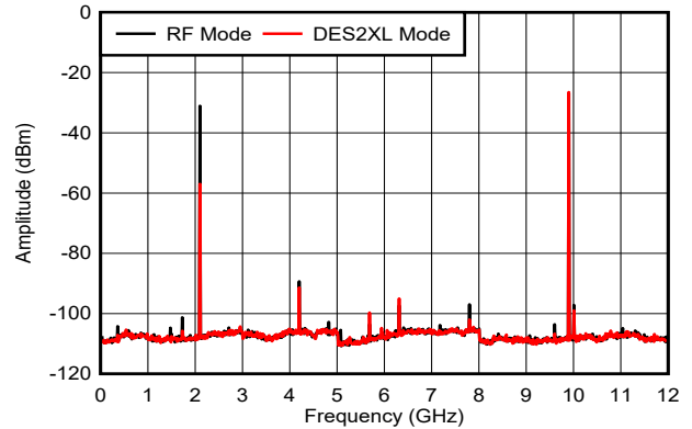
图 6-23. f_{\text{OUT}} = 9897\text{MHz} ，0dBFS
