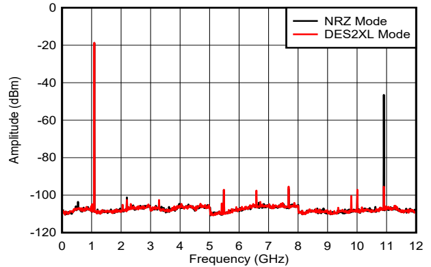
图 6-11. f_{\text{OUT}} = 1097\text{MHz} ，0dBFS
