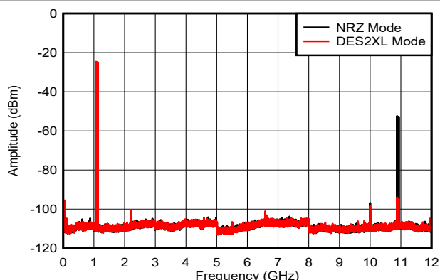
图 6-29. 双音， f_{\text{OUT}} = 1097\text{MHz} ，0dBFS
