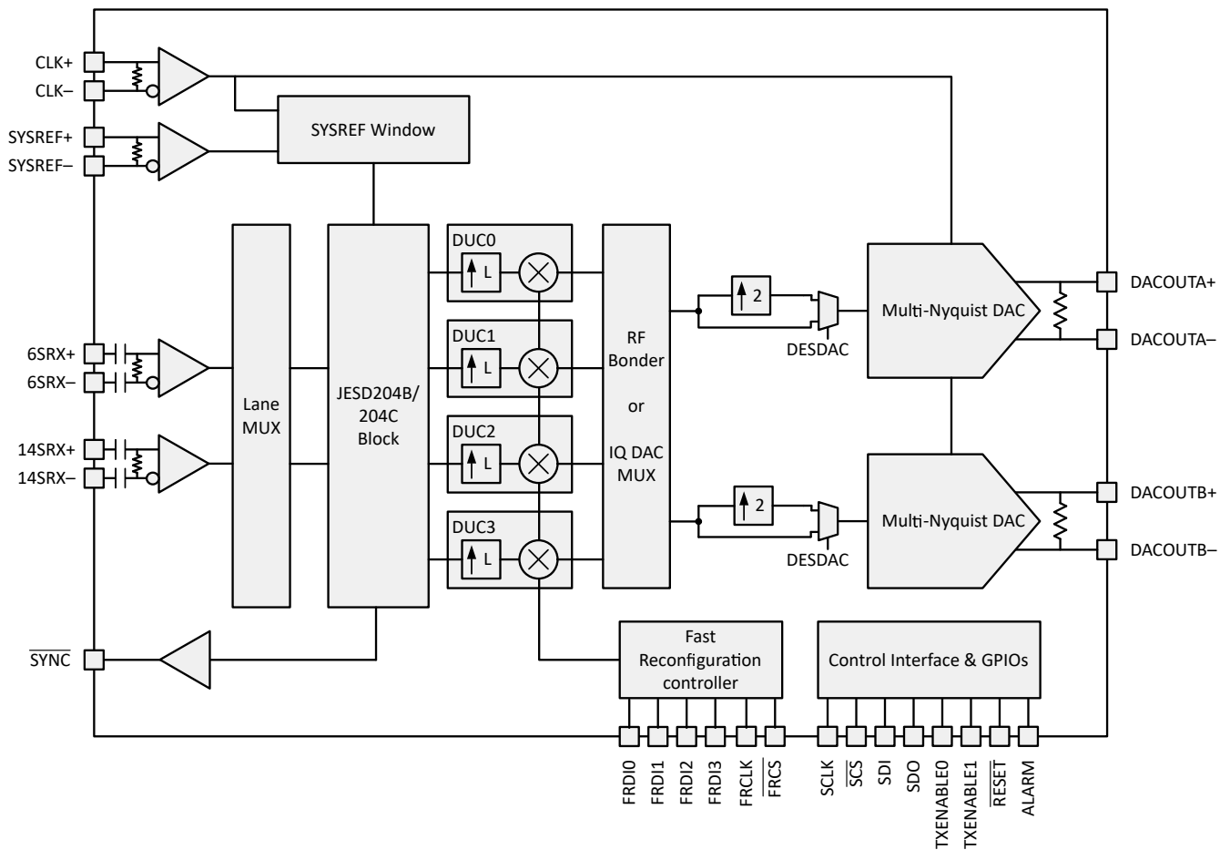
图 7-1. 双通道器件
