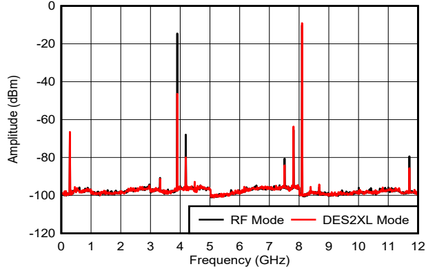
图 6-20. f_{\text{OUT}} = 8097\text{MHz} ，0dBFS
