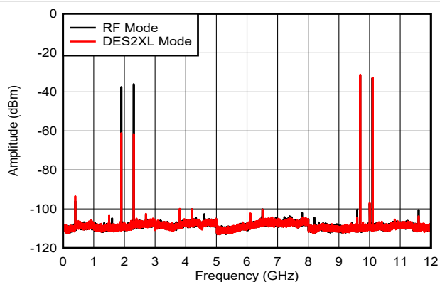
图 6-41. 双音， f_{\text{OUT}} = 9897\text{MHz} ，0dBFS
