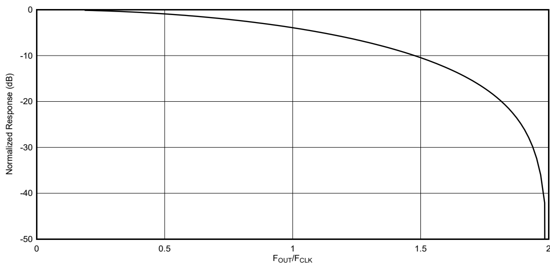
图 7-10. DES 输出频率响应
