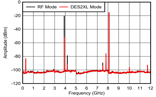
图 6-21. f_{\text{OUT}} = 8097\text{MHz} ，-6dBFS
