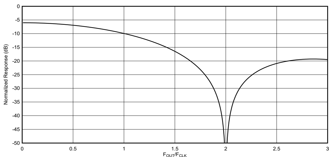
图 7-6. RTZ 模式输出频率响应
