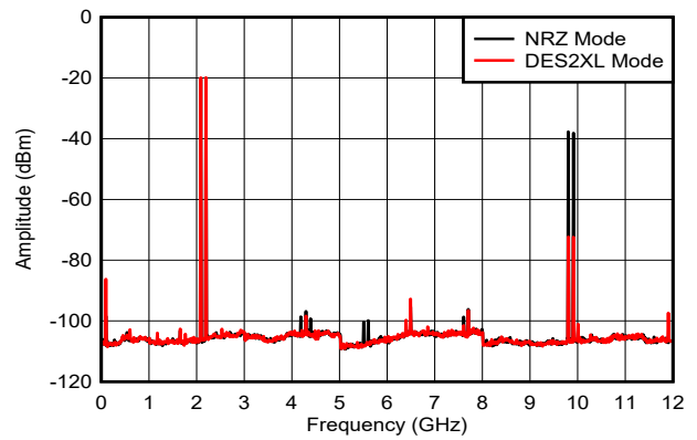
图 6-33. 双音， f_{\text{OUT}} = 2097\text{MHz} ，-6dBFS
