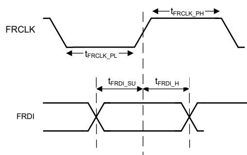
图 6-6. FRDI 时序图
