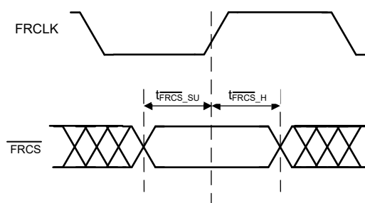
图 6-7. \overline{\text{FRCS}} 时序图
