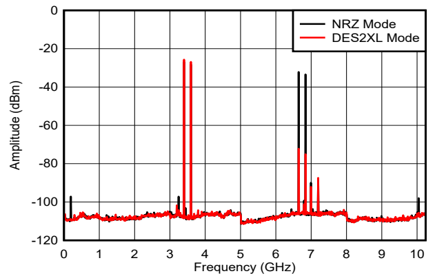
图 6-35. 双音， f_{\text{OUT}} = 3497\text{MHz} ，0dBFS
