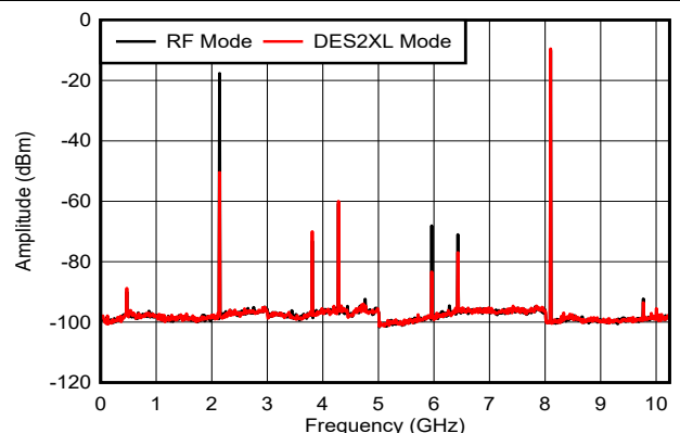
图 6-21. f_{\text{OUT}} = 5997\text{MHz} ，-6dBFS
