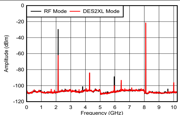
图 6-23. f_{\text{OUT}} = 8097\text{MHz} ，0dBFS
