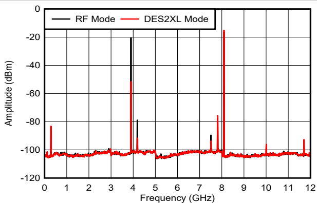
图 6-21. f_{\text{OUT}} = 8097\text{MHz} ，-6dBFS
