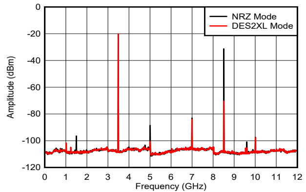
图 6-17. f_{\text{OUT}} = 3497\text{MHz} ，0dBFS
