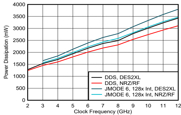
双路 DAC、 I_{\text{FS\_SWITCH}} = 20.5\text{mA}
