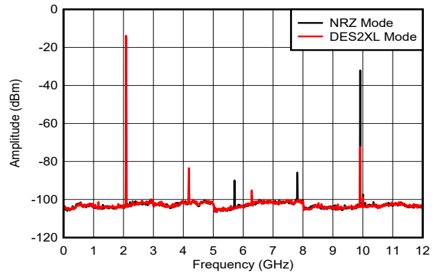
图 6-15. f_{\text{OUT}} = 2097\text{MHz} ，-6dBFS
