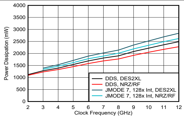
单路 DAC、 I_{\text{FS\_SWITCH}} = 41\text{mA}
