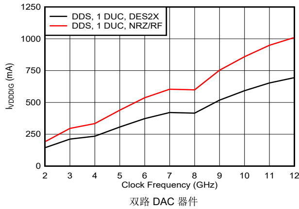
图 6-58. VDDDIG 电流与时钟频率和 DAC 模式间的关系
