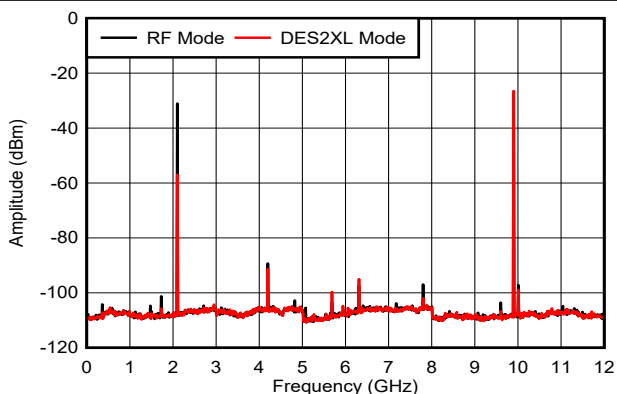
图 6-23. f_{\text{OUT}} = 9897\text{MHz} ，0dBFS
