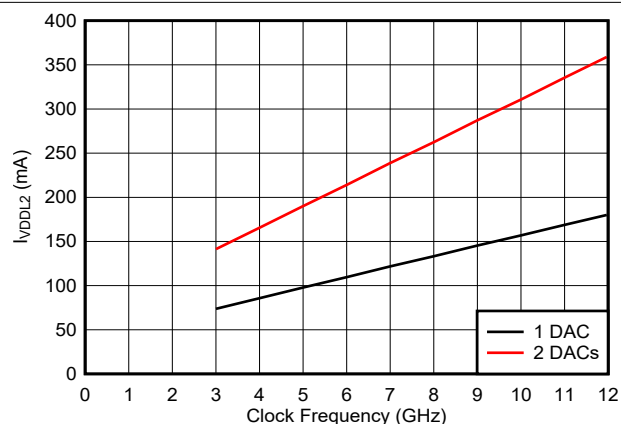
图 6-51. VDDLx 电流与时钟频率间的关系
