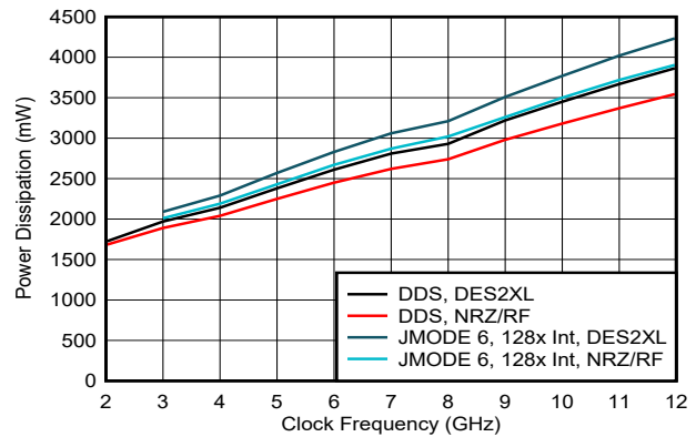
双路 DAC、 I_{\text{FS\_SWITCH}} = 41\text{mA}
