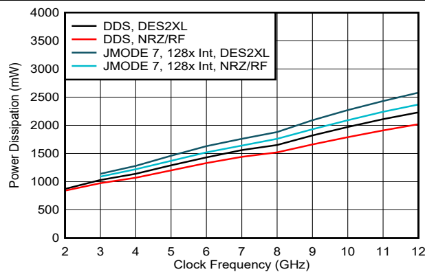
单路 DAC、 I_{\text{FS\_SWITCH}} = 20.5\text{mA}
