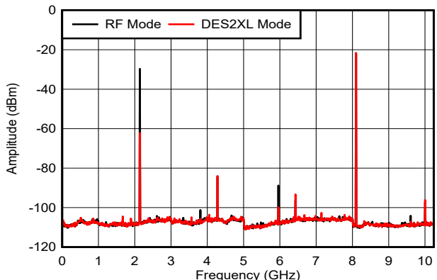
图 6-23. f_{\text{OUT}} = 8097\text{MHz} ，0dBFS
