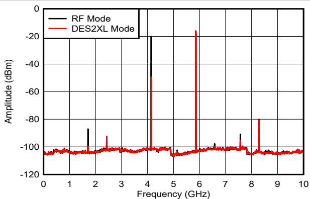
图 6-21. f_{\text{OUT}} = 5997\text{MHz} ，-6dBFS
