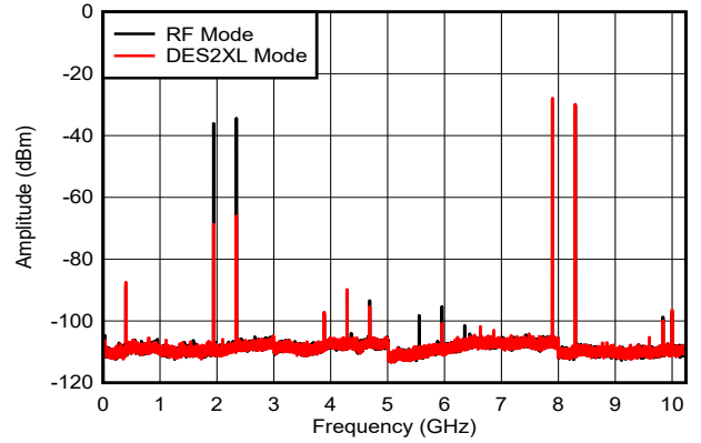
图 6-43. 双音， f_{\text{OUT}} = 8097\text{MHz} ， -12\text{dBFS}
