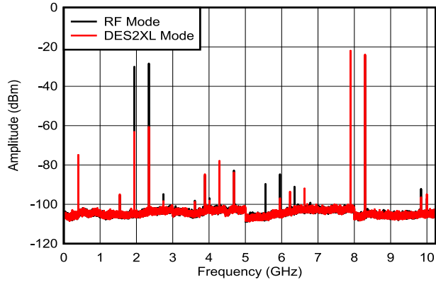
图 6-42. 双音， f_{\text{OUT}} = 8097\text{MHz} ， -6\text{dBFS}
