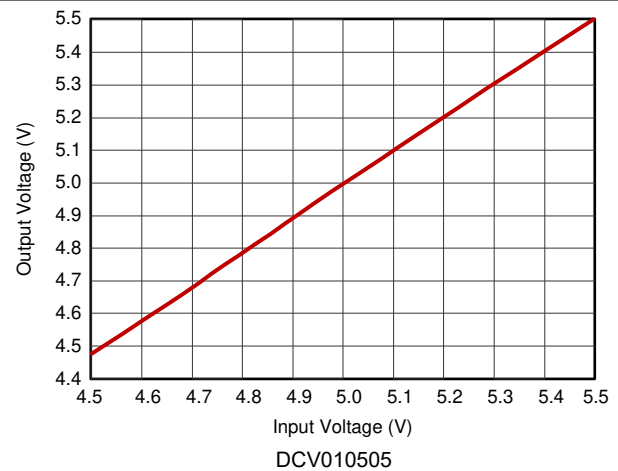
图 7-4. Line Regulation
