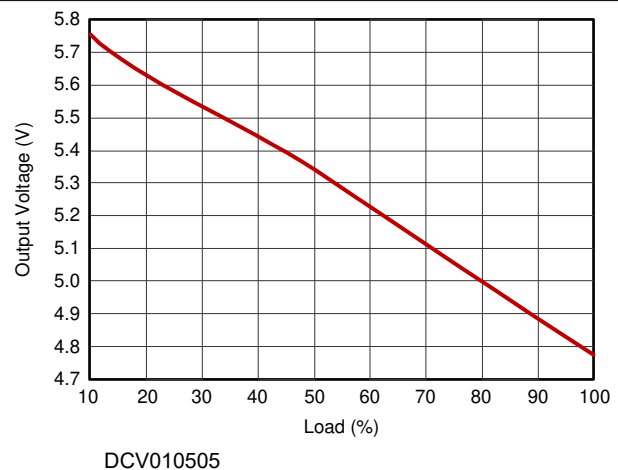
图 7-6. Load Regulation
