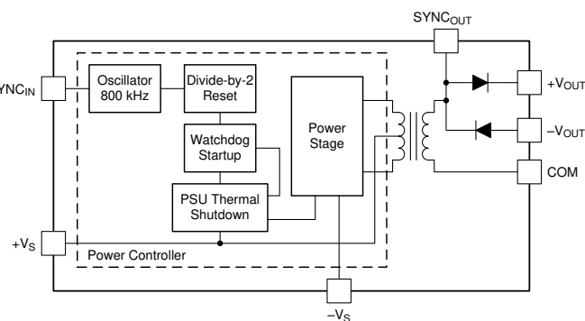
双路输出方框图
