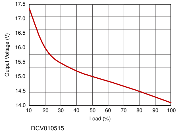
图 7-14. Load Regulation
