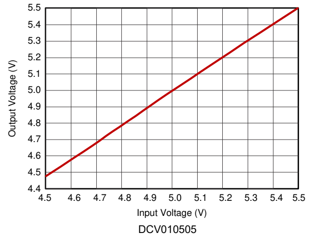
图 7-4. Line Regulation
