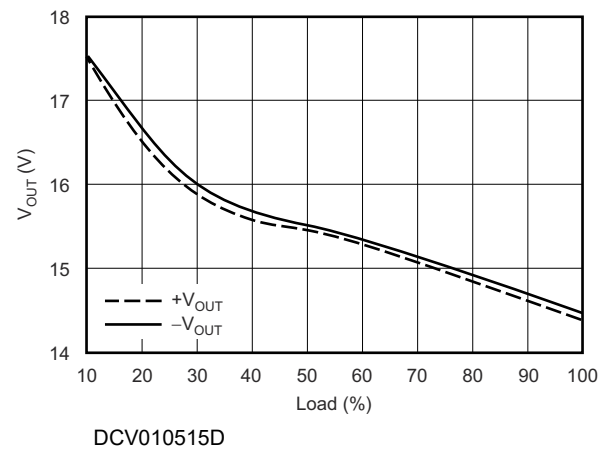
图 7-16. Load Regulation
