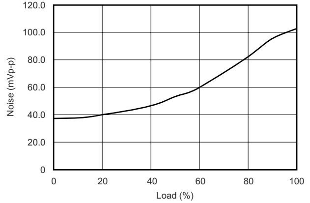
图 7-14. Output Voltage Noise
