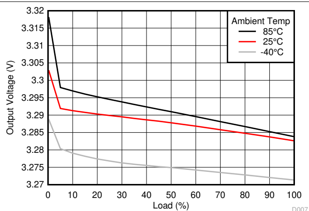
图 7-8. Load Regulation
