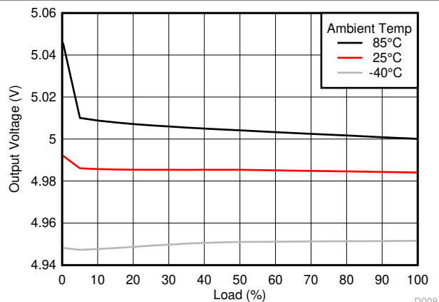
图 7-8. Load Regulation
