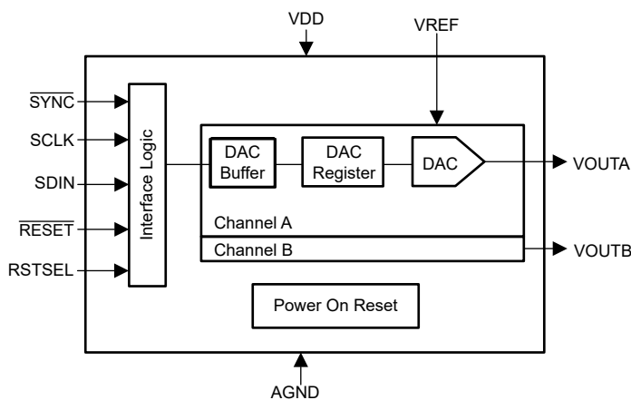
功能方框图
