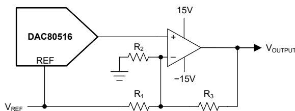
图 8-1. 使用 DAC80516 实现双极运行
