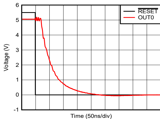
图 5-35. 干扰脉冲, 下降沿
