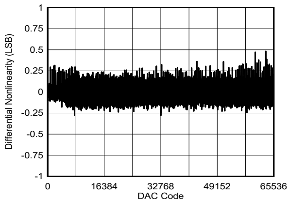
图 5-4. 微分非线性与数字输入代码间的关系
