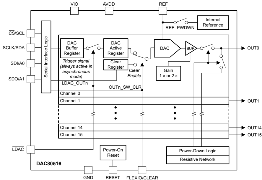
功能方框图
