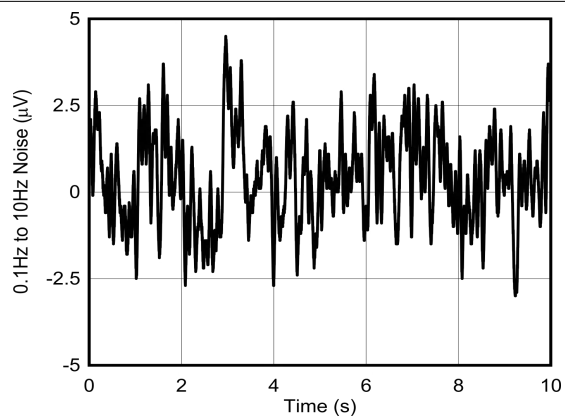
图 5-51. 内部基准噪声
