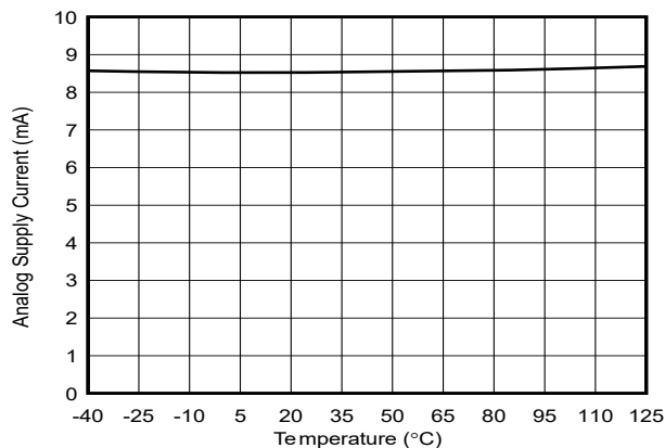
图 5-23. 采用内部基准时的电源电流与温度间的关系
