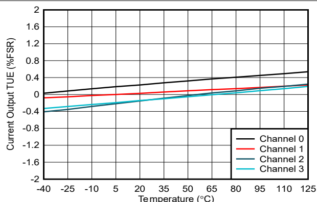
图 5-38. 电流输出 TUE 与温度间的关系
