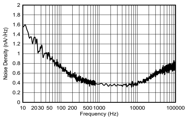
图 5-49. 电流输出噪声密度
