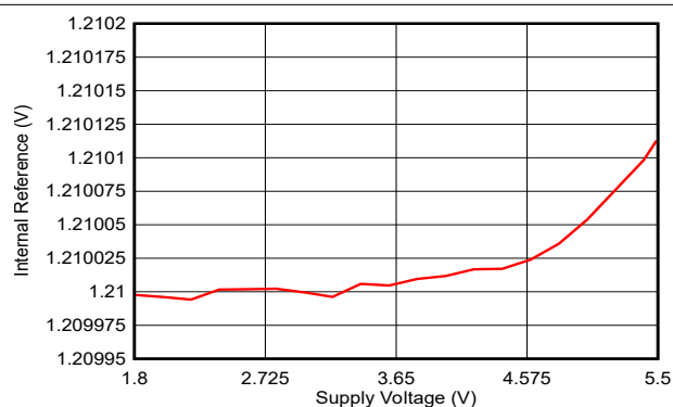
图 5-55. 内部基准与电源电压间的关系
