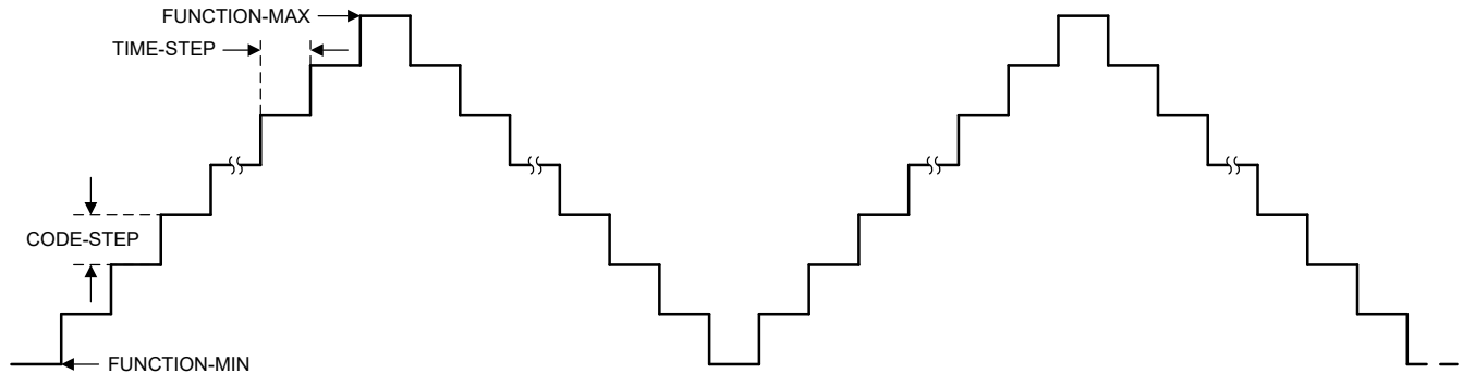
图 6-12. 三角波形
