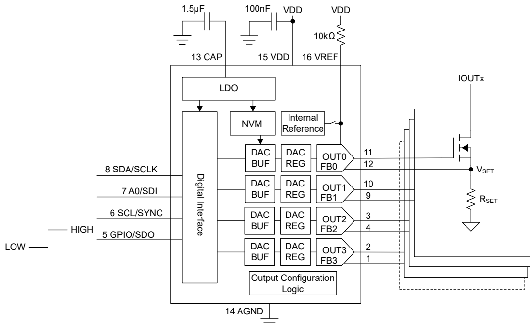
图 8-1. 电流源
