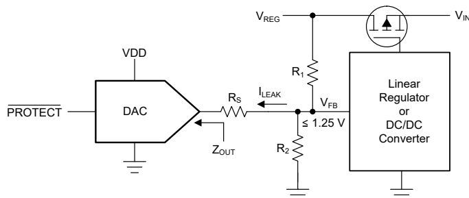
图 6-9. 高阻抗 (高阻态) 输出和 \overline{\text{PROTECT}} 输入
