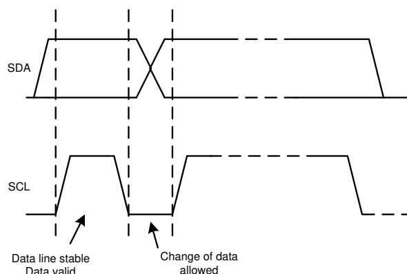
图 6-22. 在 I 2 C 总线上的位传输
