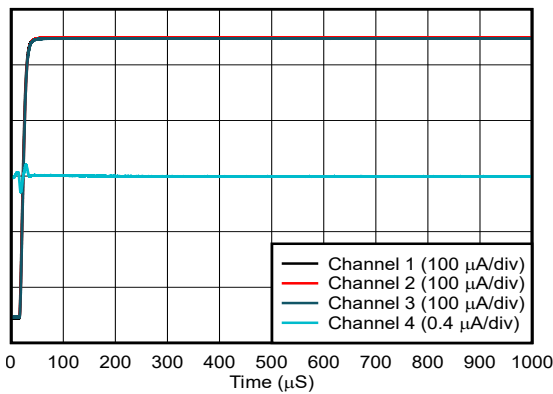
图 5-45. 电流输出上电干扰
