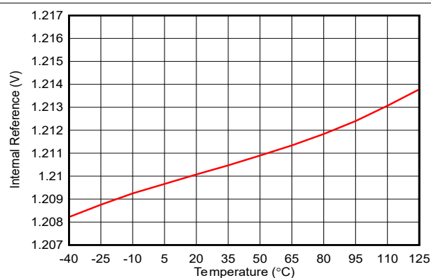
图 5-54. 内部基准与温度间的关系
