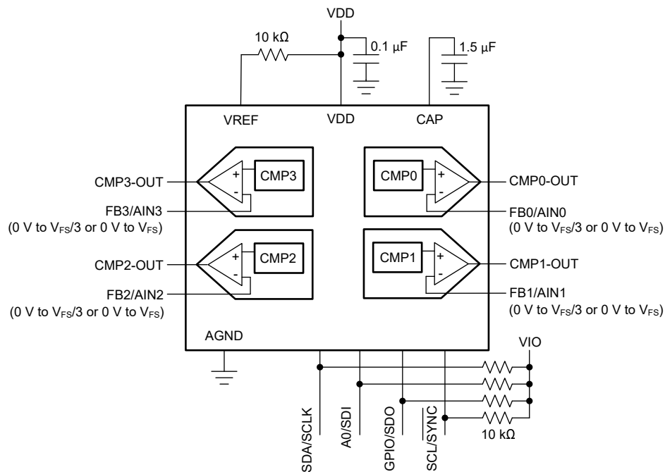
图 6-3. 比较器接口
