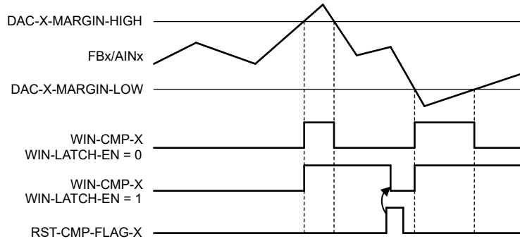
图 6-8. 窗口比较器操作
