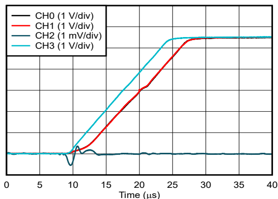
图 5-23. 电压输出上电干扰
