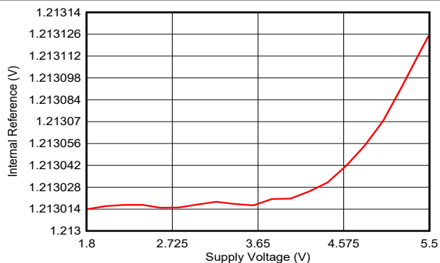
图 6-55. 内部基准与电源电压间的关系
