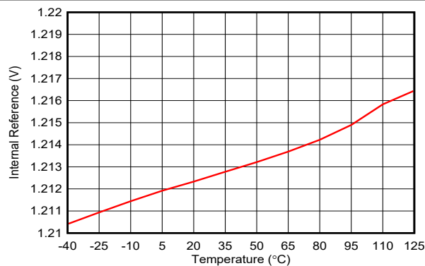
图 6-54. 内部基准与温度间的关系
