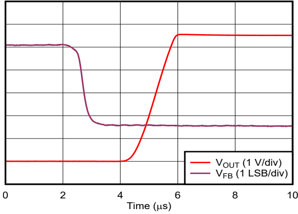
图 6-51. 比较器响应时间：低电平到高电平转换
