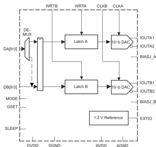
功能模块图
