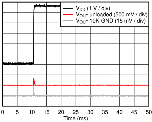
图 6-40. Power-on Glitch
