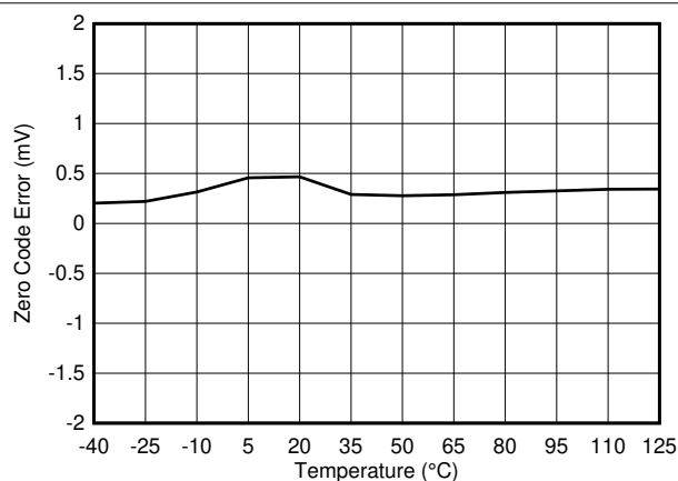
图 6-8. Zero Code Error vs Temperature
