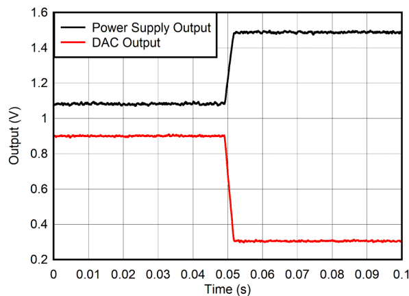
图 8-2. Power-Supply Margin High
