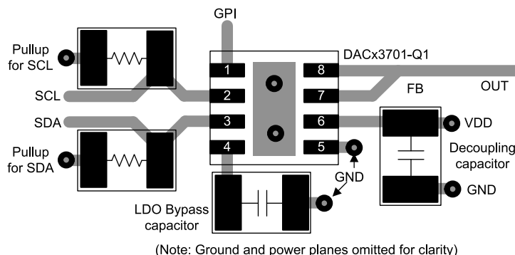
图 8-6. Layout Example
