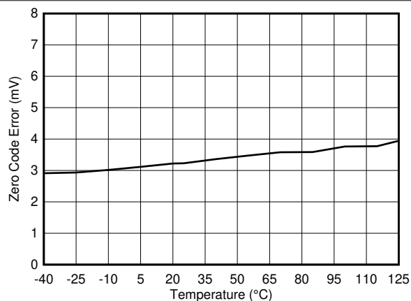
图 6-18. Zero Code Error vs Temperature
