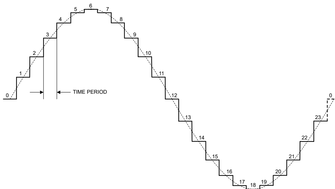
图 7-12. 正弦波生成
