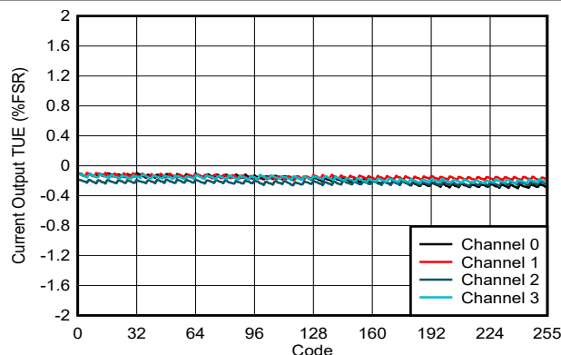
图 6-37. 电流输出 TUE 与数字输入代码间的关系
