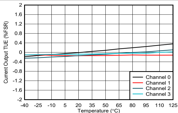
图 6-38. 电流输出 TUE 与温度间的关系
