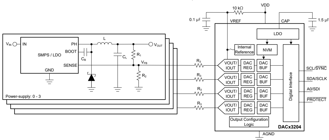
使用 DACx3204 实现电压裕量和调节
