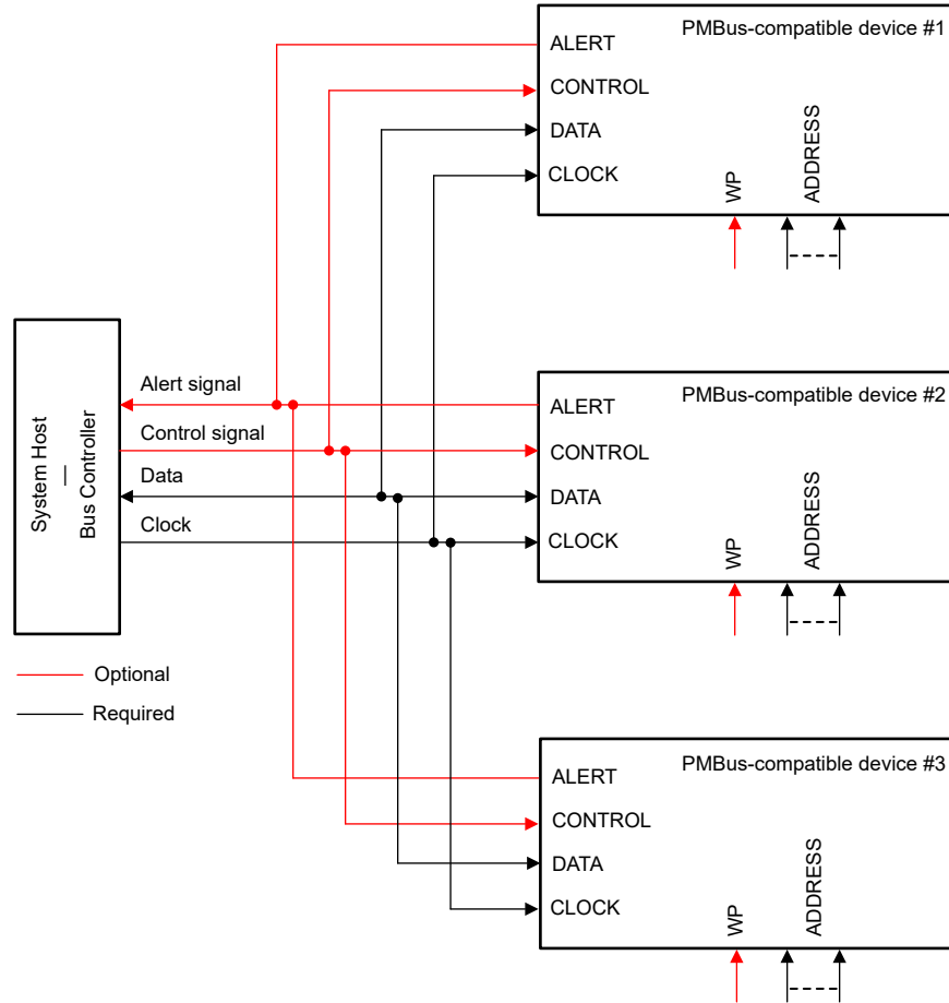
图 7-11. PMBus 连接
