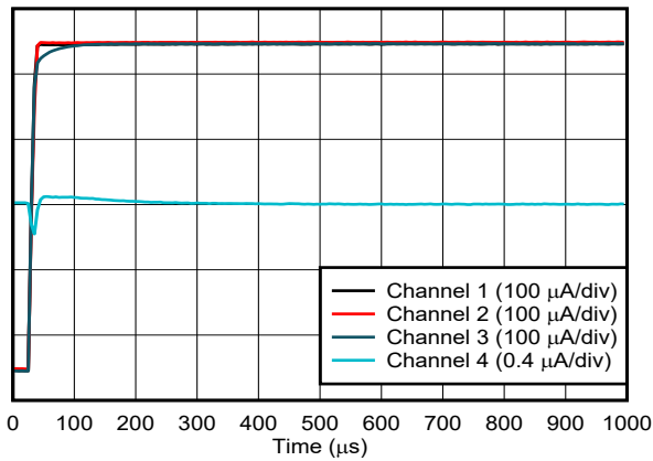
图 6-45. 电流输出加电干扰
