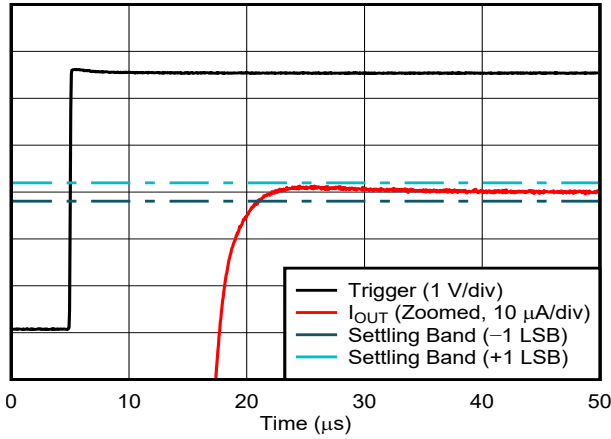
图 6-43. 电流输出建立时间 (上升沿)
