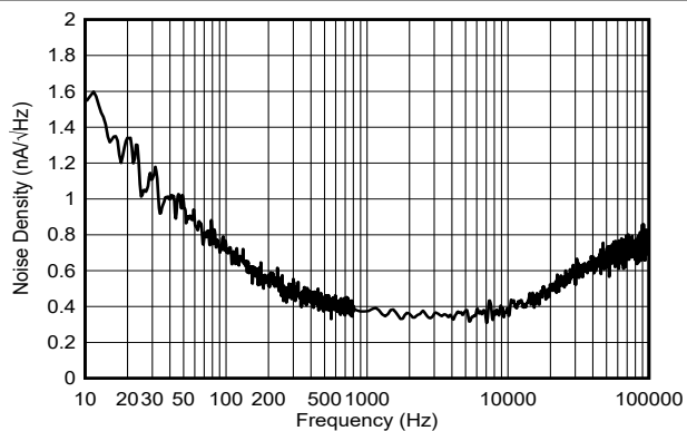
图 6-49. 电流输出噪声密度
