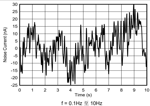
图 6-50. 电流输出闪烁噪声
