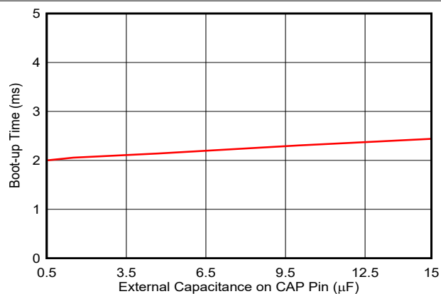
图 6-57. 启动时间与 CAP 引脚上电容间的关系
