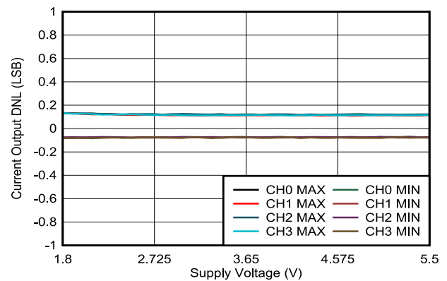
图 6-36. 电流输出 DNL 与电源电压间的关系
