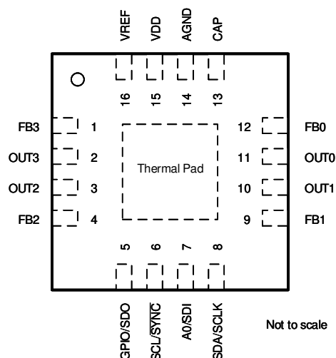
图 5-1. RTE 封装、16 引脚 WQFN，俯视图
