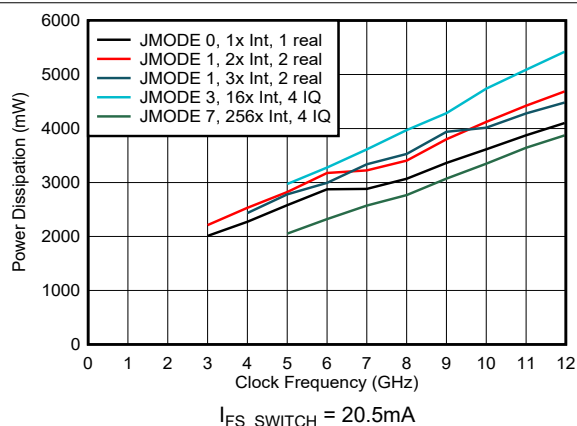
图 6-203. 功率损耗与时钟频率和数字模式间的关系
