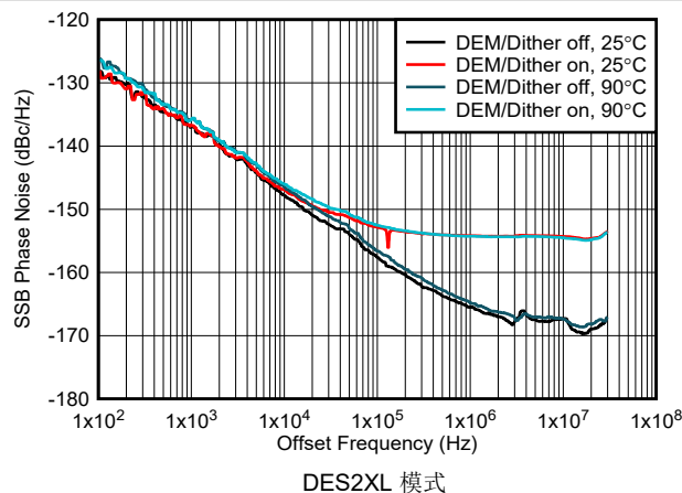
图 6-197. 1GHz 条件下相位噪声与偏移频率间的关系
