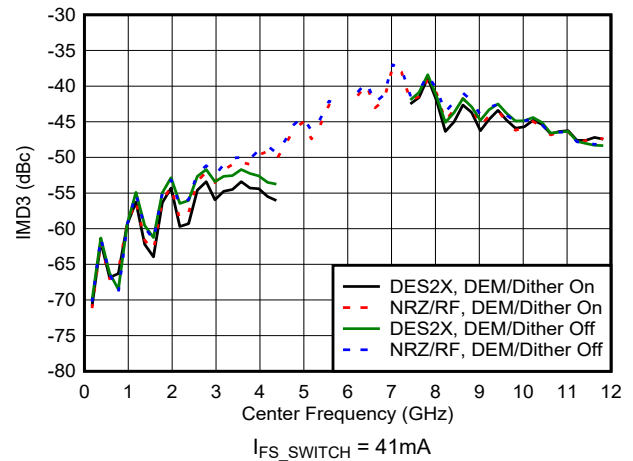
图 6-85. IMD3 与频率和模式间的关系
