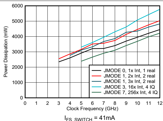
图 6-204. 功率损耗与时钟频率和数字模式间的关系
