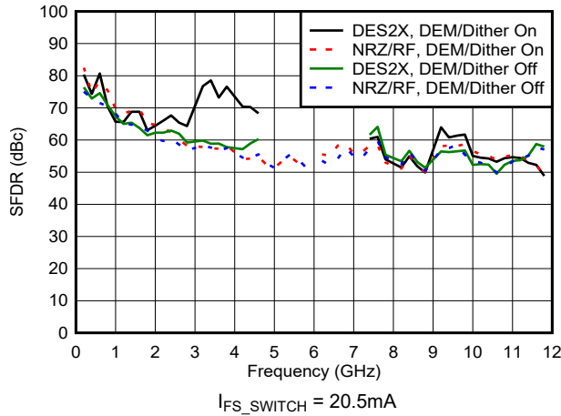
图 6-82. SFDR 与频率和模式间的关系
