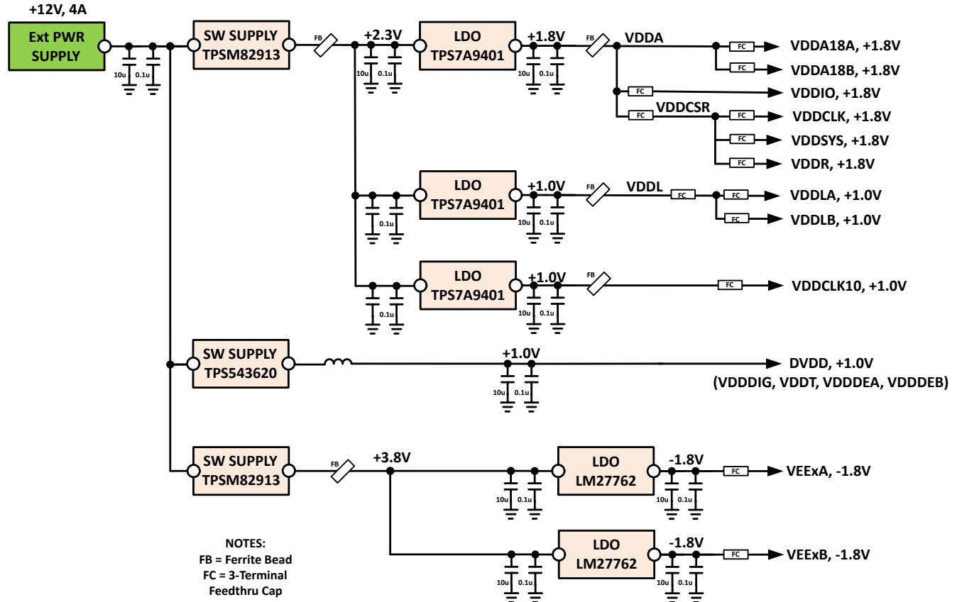
图 8-22. 推荐的电源方框图
