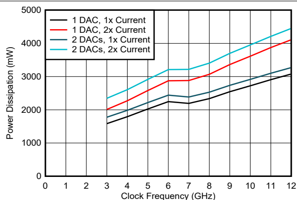
图 6-205. 功率损耗与时钟频率以及 DAC 模式间的关系
