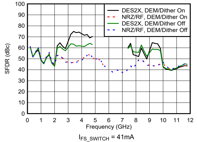
图 6-83. SFDR 与频率和模式间的关系
