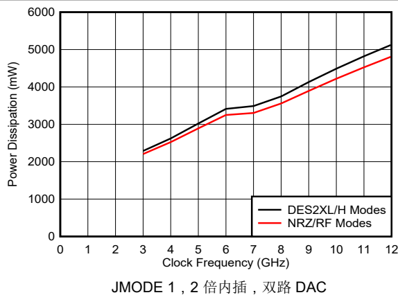
图 6-206. 功率损耗与时钟频率以及 DAC 模式间的关系
