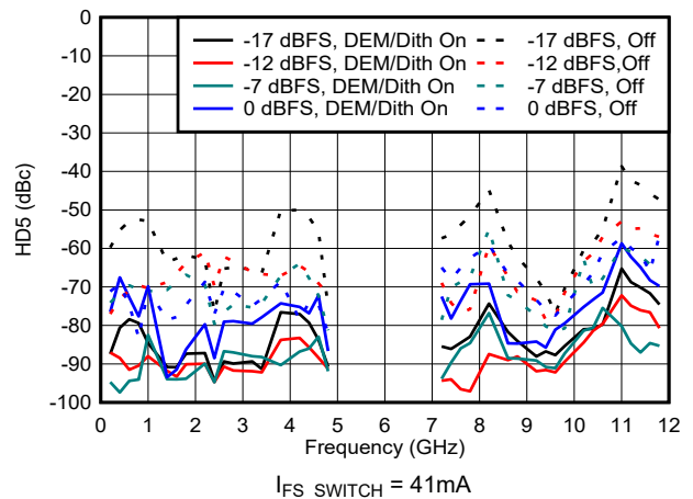
图 6-181. DES2X 模式下 HD5 与频率和数字振幅间的关系
