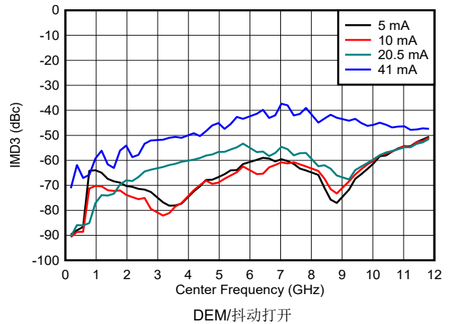
图 6-107. NRZ/RF 模式下 IMD3 与频率和输出电流间的关系
