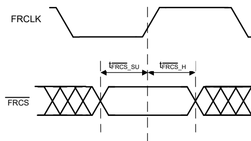
图 6-7. \overline{FRCS} 时序图
