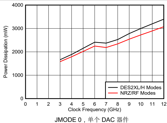
图 6-205. 功率损耗与时钟频率以及 DAC 模式间的关系
