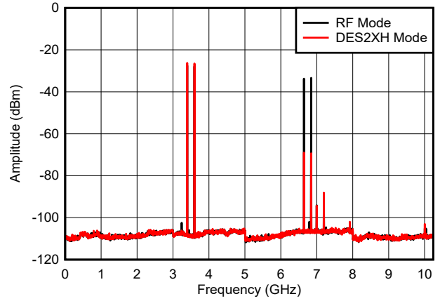
图 6-37. 双音， f_{\text{OUT}} = 3497\text{MHz} ，-12dBFS
