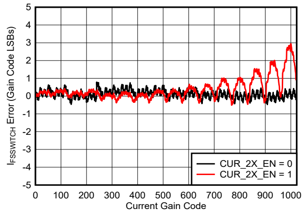
图 6-15. I_{\text{FS\_SWITCH}} 与增益代码间的关系
