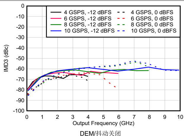
图 6-130. NRZ/RF 模式下 IMD3 与频率和采样速率间的关系
