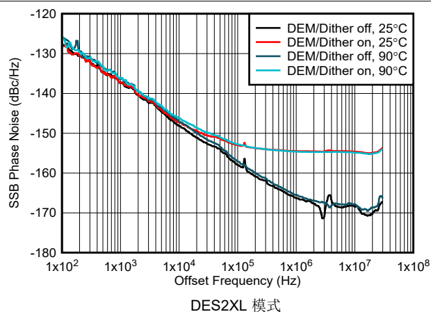
图 6-205. 1GHz 条件下相位噪声与偏移频率间的关系
