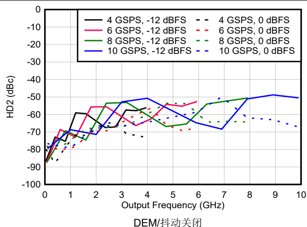
图 6-156. DES2X 模式下 HD2 与频率和采样速率间的关系
