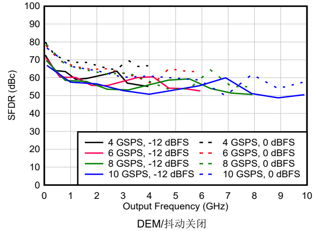
图 6-112. DES2X 模式下 SFDR 与频率和采样速率间的关系
