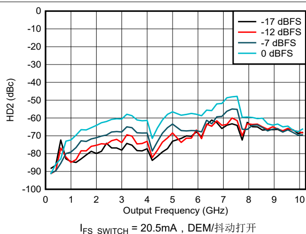
图 6-146. NRZ/RF 模式下 HD2 与频率和数字振幅间的关系
