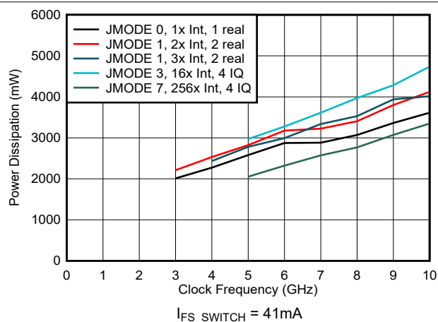
图 6-212. 功率损耗与时钟频率和数字模式间的关系
