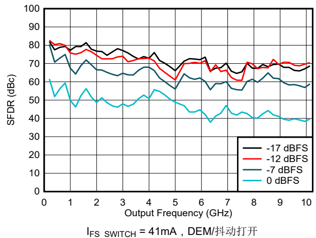
图 6-104. NRZ/RF 模式下 SFDR 与频率和数字振幅间的关系
