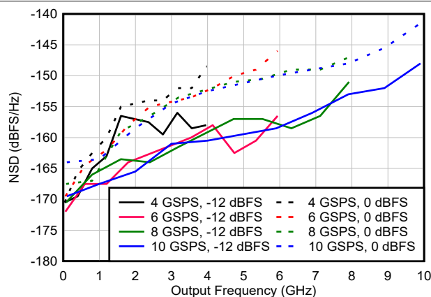
图 6-75. NSD 与输出频率和数字振幅间的关系
