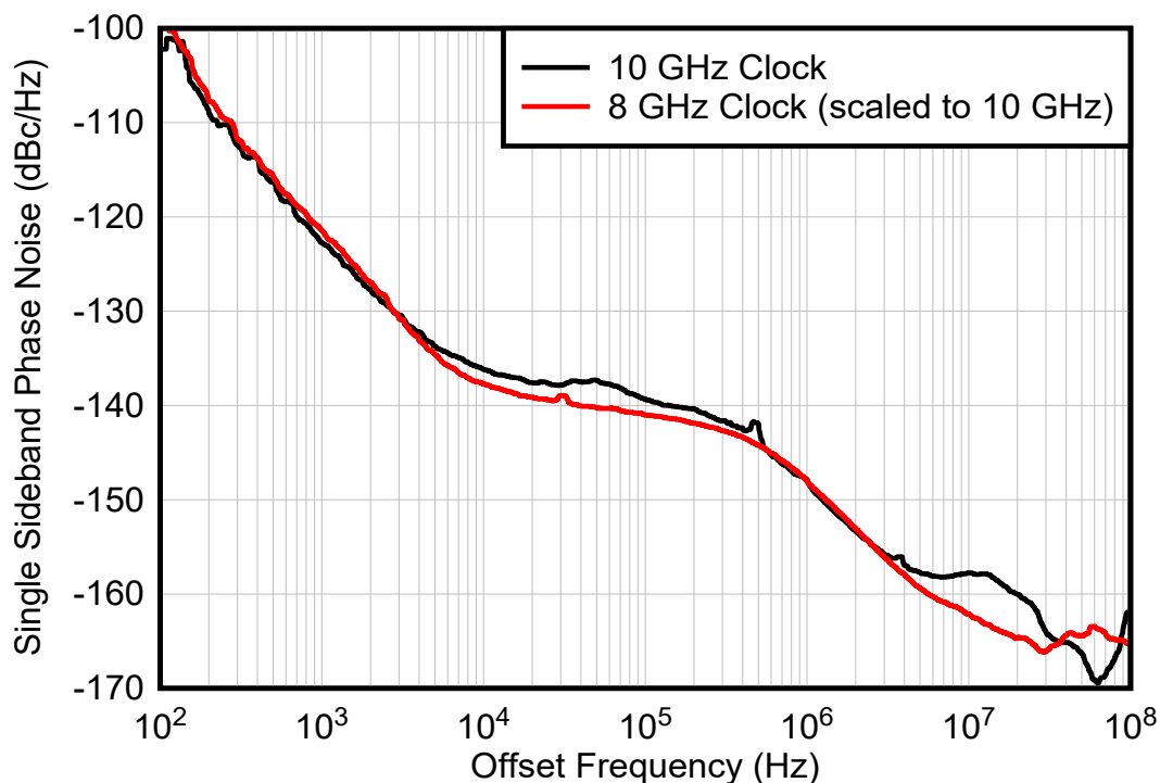
图 8-13. 8GHz 和 10GHz 时钟相位噪声
