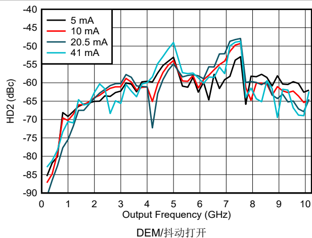
图 6-142. NRZ/RF 模式下 HD2 与频率和输出电流间的关系
