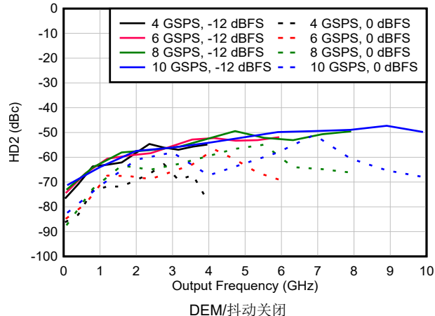
图 6-154. NRZ/RF 模式下 HD2 与频率和采样速率间的关系
