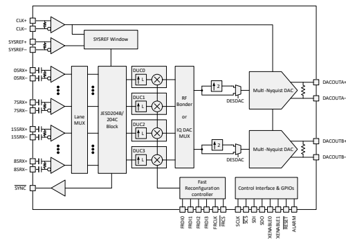
方框图
