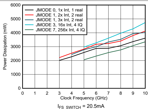
图 6-211. 功率损耗与时钟频率和数字模式间的关系
