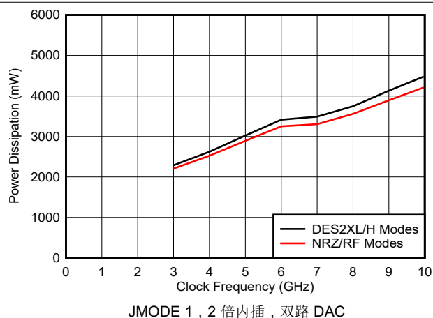
图 6-214. 功率损耗与时钟频率以及 DAC 模式间的关系
