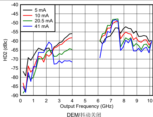
图 6-143. DES2X 模式下 HD2 与频率和输出电流间的关系
