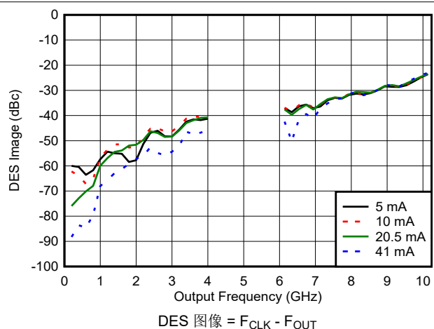
图 6-193. DES2X 模式下 DES 图像与频率和输出电流间的关系
