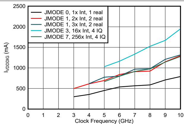
图 6-224. VDDDIG 电流与时钟频率和数字模式间的关系
