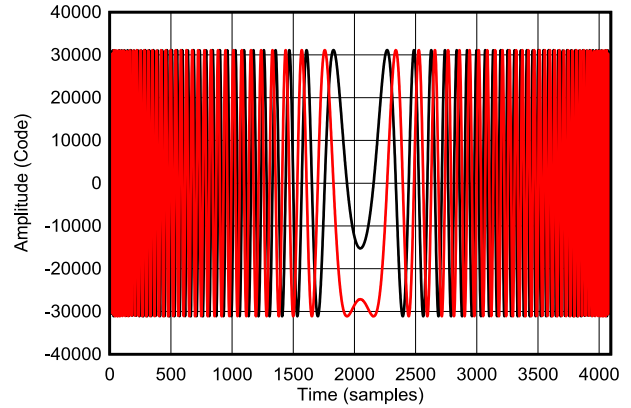
图 8-15. NLFM 线性调频脉冲的复时域 (红色 = 实数, 黑色 = 虚数)
