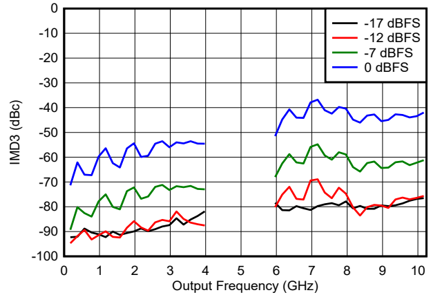
图 6-124. DES2X 模式下 IMD3 与频率和数字振幅间的关系
