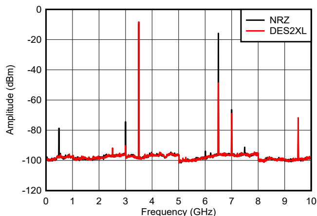
图 8-3. DES2XL 和 NRZ 模式的输出频谱比较
