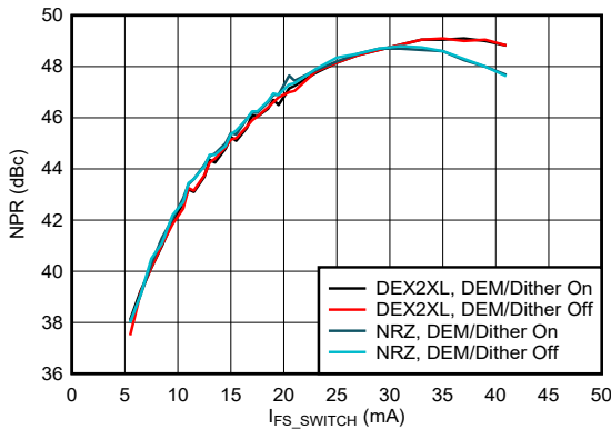
图 6-199. 电源抑制比与输出电流间的关系：第一奈奎斯特区域
