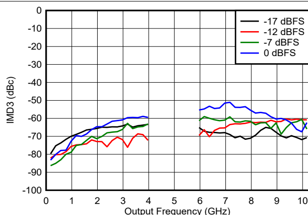
图 6-119. NRZ/RF 模式下 IMD3 与频率和数字振幅间的关系
