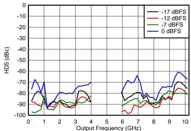
图 6-186. DES2X 模式下 HD5 与频率和数字振幅间的关系
