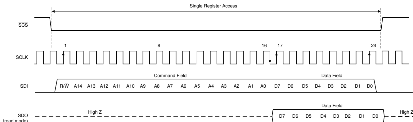
图 7-58. 串行接口协议：单独读取和写入
