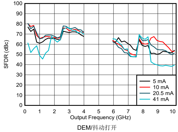
图 6-100. DES2X 模式下 SFDR 与频率和输出电流间的关系
