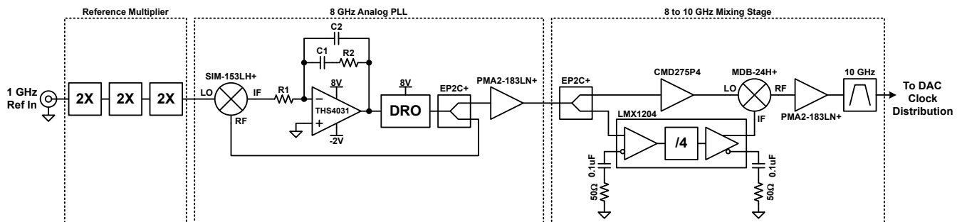
图 8-12. 10GHz 时钟合成器
