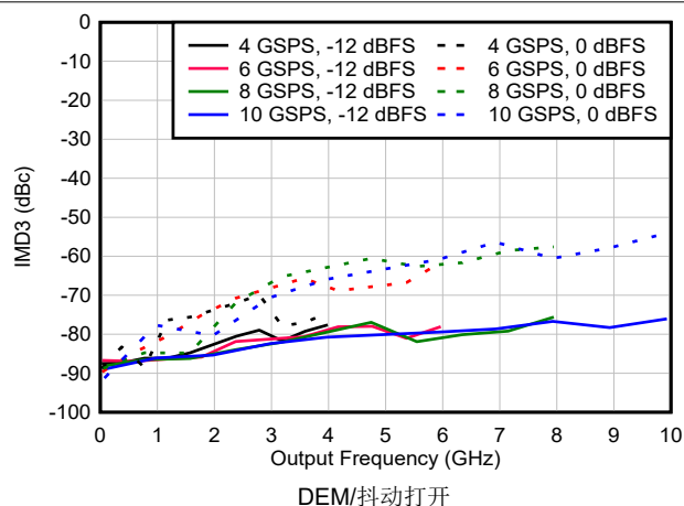
图 6-129. NRZ/RF 模式下 IMD3 与频率和采样速率间的关系
