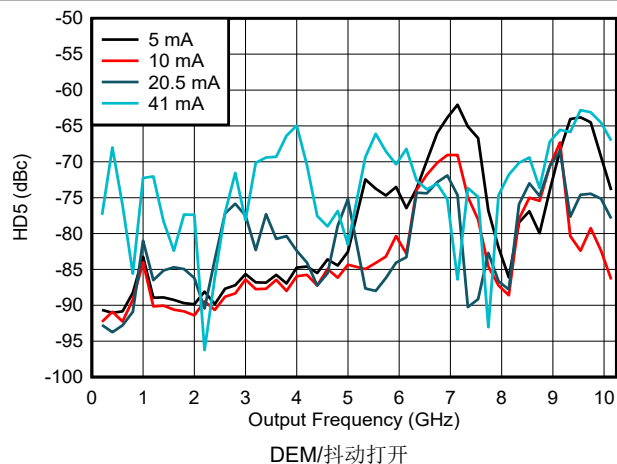
图 6-178. NRZ/RF 模式下 HD5 与频率和输出电流间的关系
