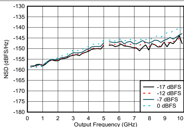
图 6-65. NSD 与输出频率和数字振幅间的关系
