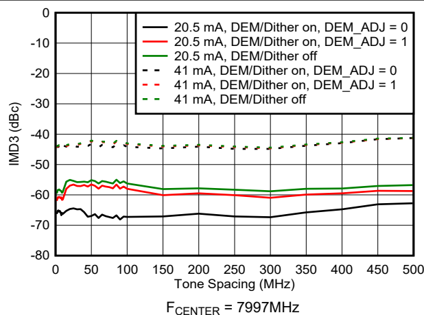
图 6-127. RF 模式下 IMD3 与频率间隔间的关系
