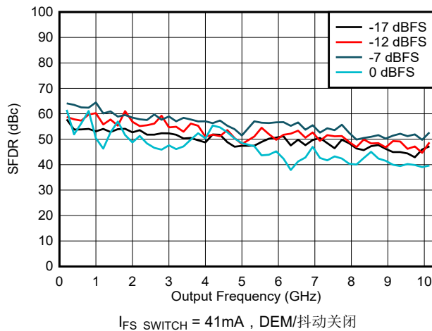
图 6-103. NRZ/RF 模式下 SFDR 与频率和数字振幅间的关系
