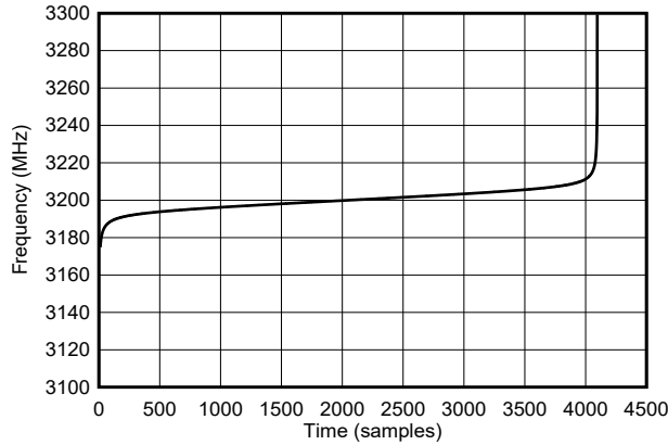
图 8-14. NLFM 频率斜升
