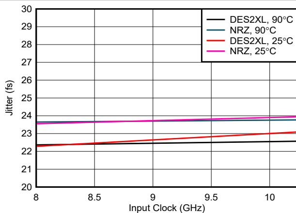
图 6-207. 抖动与输入时钟间的关系
