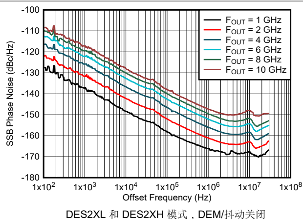
图 6-203. 相位噪声与偏移频率和输出频率间的关系
