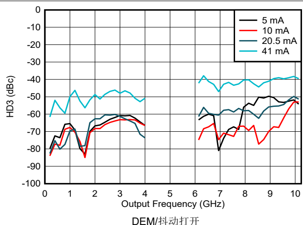
图 6-158. NRZ/RF 模式下 HD3 与频率和输出电流间的关系
