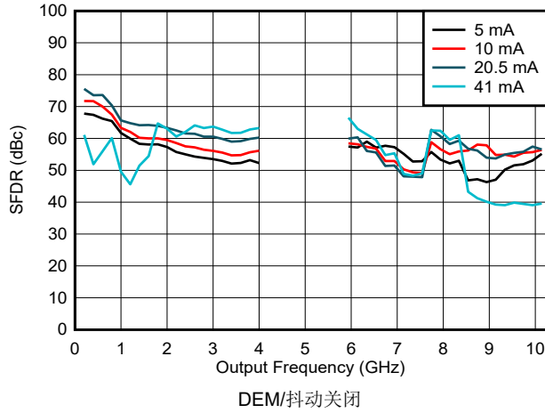
图 6-99. DES2X 模式下 SFDR 与频率和输出电流间的关系
