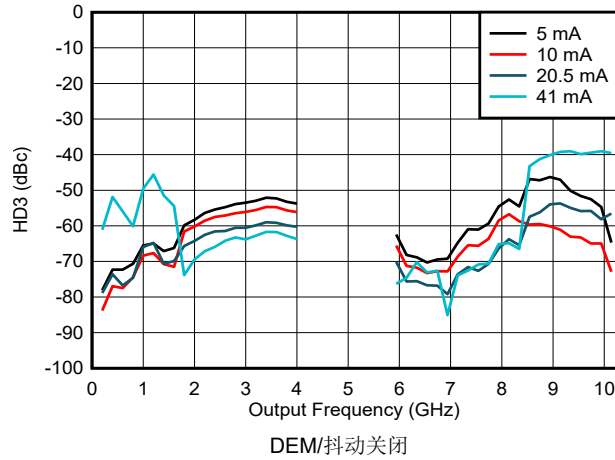
图 6-159. DES2X 模式下 HD3 与频率和输出电流间的关系
