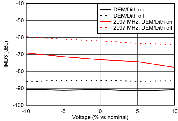
图 6-137. NRZ 模式下 IMD3 与电压间的关系
