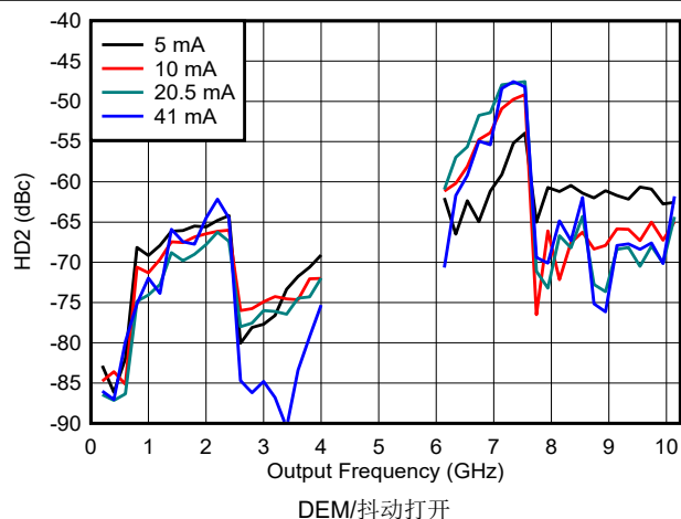
图 6-144. DES2X 模式下 HD2 与频率和输出电流间的关系
