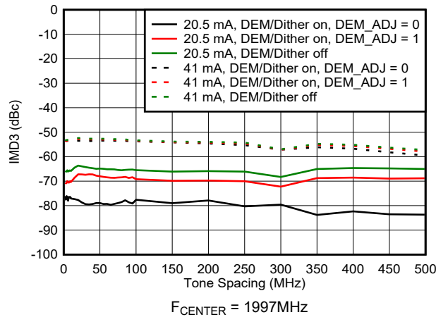
图 6-125. NRZ 模式下 IMD3 与频率间隔间的关系
