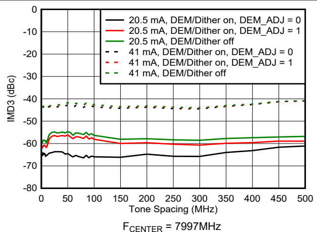
图 6-128. DES2XH 模式下 IMD3 与频率间隔间的关系
