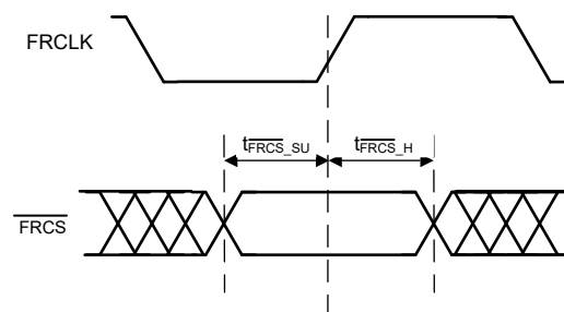
图 6-7. \overline{FRCS} 时序图
