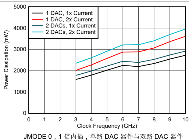
图 6-215. 功率损耗与时钟频率以及 DAC 模式间的关系
