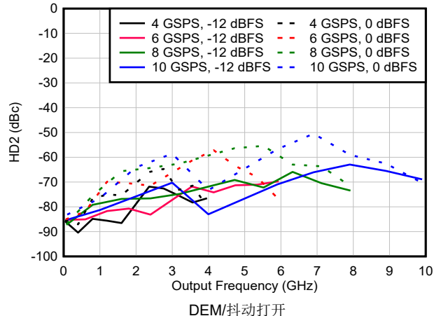
图 6-153. NRZ/RF 模式下 HD2 与频率和采样速率间的关系
