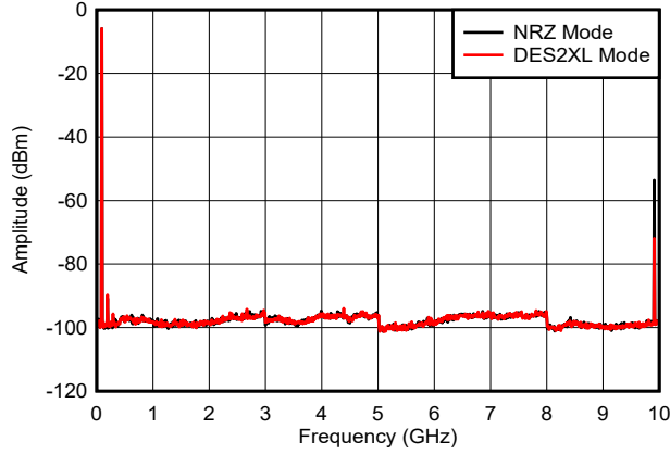
图 6-19. f_{\text{OUT}} = 97\text{ MHz} ， 0\text{ dBFS}
