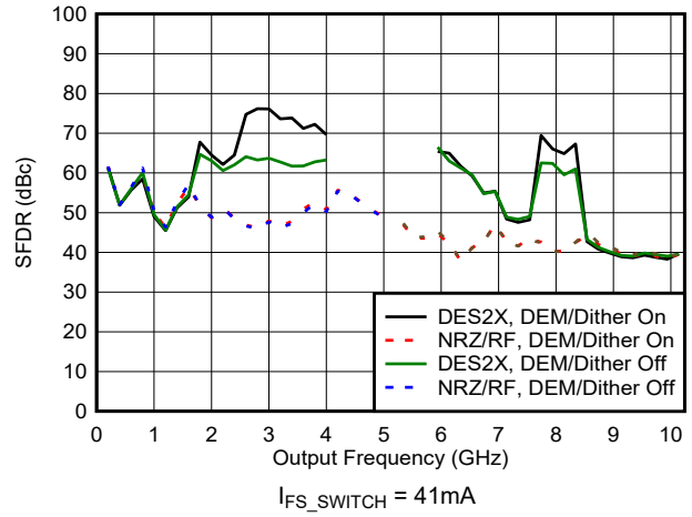
图 6-90. SFDR 与频率和模式间的关系
