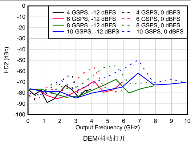
图 6-155. DES2X 模式下 HD2 与频率和采样速率间的关系
