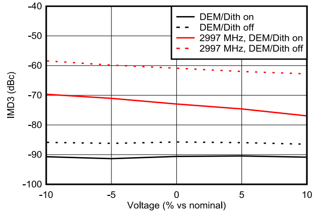
图 6-138. DES2XL 模式下 IMD3 与电压间的关系
