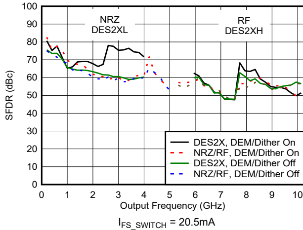
图 6-89. SFDR 与频率和模式间的关系
