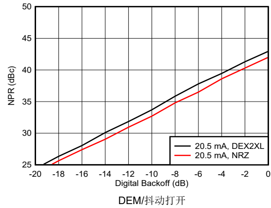
图 6-198. 噪声功率比与数字退避：第二个奈奎斯特区域
