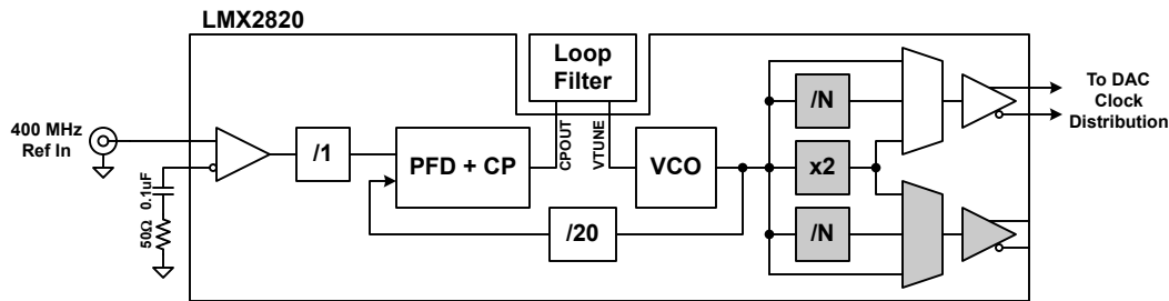
图 8-8. 带内部 VCO 的 LMX2820
