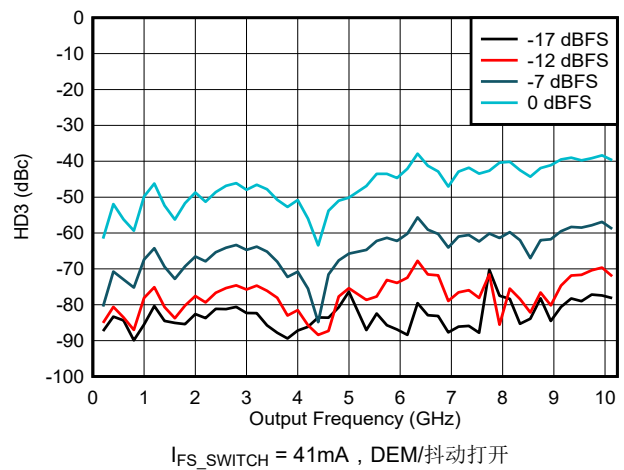
图 6-164. NRZ/RF 模式下 HD3 与频率和数字振幅间的关系
