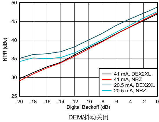
图 6-195. 噪声功率比与数字退避：第一奈奎斯特区域
