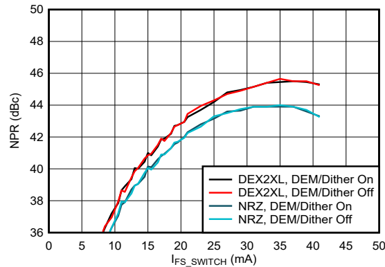
图 6-200. 电源抑制比与输出电流间的关系：第二个奈奎斯特区域
