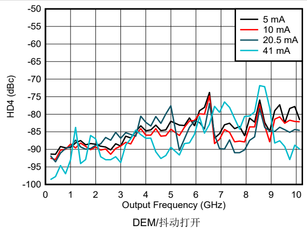
图 6-174. NRZ/RF 模式下 HD4 与频率和输出电流间的关系
