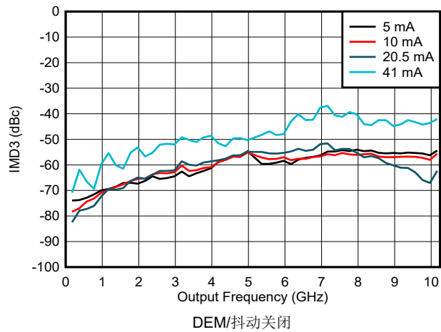
图 6-113. NRZ/RF 模式下 IMD3 与频率和输出电流间的关系
