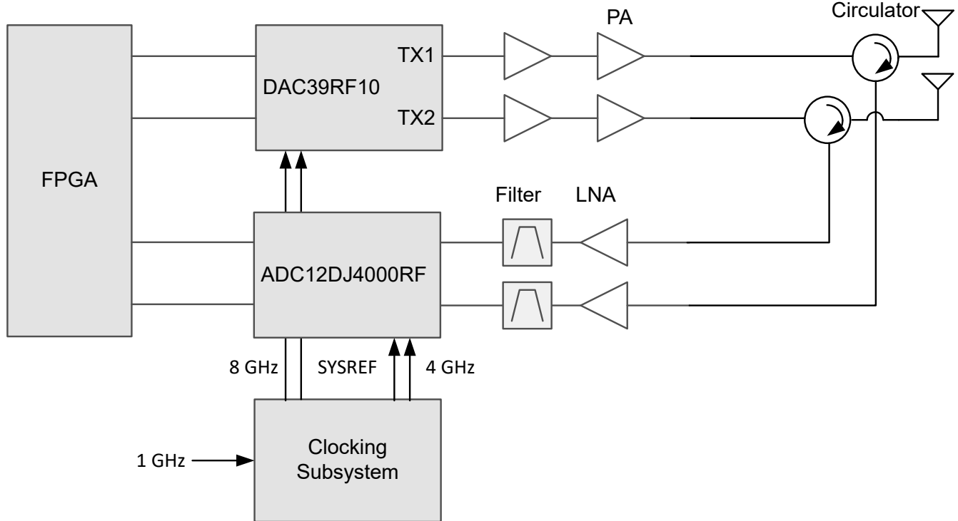
图 8-6. 使用 DAC39RF10 和 ADC12DJ4000RF 的双通道雷达收发器
