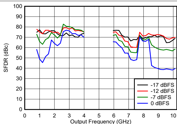
图 6-106. DES2X 模式下 SFDR 与频率和数字振幅间的关系
