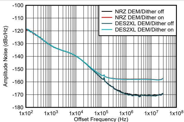
图 6-208. 1GHz 条件下振幅噪声与偏移频率间的关系
