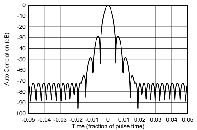
图 8-17. NLFM 线性调频脉冲的自动关联
