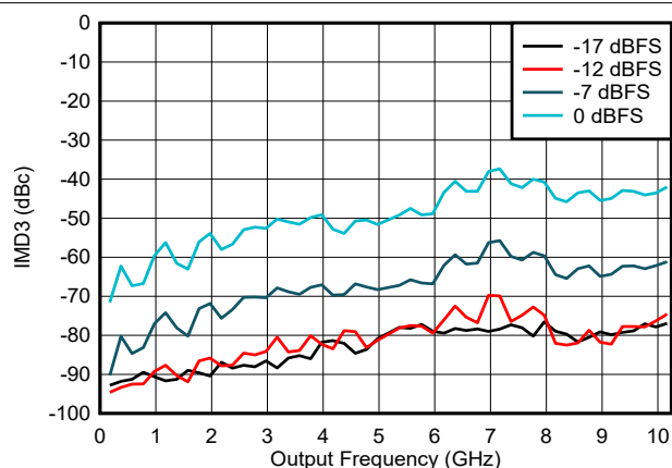
图 6-118. NRZ/RF 模式下 IMD3 与频率和数字振幅间的关系
