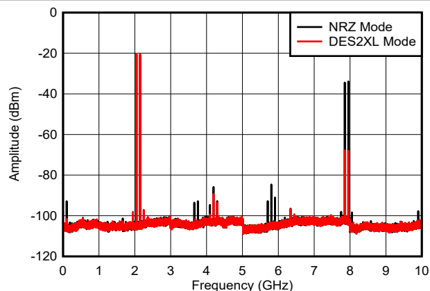
图 6-47. 双音， f_{\text{OUT}} = 2097\text{ MHz} ，-6dBFS
