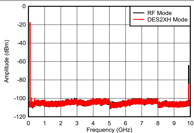
图 6-37. 双音， f_{\text{OUT}} = 97\text{ MHz} ， 0\text{ dBFS} ( 0 - f_{\text{CLK}} )
