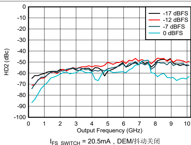
图 6-145. NRZ/RF 模式下 HD2 与频率和数字振幅间的关系
