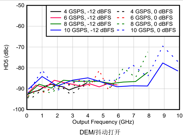
图 6-189. NRZ/RF 模式下 HD5 与频率和采样速率间的关系
