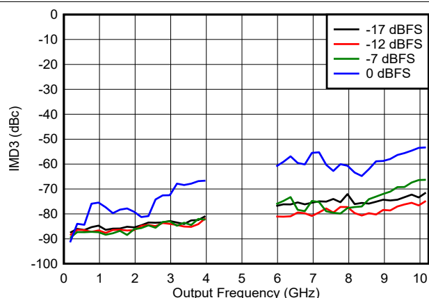
图 6-120. NRZ/RF 模式下 IMD3 与频率和数字振幅间的关系
