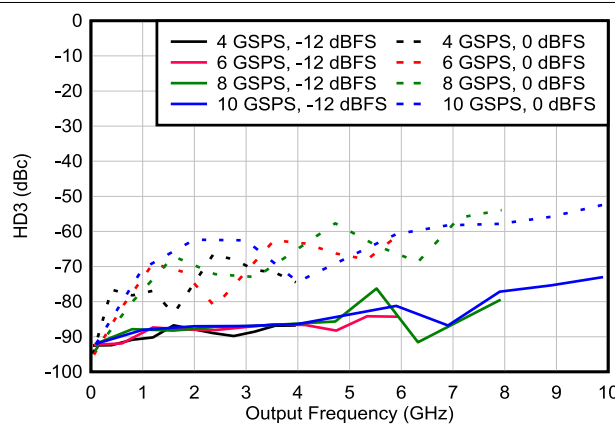
图 6-167. DES2X 模式下 HD3 与频率和数字振幅间的关系
