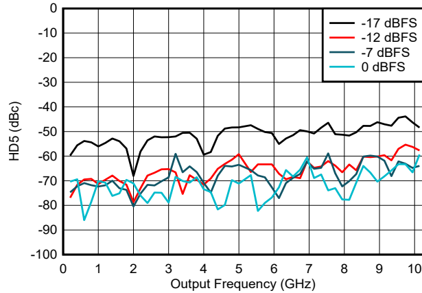
图 6-183. NRZ/RF 模式下 HD5 与频率和数字振幅间的关系
