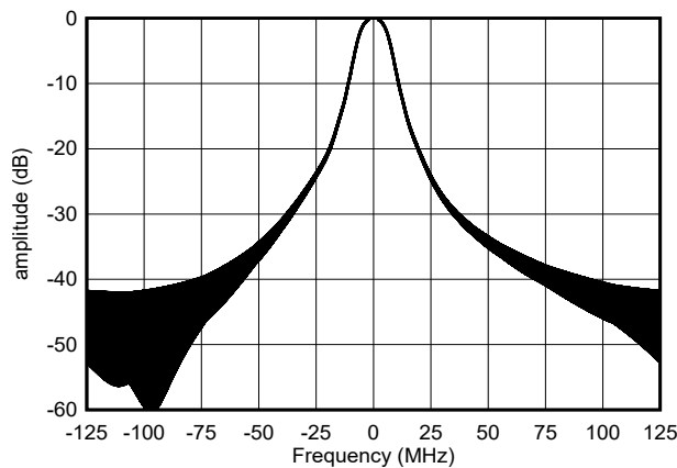
图 8-16. NLFM 线性调频脉冲的数字频谱
