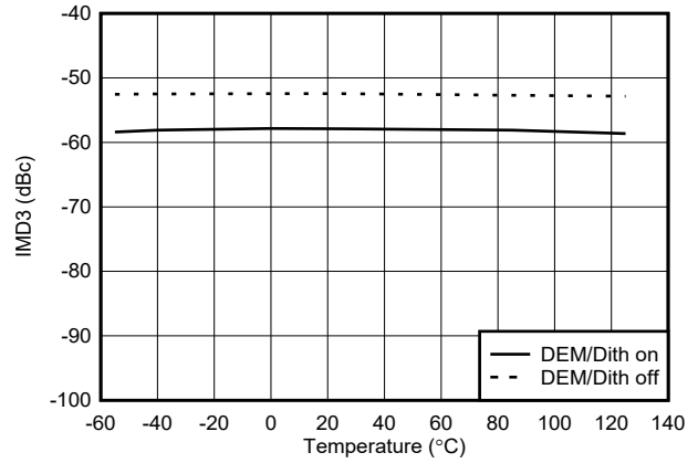
图 6-136. 7247MHz DES2XH 模式下 IMD3 与温度间的关系
