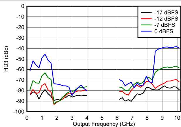
图 6-166. DES2X 模式下 HD3 与频率和数字振幅间的关系
