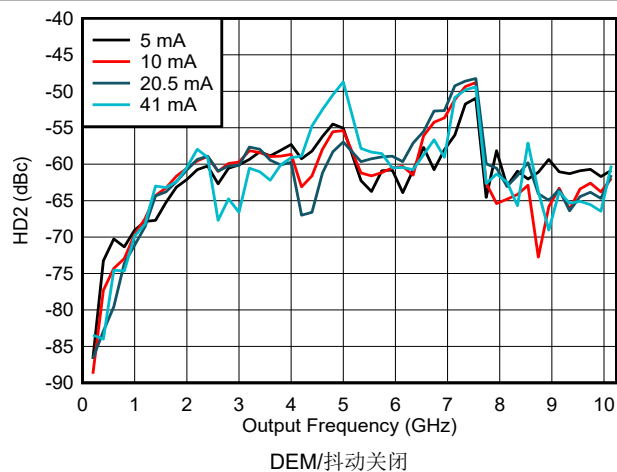
图 6-141. NRZ/RF 模式下 HD2 与频率和输出电流间的关系
