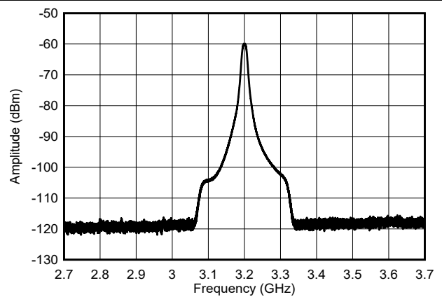
图 8-19. 1GHz 频率下的 NLFM 线性调频脉冲输出频谱
