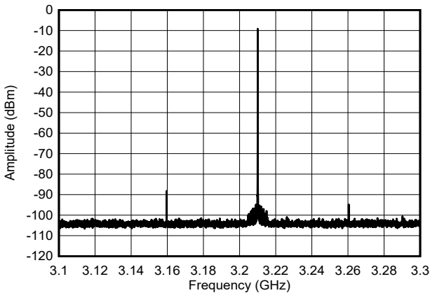
图 8-20. f_{OUT} = 3.211\text{GHz} 时的带内单音频谱
