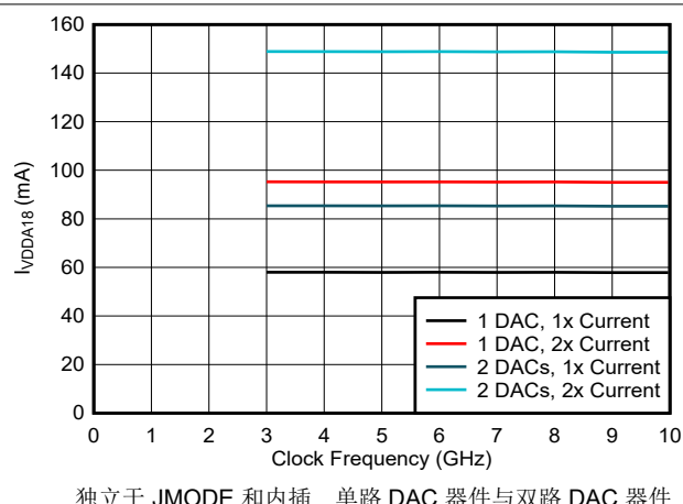
图 6-216. VDDA18 电流与时钟频率和 DAC 模式间的关系
