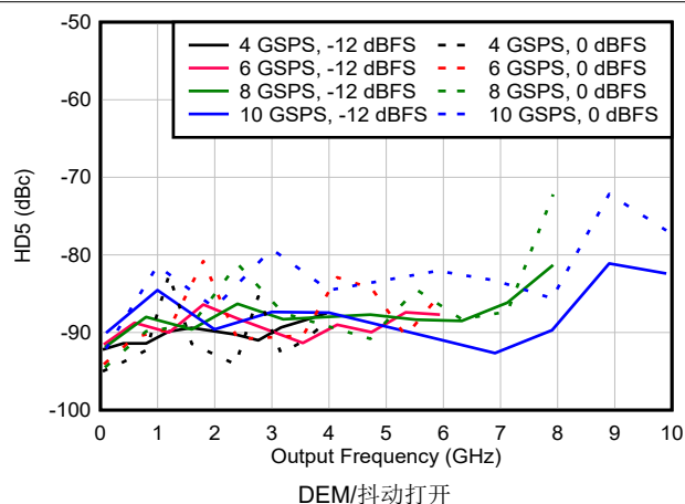
图 6-191. DES2X 模式下 HD5 与频率和采样速率间的关系
