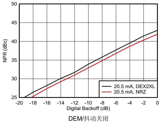
图 6-197. 噪声功率比与数字退避：第二个奈奎斯特区域
