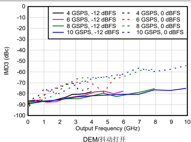
图 6-131. DES2X 模式下 IMD3 与频率和采样速率间的关系
