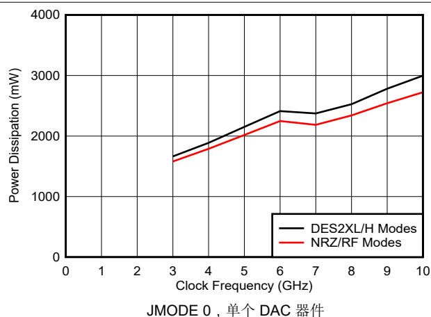
图 6-213. 功率损耗与时钟频率以及 DAC 模式间的关系
