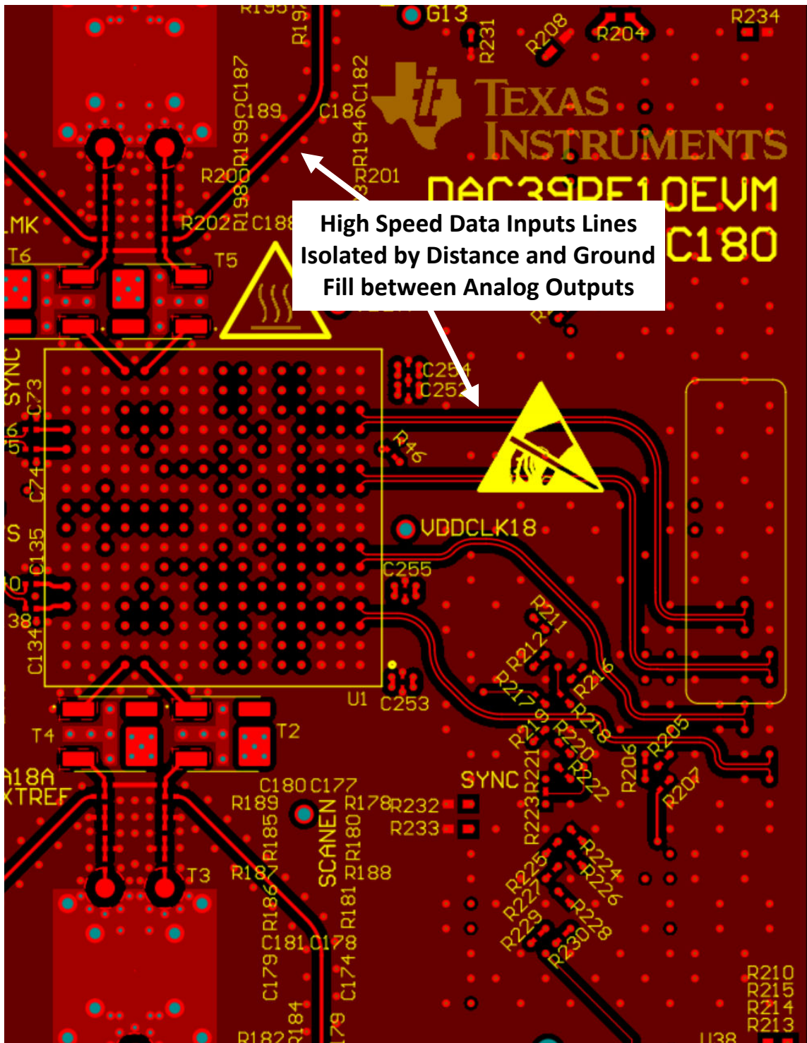
图 8-29. 具有地线填充隔离的串行器/解串器顶层布线
