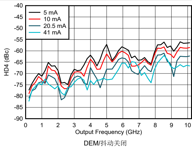
图 6-173. NRZ/RF 模式下 HD4 与频率和输出电流间的关系
