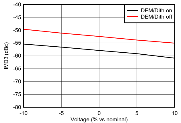
图 6-140. 7247MHz DES2XH 模式下 IMD3 与电压间的关系
