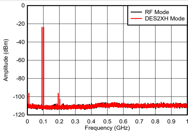
图 6-40. 双音， f_{\text{OUT}} = 97\text{ MHz} ， -6\text{ dBFS} ( 0\text{ GHz} 至 1\text{ GHz} )
