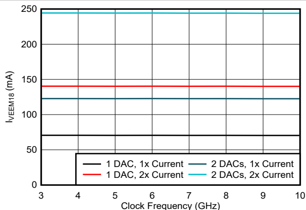
图 6-218. VEEM18 电流与时钟频率和 DAC 模式间的关系
