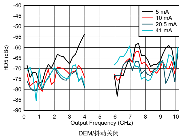
图 6-179. DES2X 模式下 HD5 与频率和输出电流间的关系
