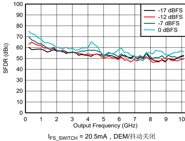
图 6-101. NRZ/RF 模式下 SFDR 与频率和数字振幅间的关系
