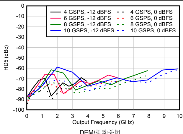
图 6-192. DES2X 模式下 HD5 与频率和采样速率间的关系
