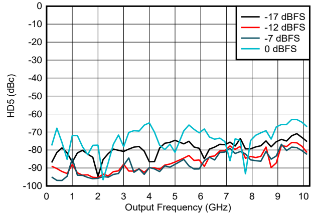
图 6-184. NRZ/RF 模式下 HD5 与频率和数字振幅间的关系
