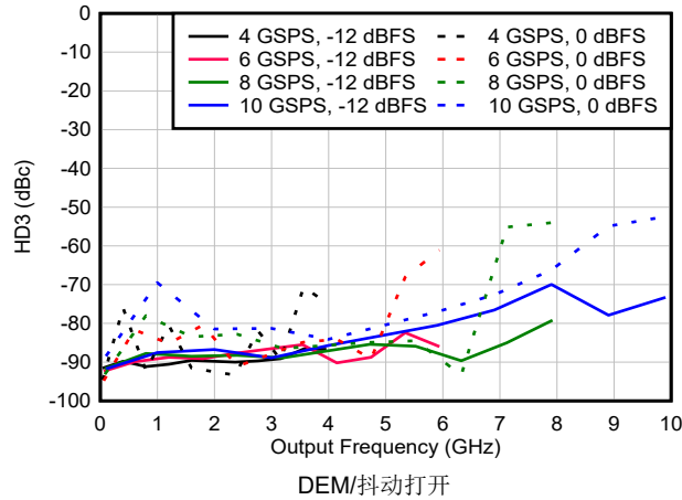
图 6-171. DES2X 模式下 HD3 与频率和采样速率间的关系
