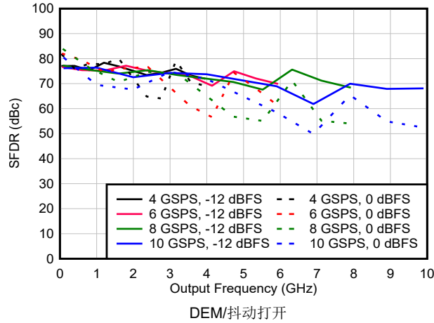
图 6-111. DES2X 模式下 SFDR 与频率和采样速率间的关系
