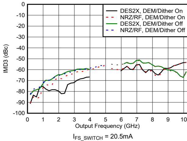
图 6-91. IMD3 与频率和模式间的关系
