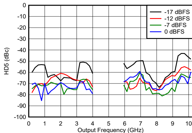
图 6-185. DES2X 模式下 HD5 与频率和数字振幅间的关系
