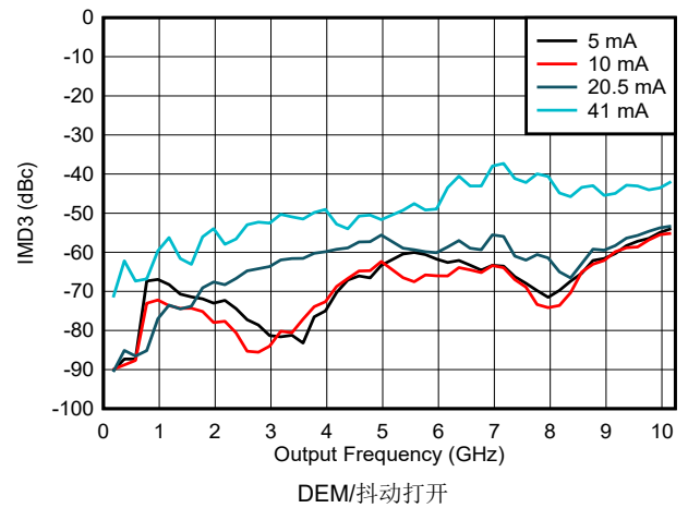
图 6-114. NRZ/RF 模式下 IMD3 与频率和输出电流间的关系
