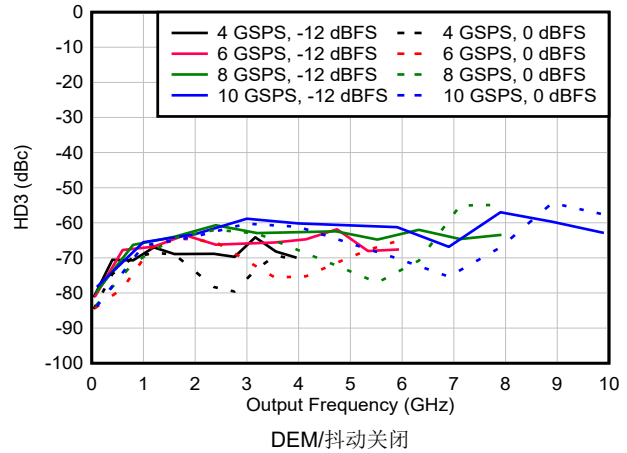
图 6-172. DES2X 模式下 HD3 与频率和采样速率间的关系
