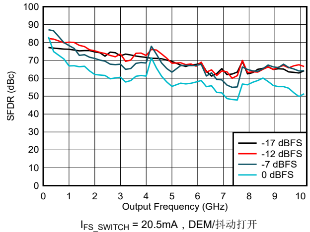
图 6-102. NRZ/RF 模式下 SFDR 与频率和数字振幅间的关系
