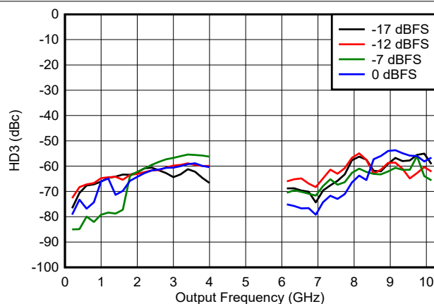
图 6-165. DES2X 模式下 HD3 与频率和数字振幅间的关系
