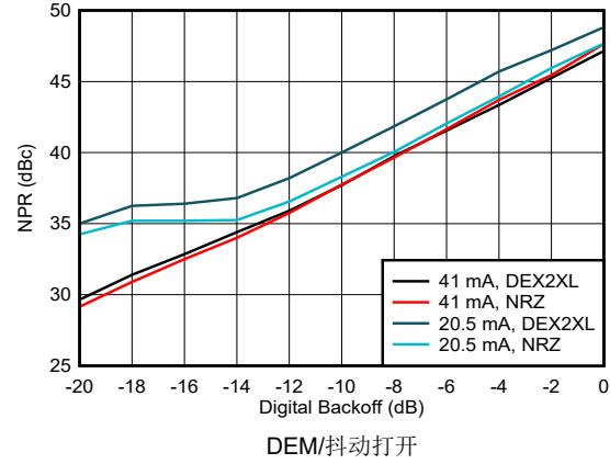
图 6-196. 噪声功率比与数字退避：第一奈奎斯特区域
