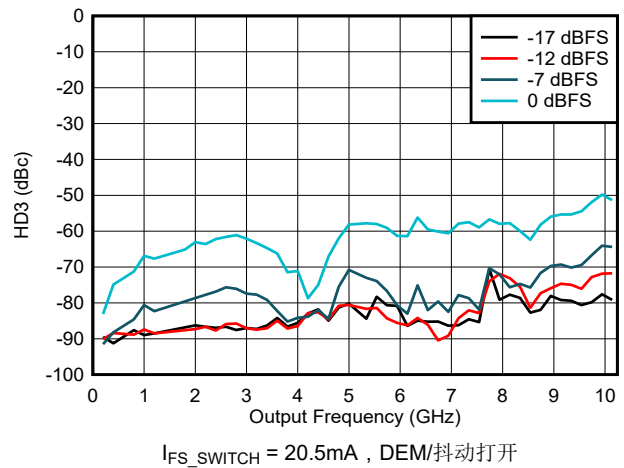
图 6-162. NRZ/RF 模式下 HD3 与频率和数字振幅间的关系
