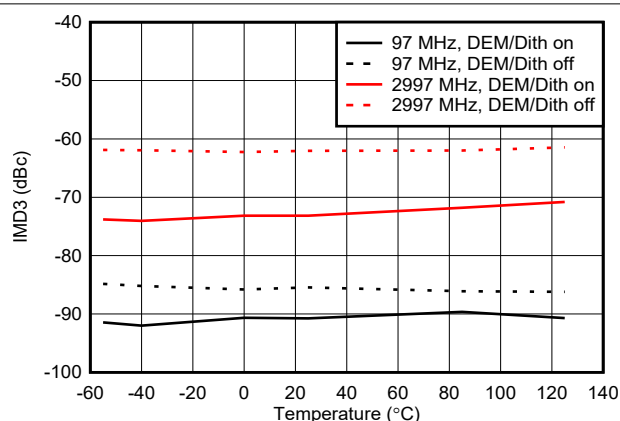
图 6-133. NRZ 模式下 IMD3 与温度间的关系
