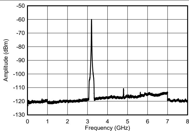
图 8-18. 0GHz 至 8GHz 频率下的 NLFM 线性调频脉冲输出频谱
