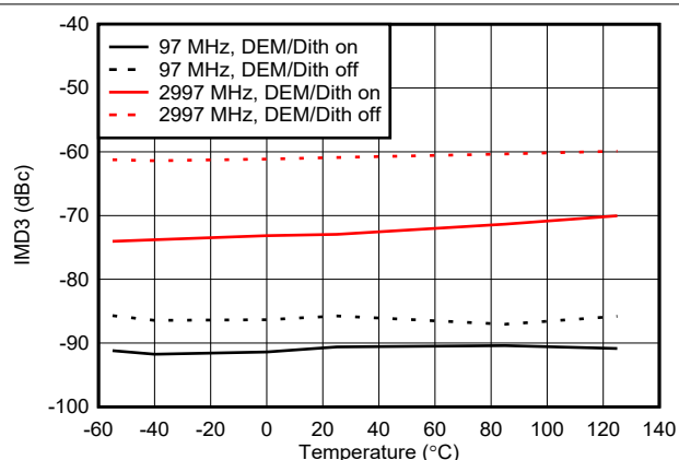
图 6-134. DES2XL 模式下 IMD3 与温度间的关系
