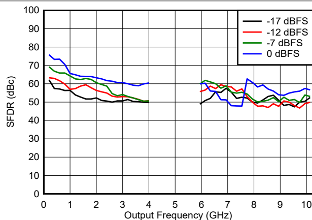
图 6-105. DES2X 模式下 SFDR 与频率和数字振幅间的关系
