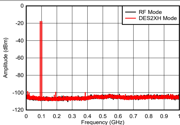
图 6-38. 双音， f_{\text{OUT}} = 97\text{ MHz} ， 0\text{ dBFS} ( 0\text{ GHz} 至 1\text{ GHz} )
