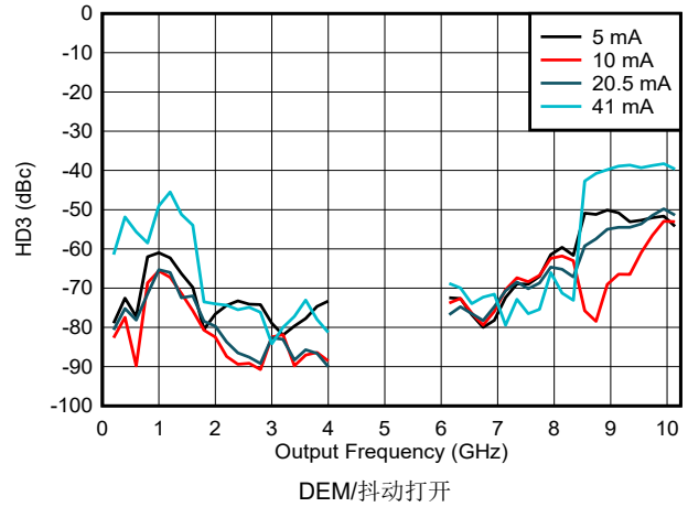
图 6-160. DES2X 模式下 HD3 与频率和输出电流间的关系
