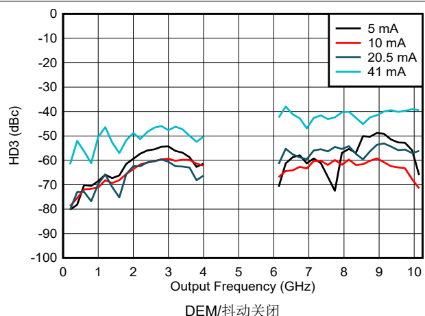
图 6-157. NRZ/RF 模式下 HD3 与频率和输出电流间的关系
