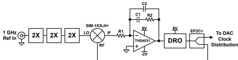
图 8-10. 分立式模拟 PLL
