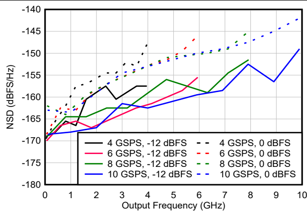
图 6-77. NSD 与输出频率和采样速率间的关系
