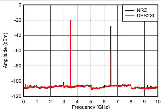
图 6-28. f_{\text{OUT}} = 3497\text{ MHz} ，0dBFS
