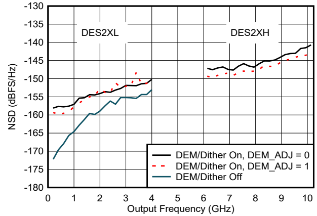
图 6-59. NSD 与输出频率和 DEM/抖动模式间的关系
