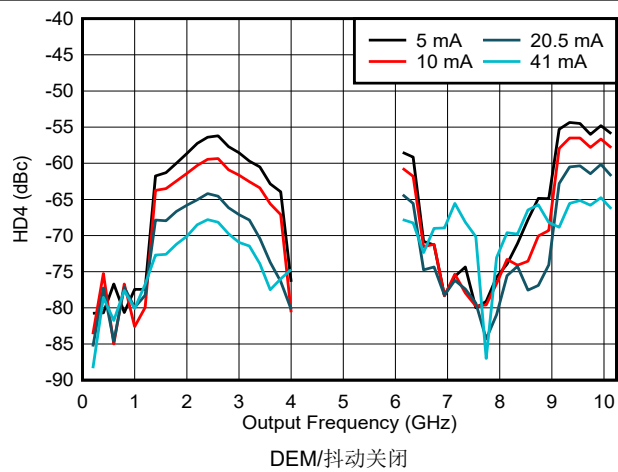
图 6-175. DES2X 模式下 HD4 与频率和输出电流间的关系
