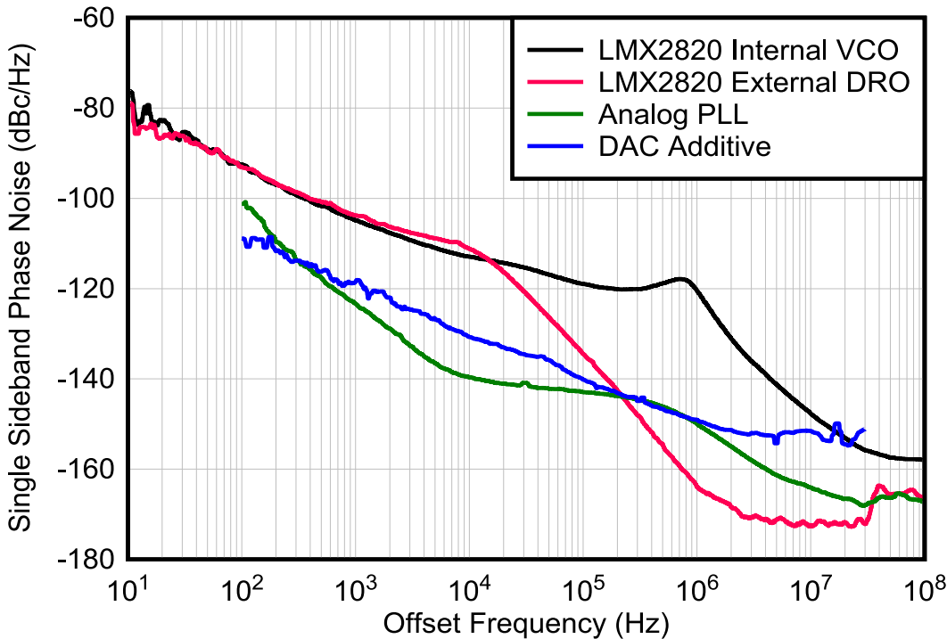
图 8-7. 具有器件附加相位噪声的 DAC 时钟示例的相位噪声
