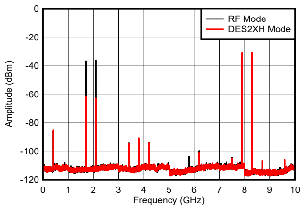
图 6-55. 双音， f_{\text{OUT}} = 8097\text{ MHz} ，0dBFS
