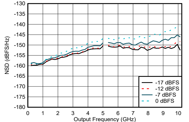
图 6-69. NSD 与输出频率和数字振幅间的关系
