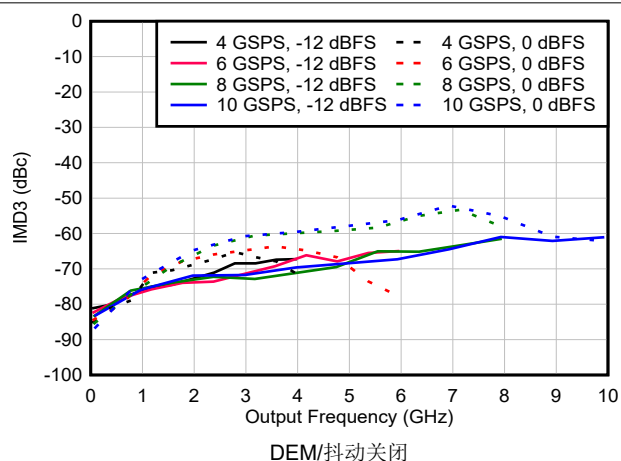
图 6-132. DES2X 模式下 IMD3 与频率和采样速率间的关系
