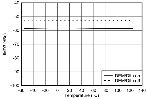
图 6-135. 7247MHz RF 模式下 IMD3 与温度间的关系
