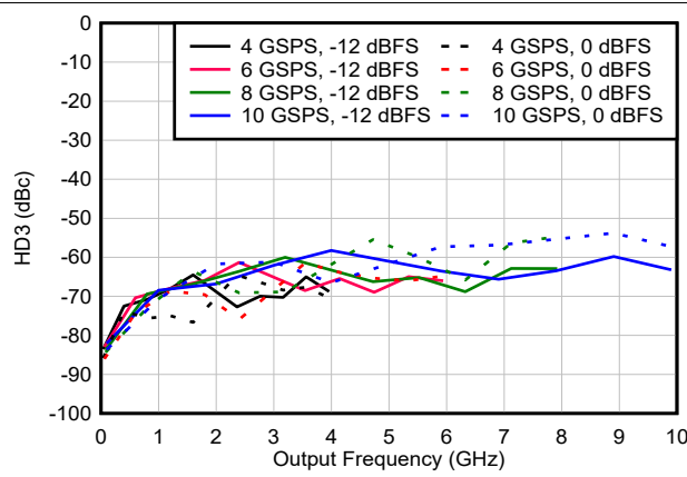
图 6-168. DES2X 模式下 HD3 与频率和数字振幅间的关系
