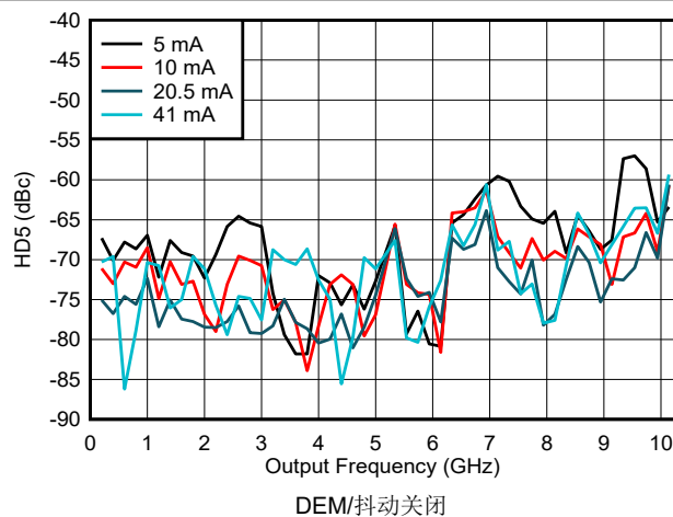
图 6-177. NRZ/RF 模式下 HD5 与频率和输出电流间的关系
