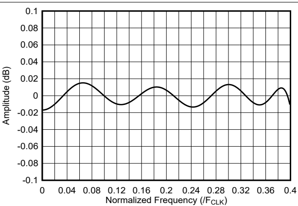
图 7-49. DES 内插器频率响应 (通带)
