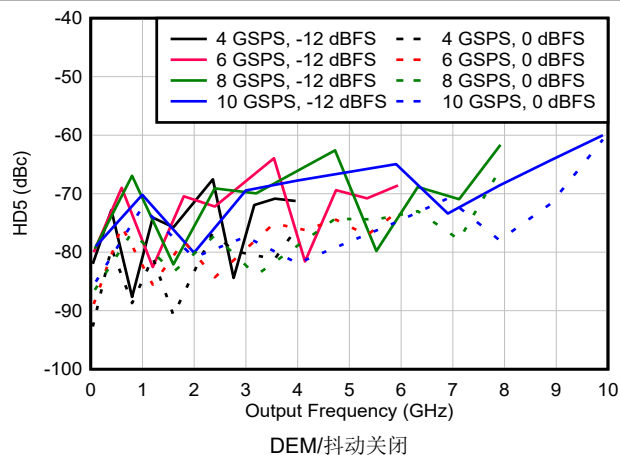
图 6-190. NRZ/RF 模式下 HD5 与频率和采样速率间的关系
