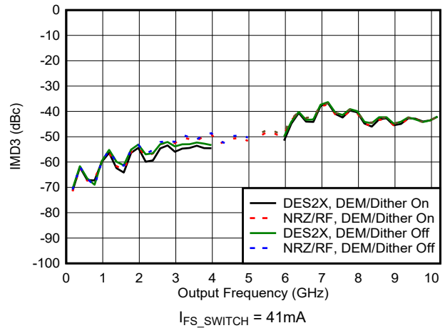
图 6-92. IMD3 与频率和模式间的关系
