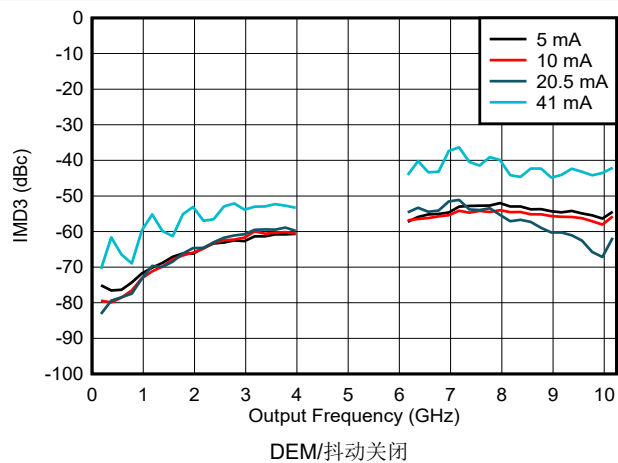
图 6-115. DES2X 模式下 IMD3 与频率和输出电流间的关系
