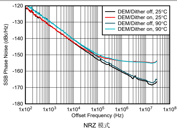
图 6-204. 1GHz 条件下相位噪声与偏移频率间的关系
