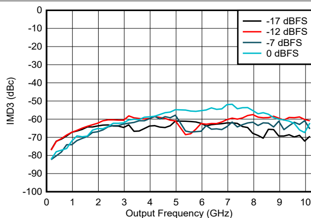
图 6-117. NRZ/RF 模式下 IMD3 与频率和数字振幅间的关系
