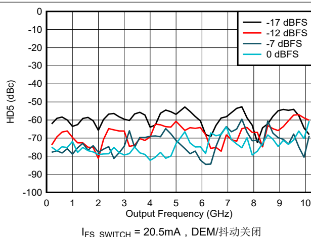
图 6-181. NRZ/RF 模式下 HD5 与频率和数字振幅间的关系
