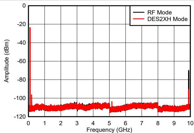
图 6-39. 双音， f_{\text{OUT}} = 97\text{ MHz} ， -6\text{ dBFS} ( 0 - f_{\text{CLK}} )
