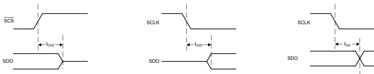
图 6-3. SPI 数据输出时序图
