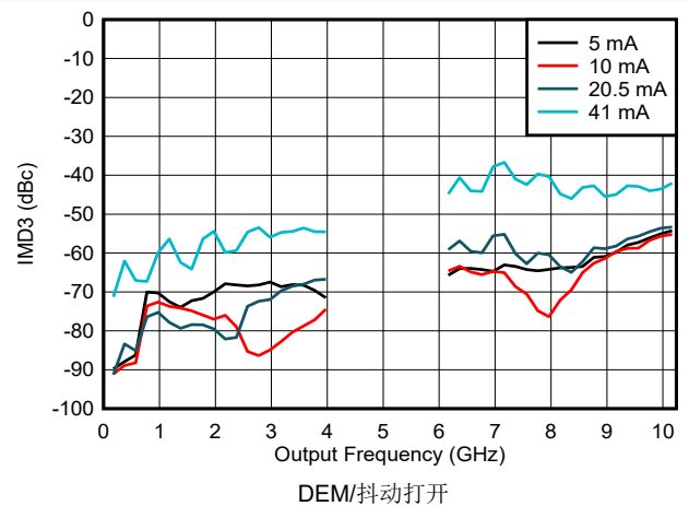
图 6-116. DES2X 模式下 IMD3 与频率和输出电流间的关系
