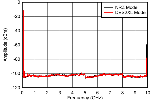
图 6-20. f_{\text{OUT}} = 97\text{ MHz} ， -6\text{ dBFS}
