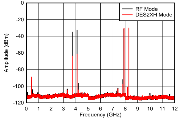
图 6-52. 双音， f_{\text{OUT}} = 8097\text{MHz} ， 0\text{dBFS}
