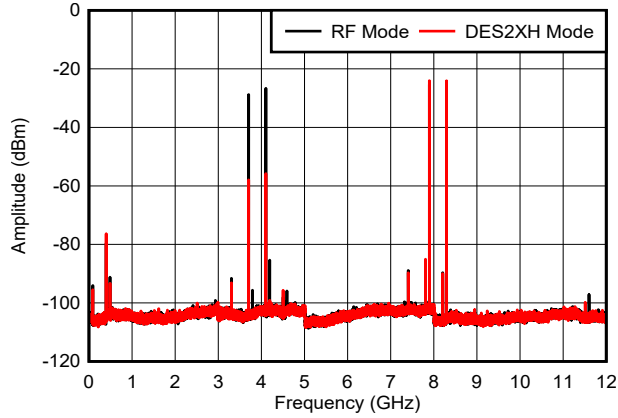
图 6-51. 双音， f_{\text{OUT}} = 3497\text{MHz} ， -12\text{dBFS}
