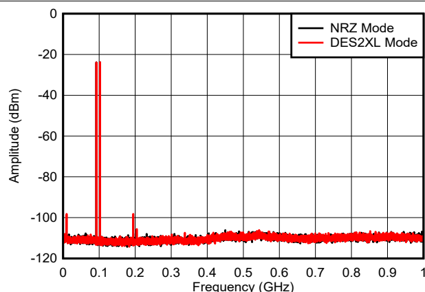
图 6-40. 双音， f_{\text{OUT}} = 97\text{MHz} ，-6dBFS (0GHz 至 1GHz)
