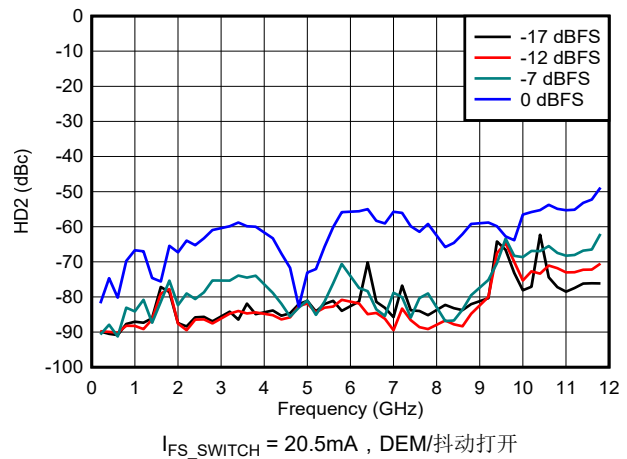
图 6-155. NRZ/RF 模式下 HD2 与频率和数字振幅间的关系
