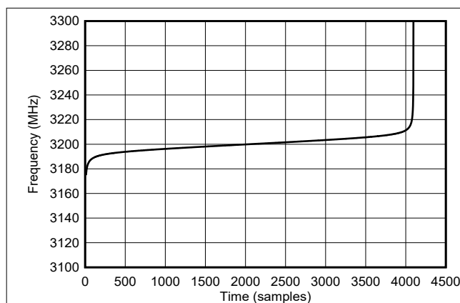
图 8-13. NLFM 频率斜升
