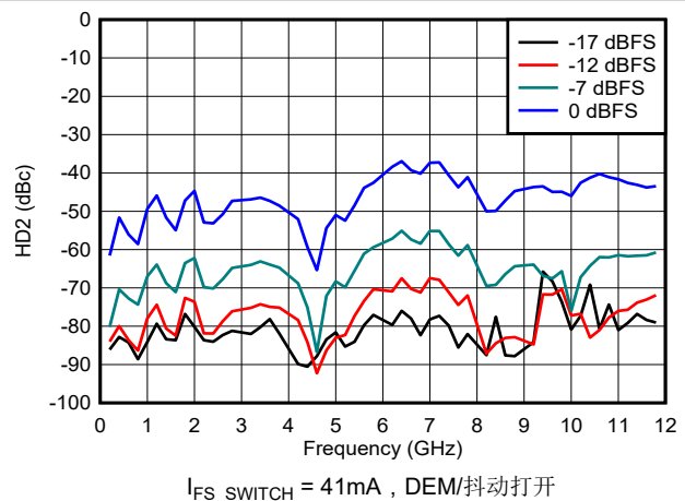
图 6-157. NRZ/RF 模式下 HD2 与频率和数字振幅间的关系
