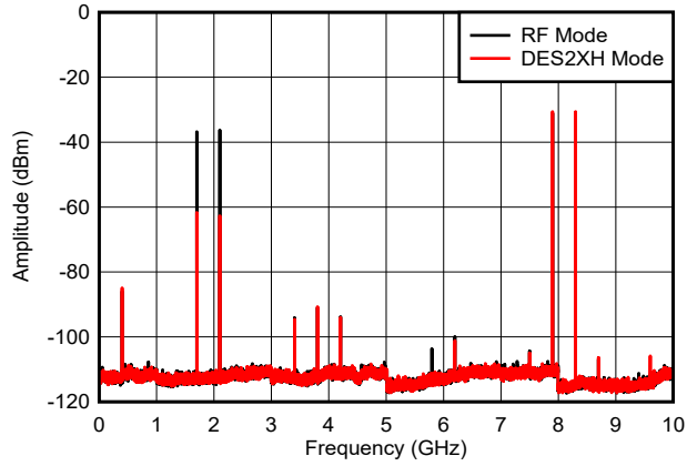
图 6-57. 双音， f_{\text{OUT}} = 7997\text{MHz} ， -12\text{dBFS}
