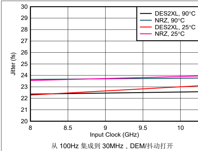
图 6-222. 抖动与输入时钟间的关系
