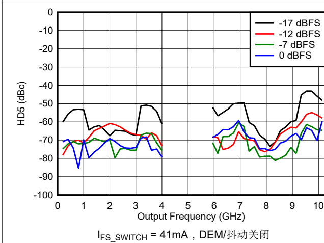
图 6-202. DES2X 模式下 HD5 与频率和数字振幅间的关系
