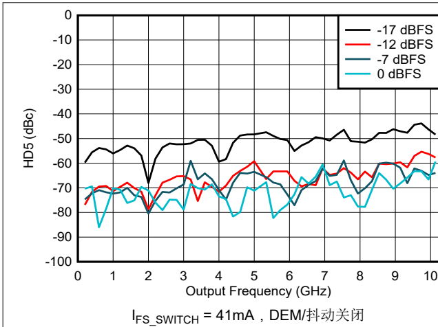
图 6-198. NRZ/RF 模式下 HD5 与频率和数字振幅间的关系
