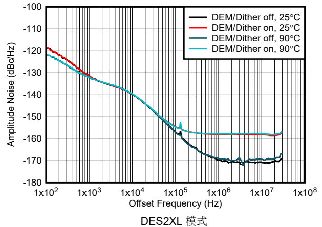
图 6-225. 1GHz 条件下振幅噪声与偏移频率和温度间的关系
