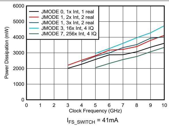
图 6-90. 功率损耗与时钟频率和数字模式间的关系
