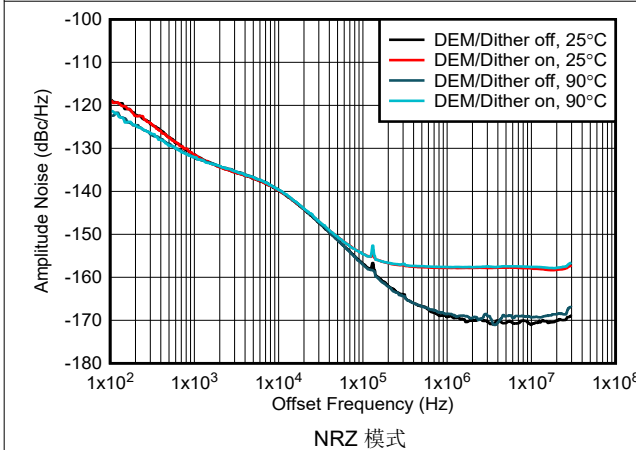
图 6-224. 1GHz 条件下振幅噪声与偏移频率和温度间的关系
