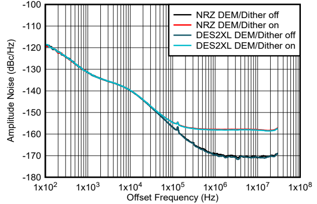
图 6-223. 1GHz 条件下振幅噪声与偏移频率间的关系
