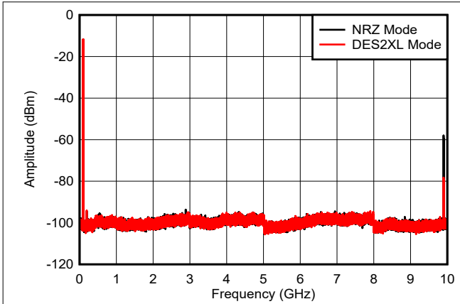
图 6-37. 双音， f_{\text{OUT}} = 97\text{MHz} ，0dBFS (0 - f_{\text{CLK}} )
