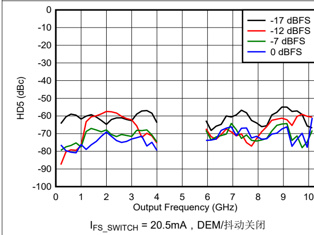
图 6-200. DES2X 模式下 HD5 与频率和数字振幅间的关系
