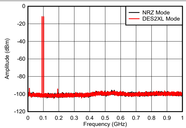
图 6-38. 双音， f_{\text{OUT}} = 97\text{MHz} ，0dBFS (0GHz 至 1GHz)
