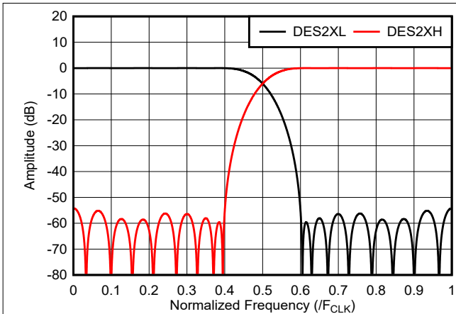
图 7-48. DES 内插器频率响应
