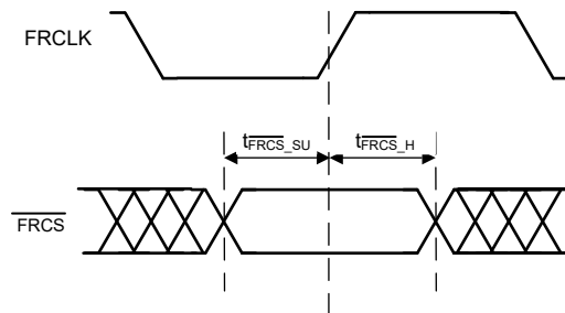
图 6-7. \overline{FRCS} 时序图
