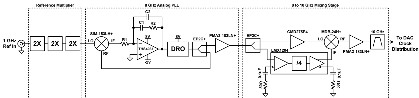
图 8-12. 10GHz 时钟合成器
