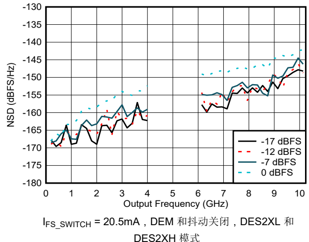
图 6-71. NSD 与输出频率和数字振幅间的关系
