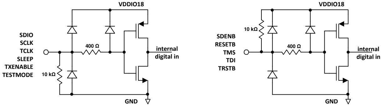
图 7-26. CMOS 数字等效输入
