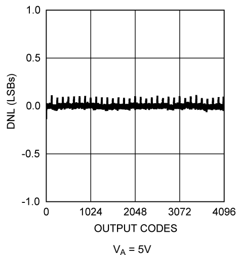
图 5-3. DNL 与输出代码间的关系
