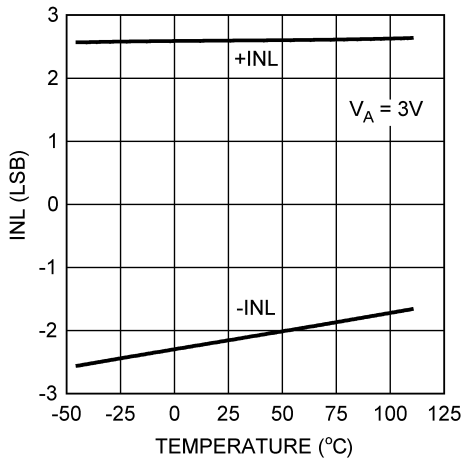
图 5-17. 3V INL 与温度间的关系
