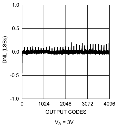
图 5-2. DNL 与输出代码间的关系
