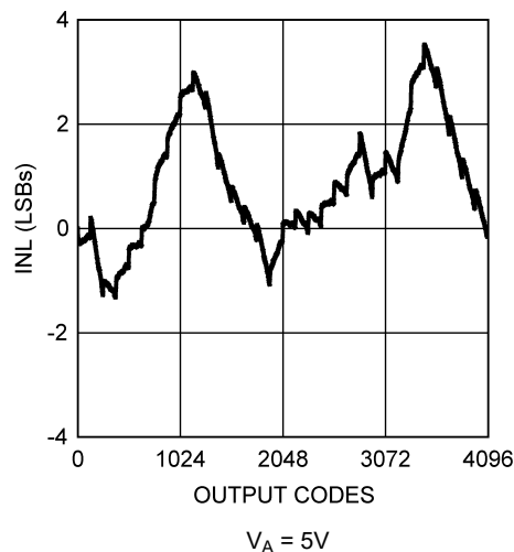
图 5-5. INL 与输出代码间的关系
