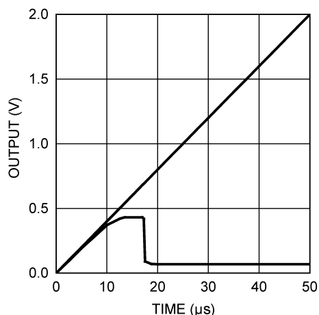
图 5-28. 上电复位
