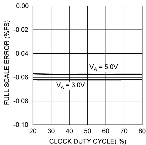
图 5-23. 满量程误差与时钟占空比间的关系
