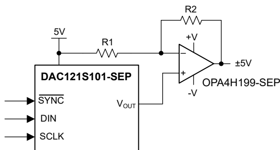
图 7-1. 双极运行
