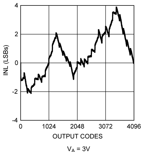
图 5-4. INL 与输出代码间的关系
