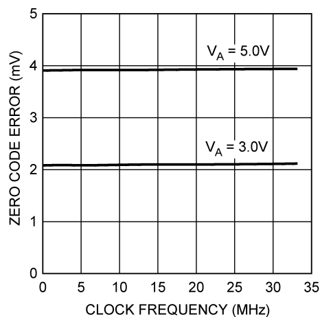
图 5-19. 零代码误差与时钟频率间的关系
