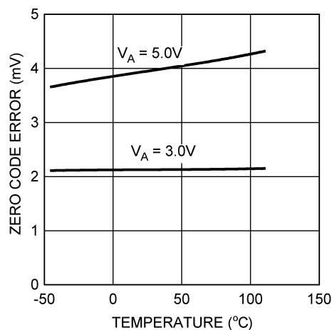
图 5-21. 零代码误差与温度间的关系
