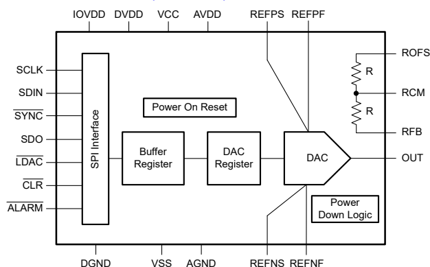
功能方框图
