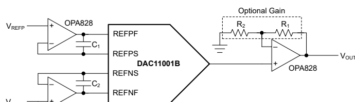
任意波形发生电路
