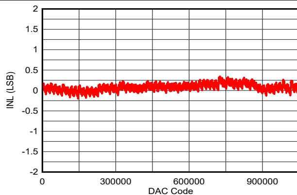
图 8-5. INL at \pm 5\text{-V} Output
