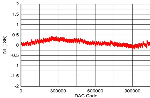
图 8-2. INL at \pm 10 -V Output
