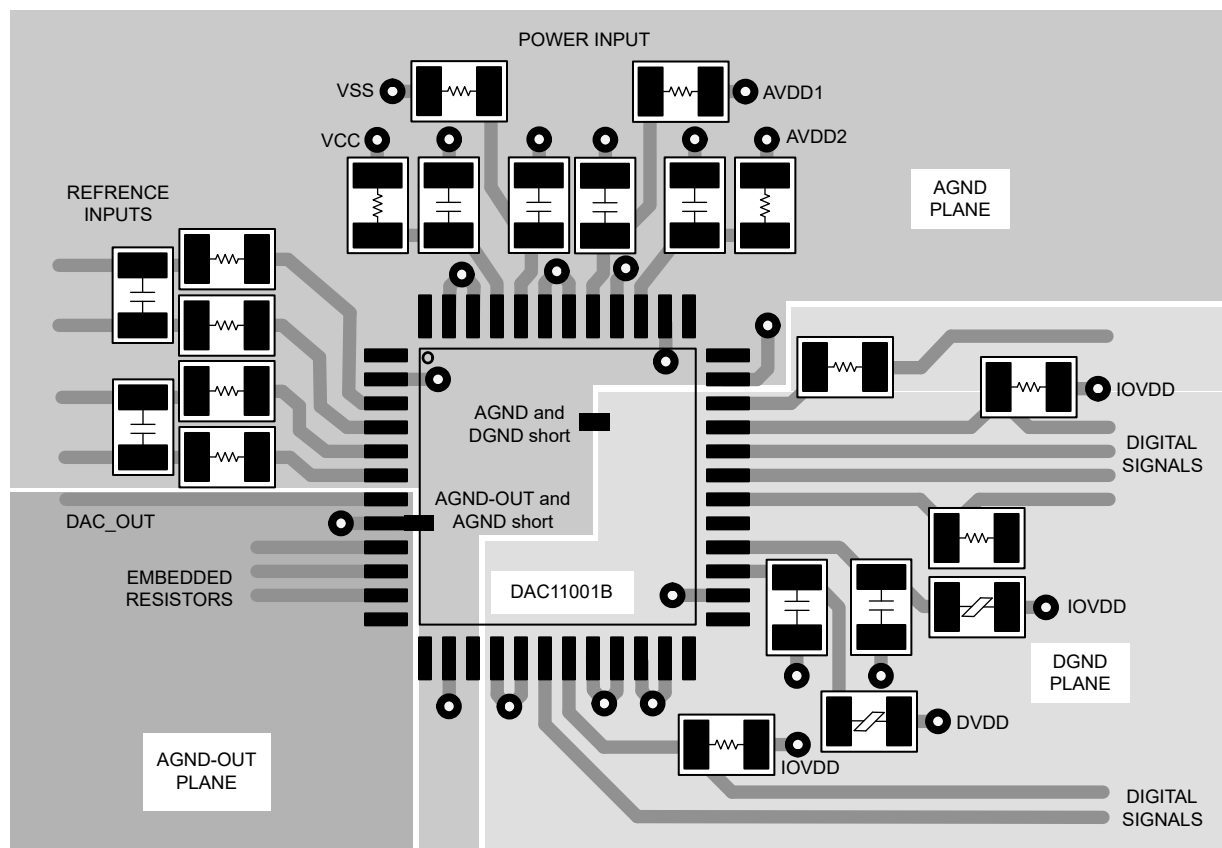
图 10-4. Layout Example
