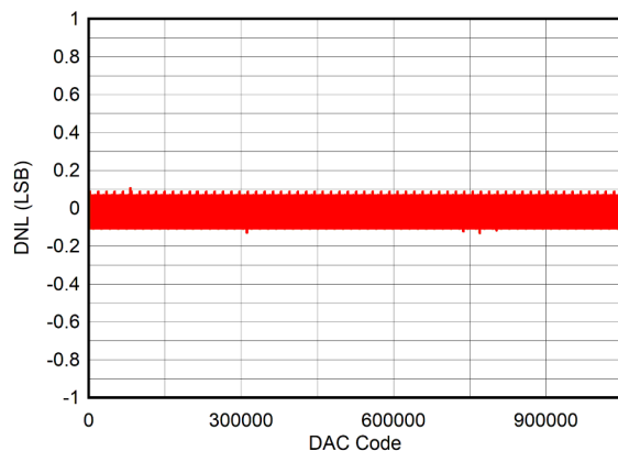
图 8-3. DNL at \pm 10 -V Output
