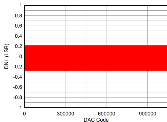
图 8-6. DNL at \pm 5\text{-V} Output
