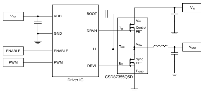
典型电路
