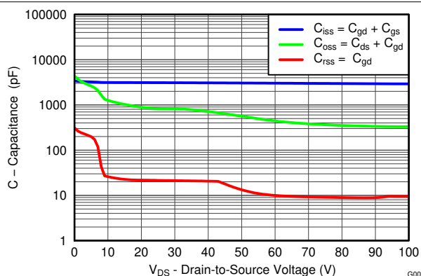
图 4-5. Capacitance
