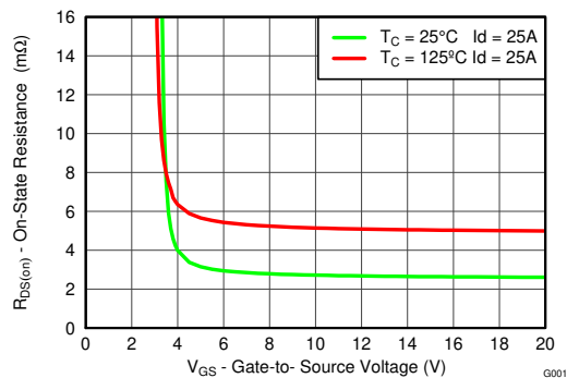
R_{DS(on)} 与 V_{GS} 之间的关系
