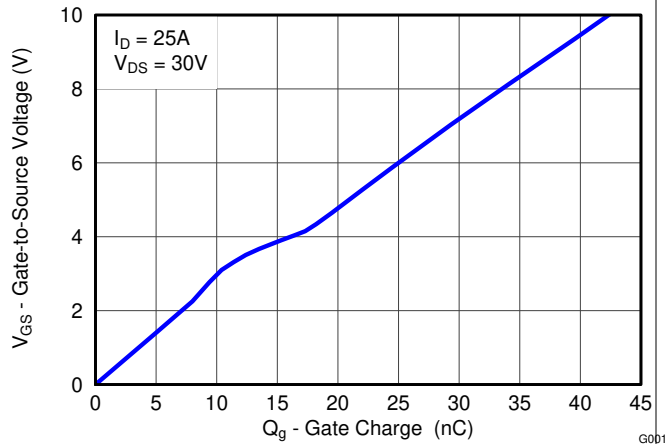
图 4-4. 栅极电荷
