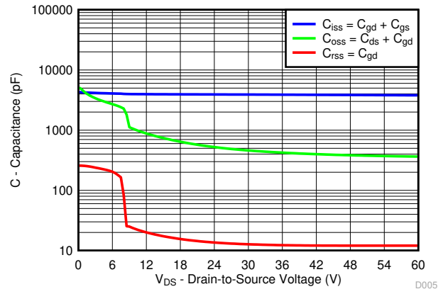
图 4-5. 电容
