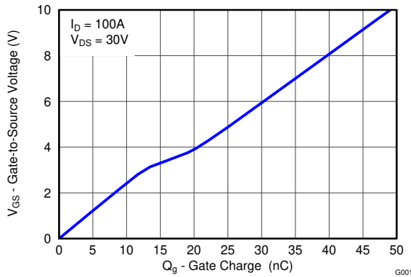
图 3-4. Gate Charge
