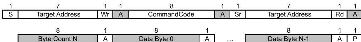
图 7-8. 块读取协议
