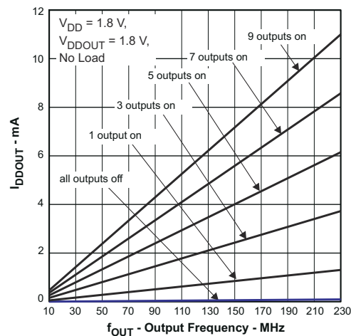
图 5-3. CDCEL949 输出电流与输出频率对比
