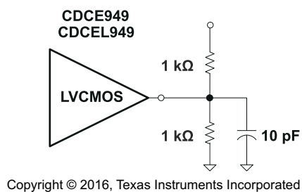
图 6-1. 测试负载
