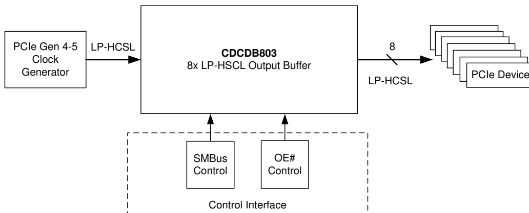
CDCDB803 系统图
