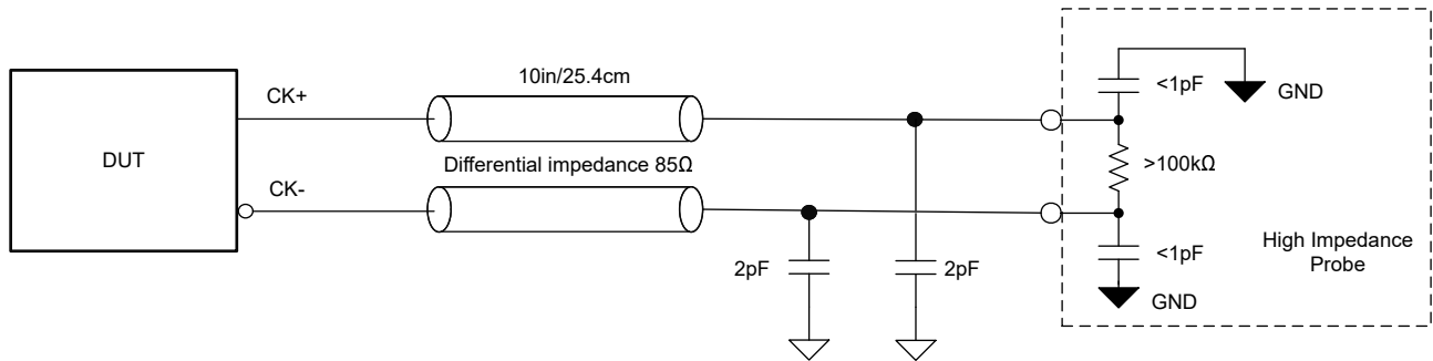
图 6-1. 交流测试负载 (参考 Intel DB2000QL 文档)
