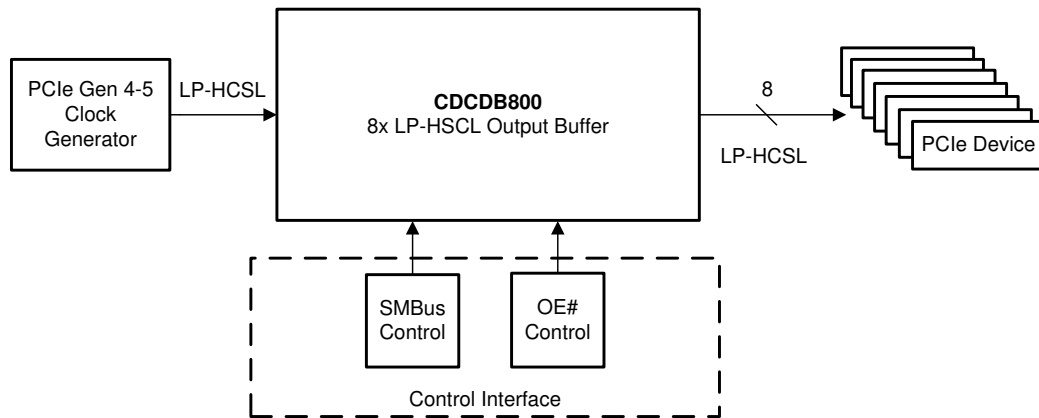
CDCDB800 系统图
