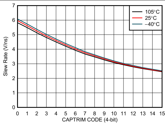
图 9-2. 输出压摆率与 CAPTRIM 代码间的关系
