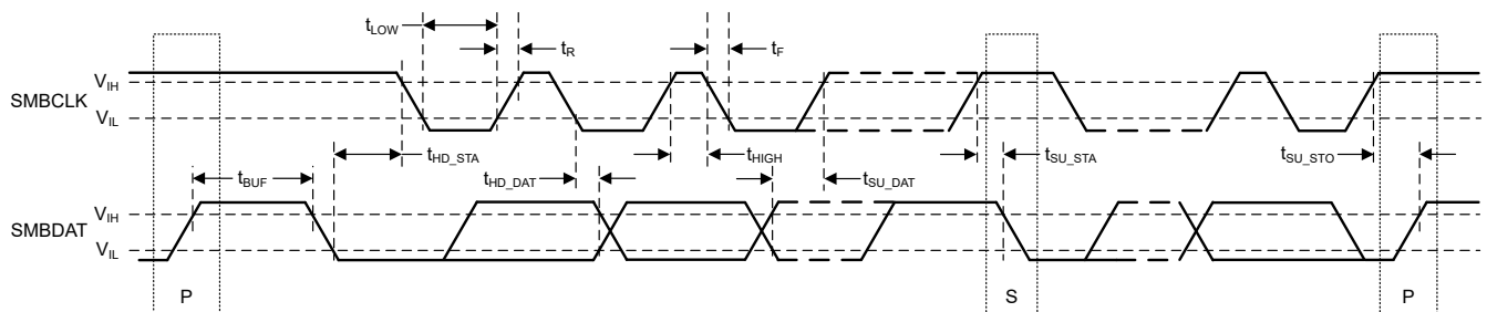
图 7-7. SMBus 时序图
