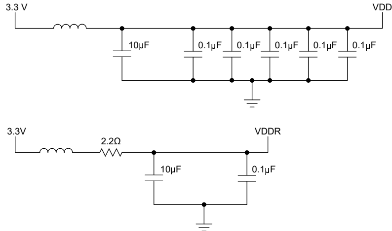
图 9-4. 电源去耦
